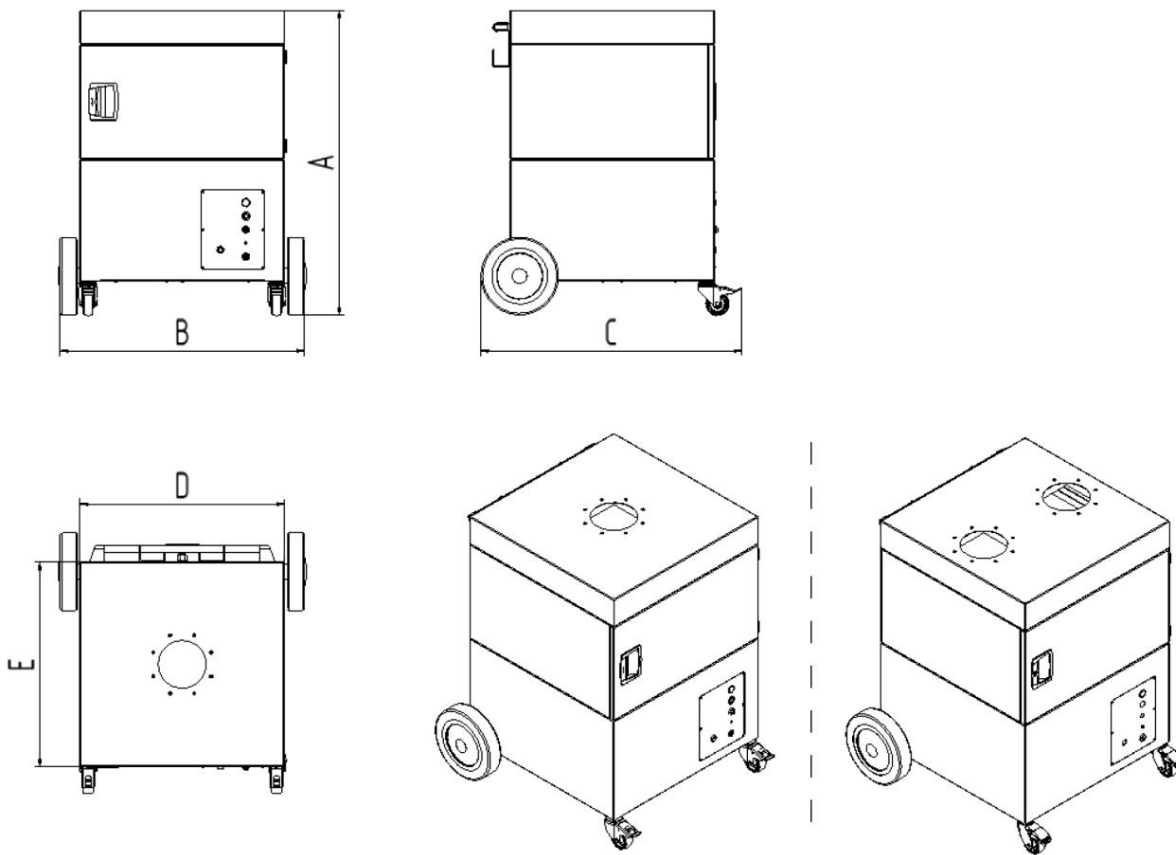
Abb. 9: Maßblatt 60650 + 60650DA
