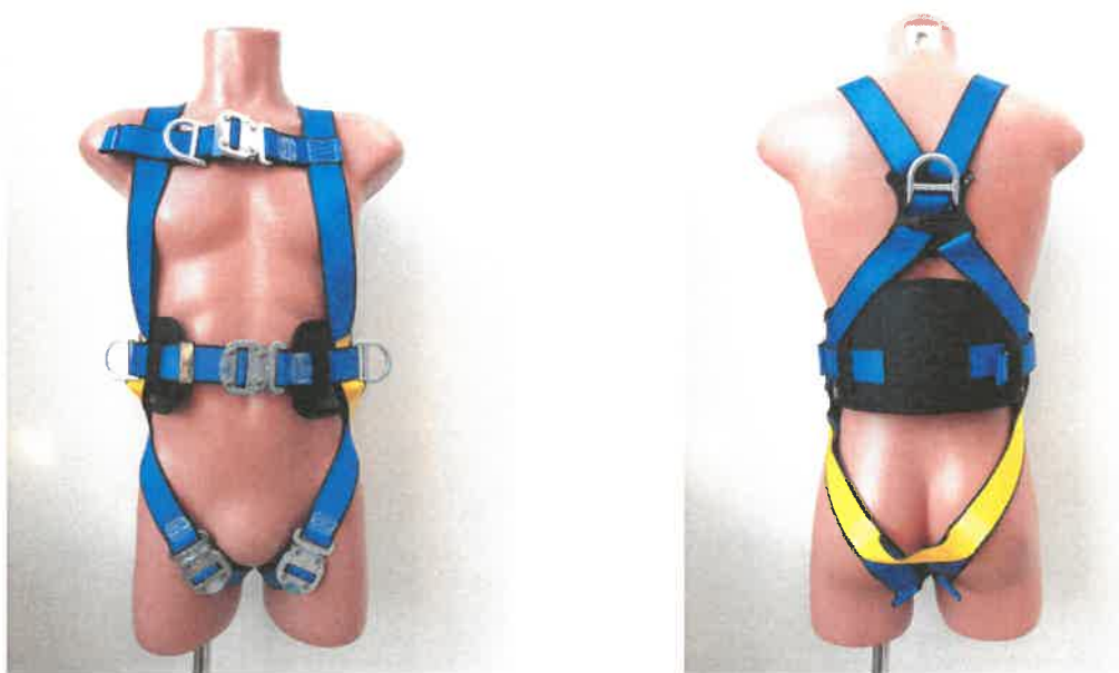
Bezpečnostní postroj / Full body harness, typ / type 1310125
