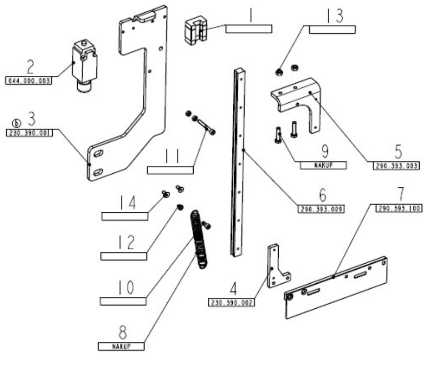
Fig / Abb. 9: Spare part drawing / Ersatzteilzeichnung 8 A: Control panel/ Bedienfeld, B: Working position / Arbeitsposition
