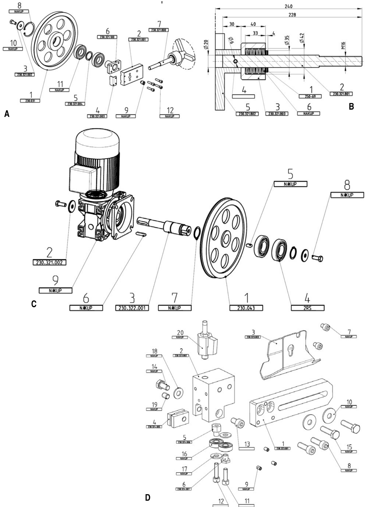
Fig. / Abb. 7: Spare part drawing / Ersatzteilzeichnung 7 - A: Tension pulley / Spannrolle, B: clamping device / Spannvorrichtung, C: Drive roller /Antriebsrolle, D: Fixed guide / Feste Bandführung
