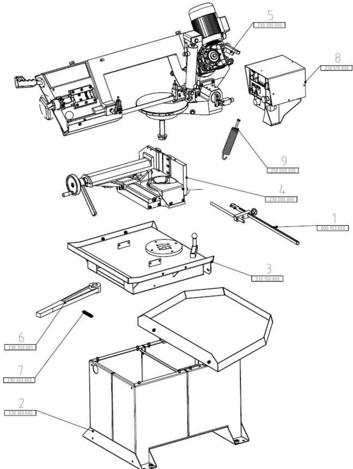
Fig. / Abb. 1: Spare part drawing 1 / Ersatzteilzeichnung 1
