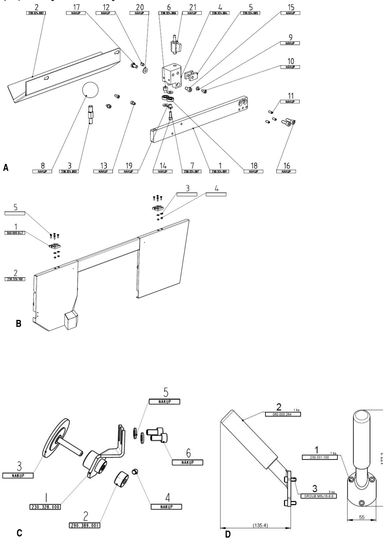
Fig. / Abb. 8: Spare part drawing / Ersatzteilzeichnung 8 A: Movable guide / Bewegliche Bandführung, B: Rollers cover / Rollen-Abdeckung C: Chip brushes / Spänebürste, D: Handle / Griff
