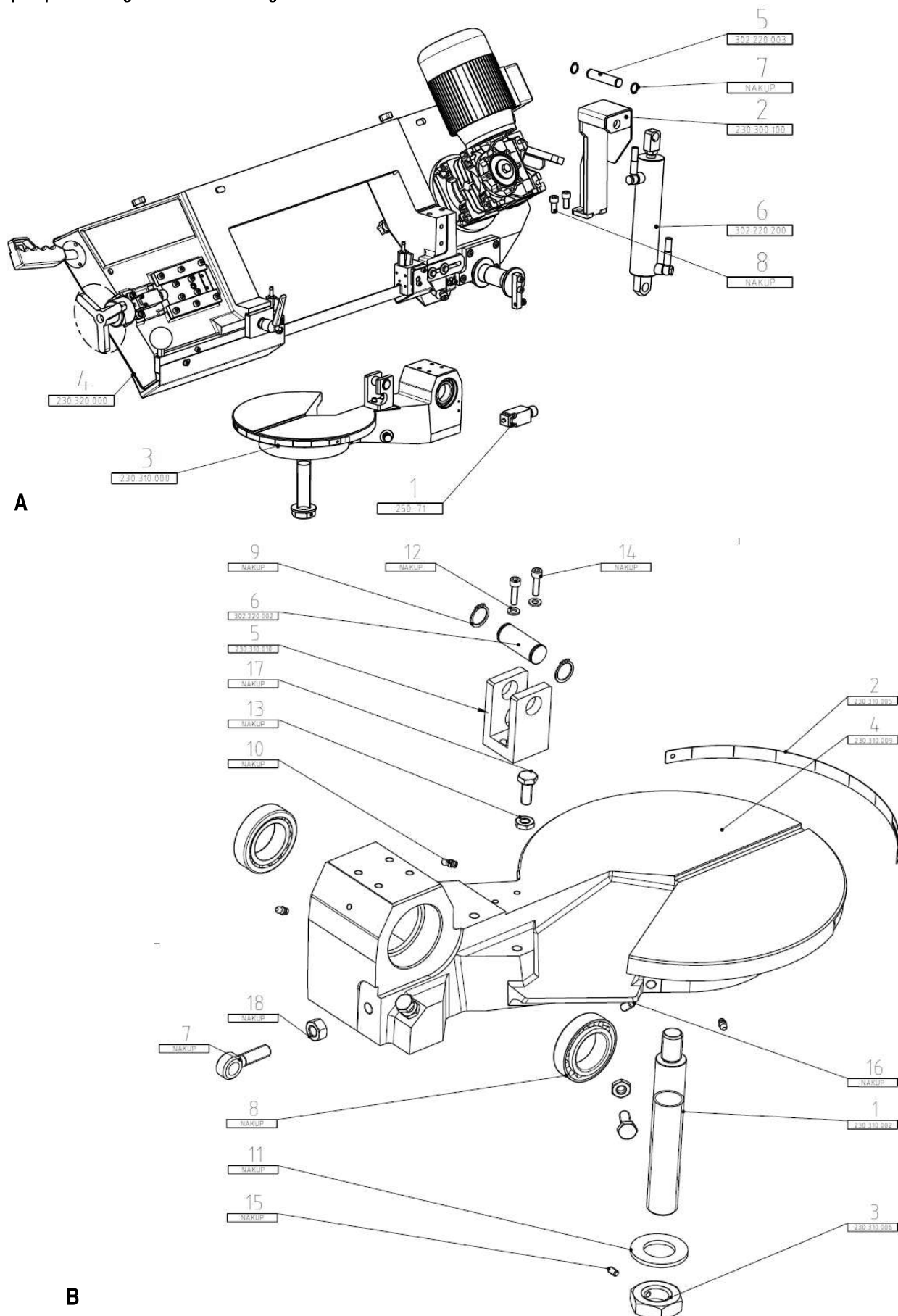
Fig. / Abb. 5: Spare part drawing / Ersatzteilzeichnung 5 - A: Working table with saw arm / Arbeitstisch mit Sägearm ; B: Working table / Arbeitstisch
