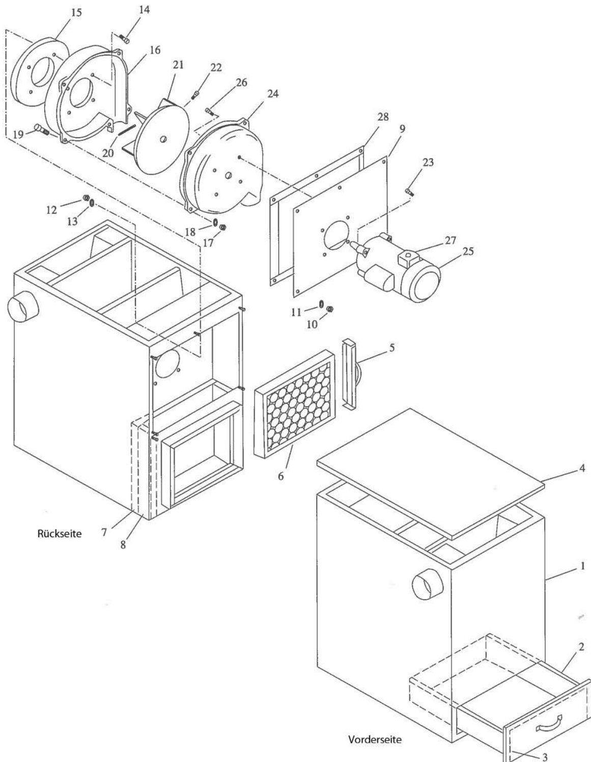
Abb. / Fig. 1: Ersatzteilzeichnung 1/ Spare parts drawing 1
