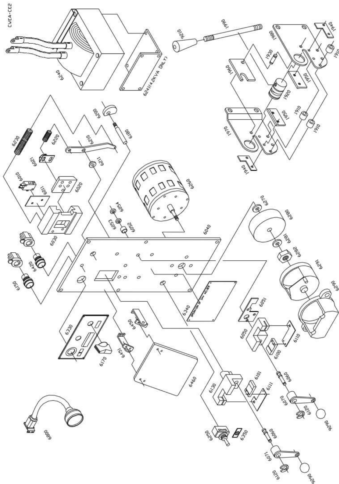
Abb. / Fig. 2: Ersatzteilzeichnung 2 VMBS 1610 / Spare parts drawing 2 VMBS 1610
