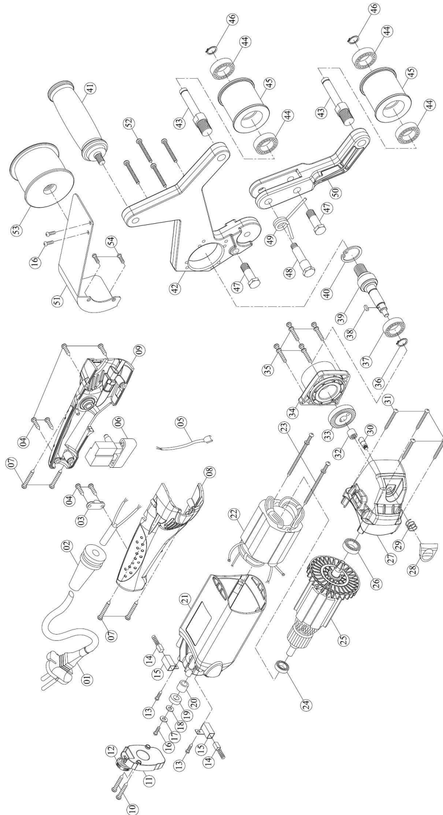
Abb. / Fig. 2: Ersatzteilzeichnung / Spare parts Drawing RSM 760
