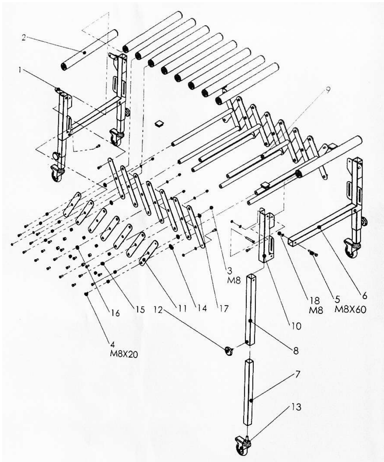
Abb. / Fig. 1: Ersatzteilzeichnung - SRB 130 / Spare parts drawing - SRB 130
