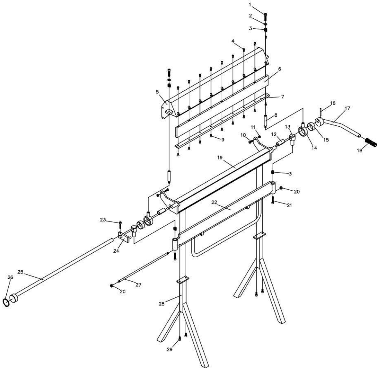
Abb. / Fig. 1: Ersatzteilzeichnung 1 H & N Serie / Spare parts drawing 1 H & N Series
