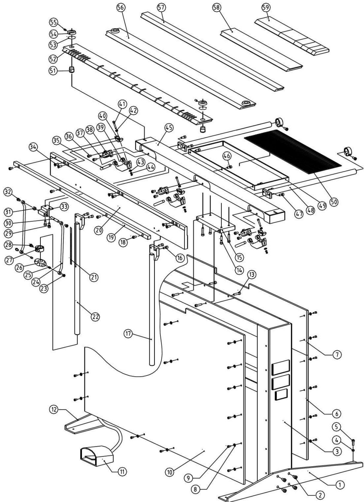
Abb. / Fig. 1: Ersatzteilzeichnung / Spare parts drawing MBM 1250
