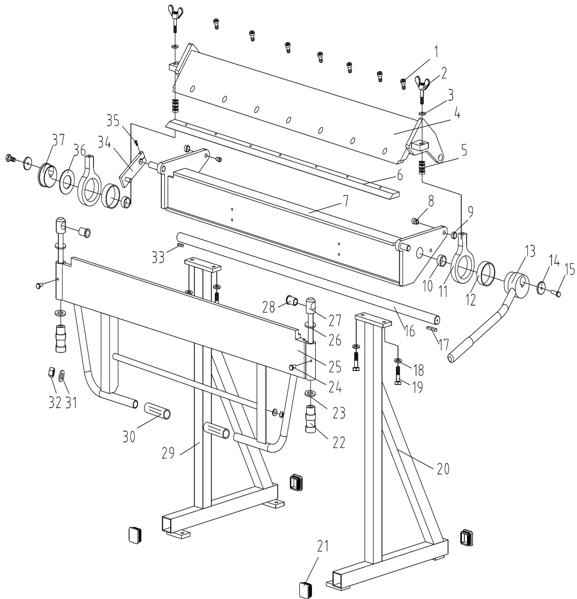
Abb. / Fig. 1: Ersatzteilzeichnung HSBM 1020 - 10 / Spare parts drawing HSBM 1020 - 10
