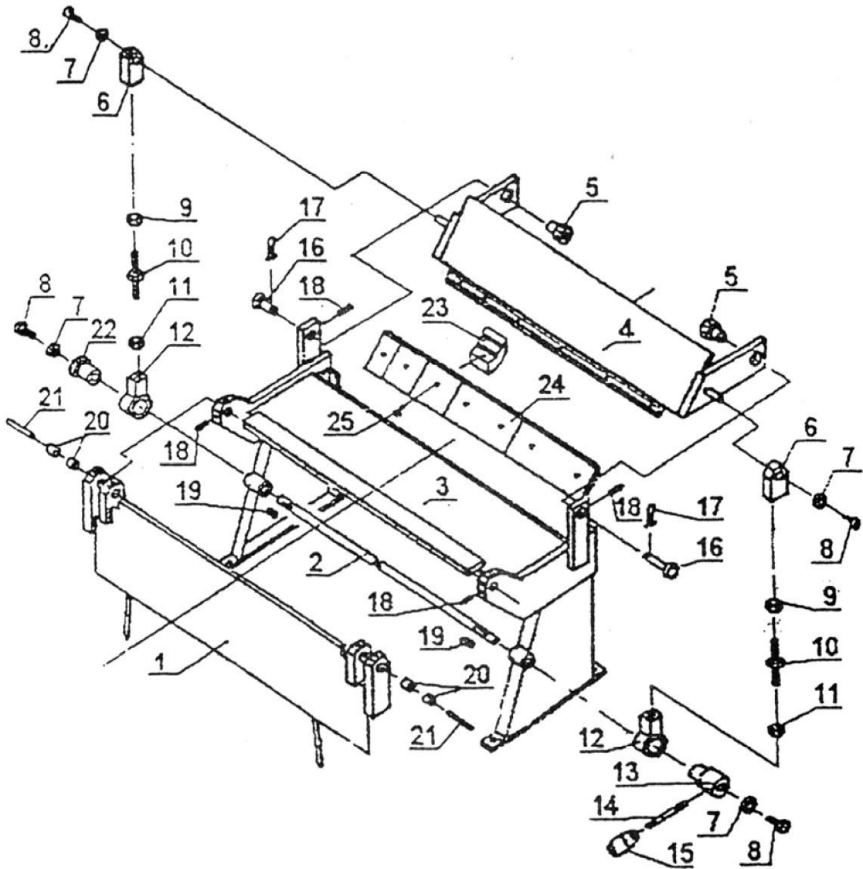
Abb. 8: Ersatzteilzeichnung
