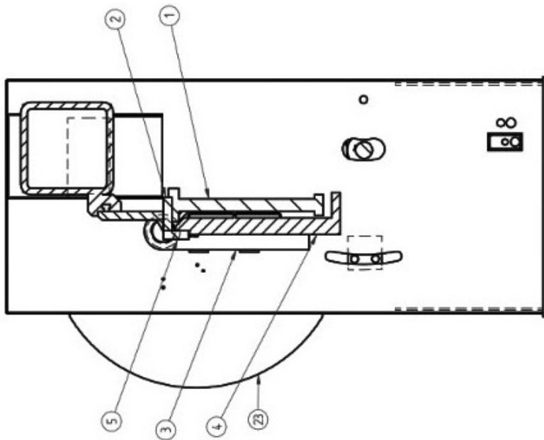
Abb. 2: Ersatzteilzeichnung 2 / Spare parts drawing 2
