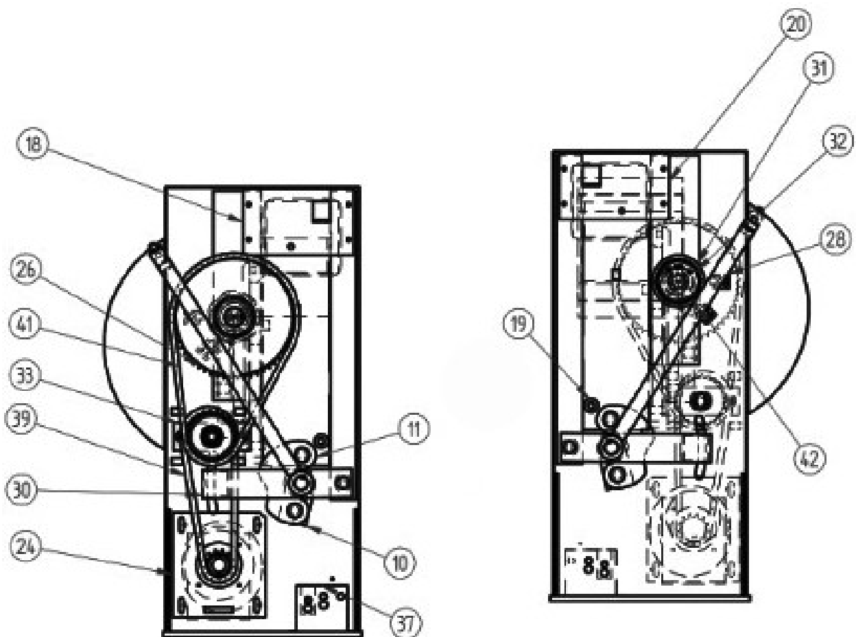
Abb. 3: Ersatzteilzeichnung 3 / Spare parts drawing 3
