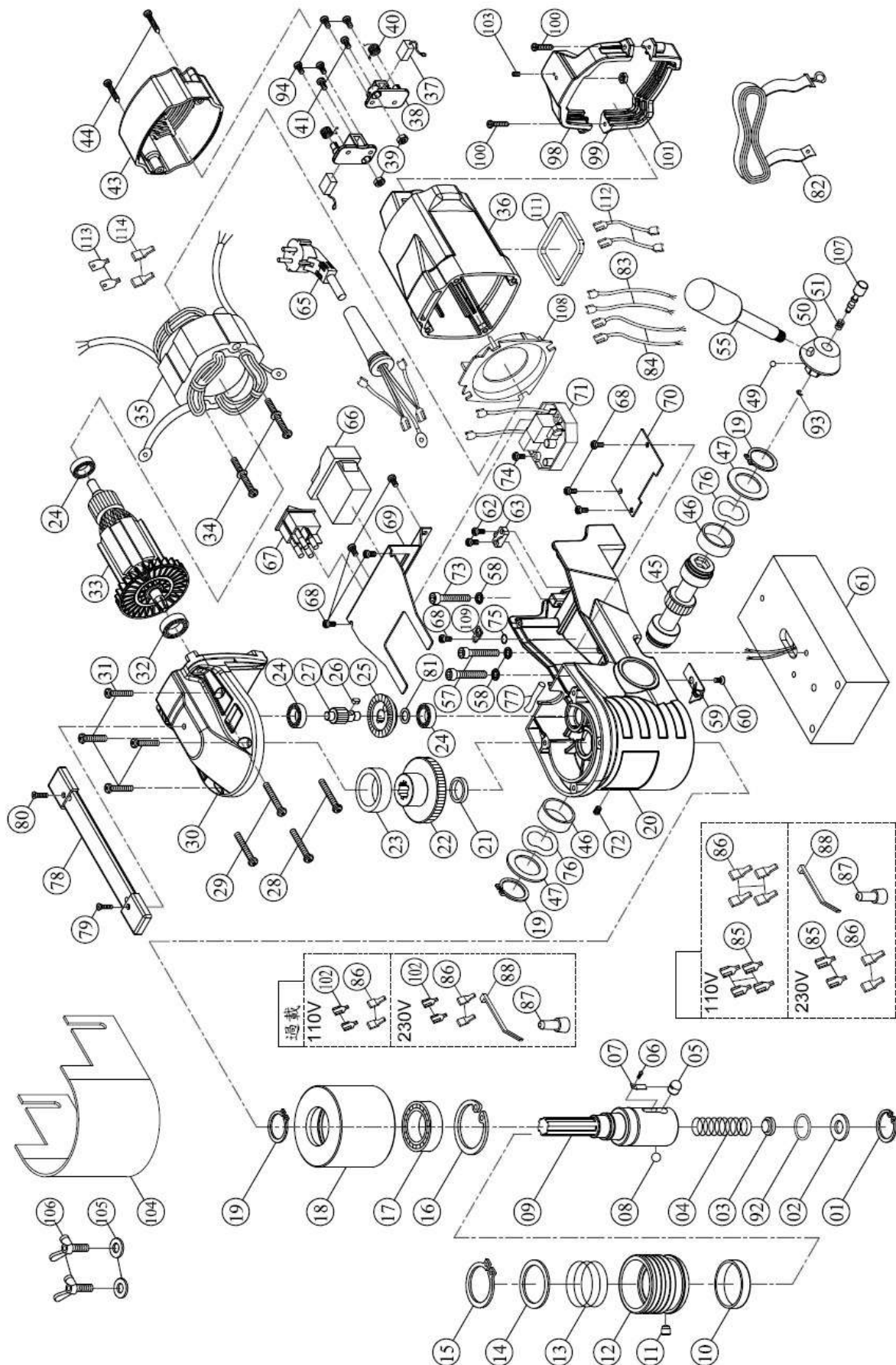
Abb. / Fig. 1: Ersatzteilzeichnung MB 351 F / Spare parts drawing MB 351 F
