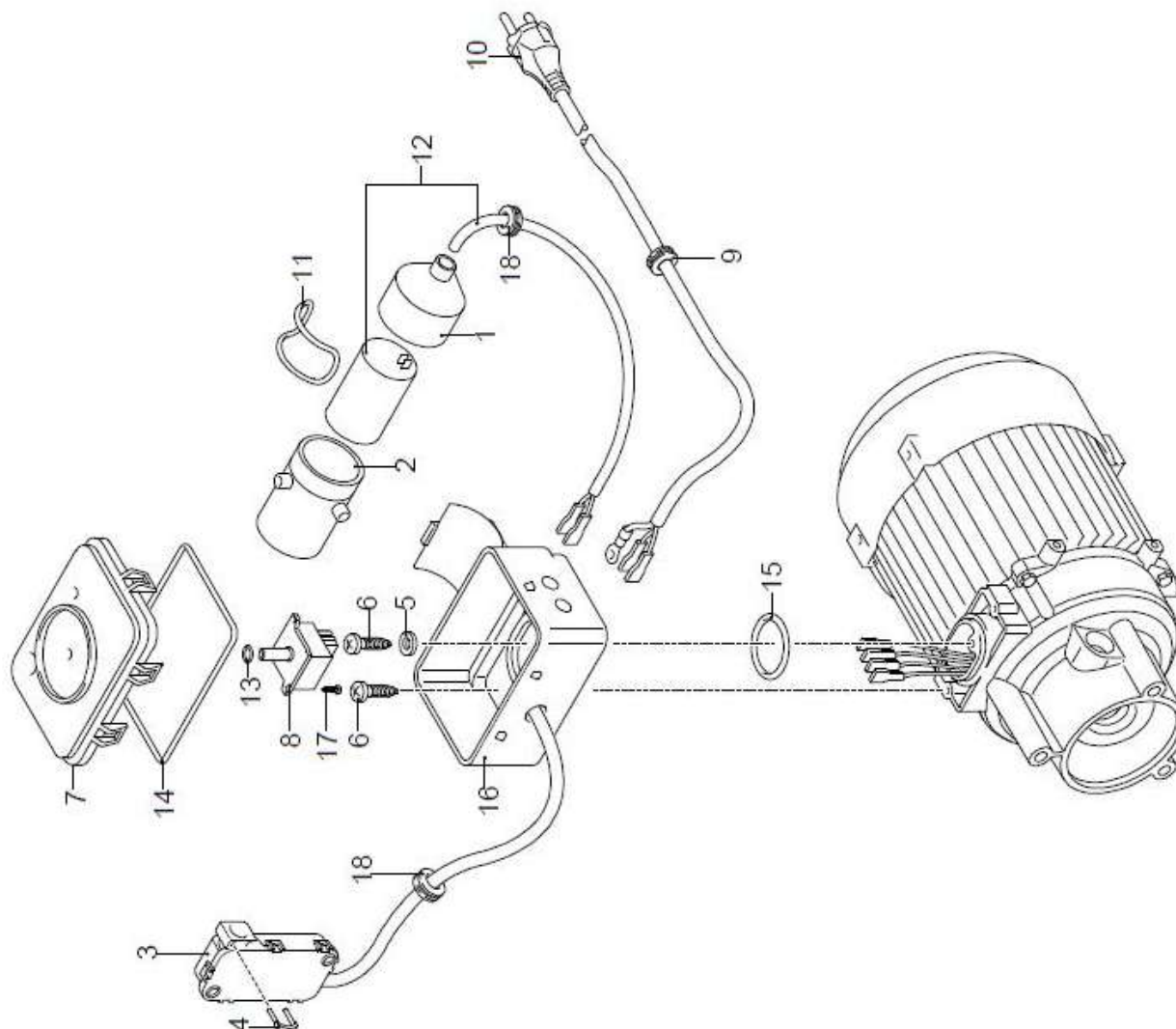
Abb./Img.4: Ersatzteilzeichnung 4 - Spare parts drawing 4
