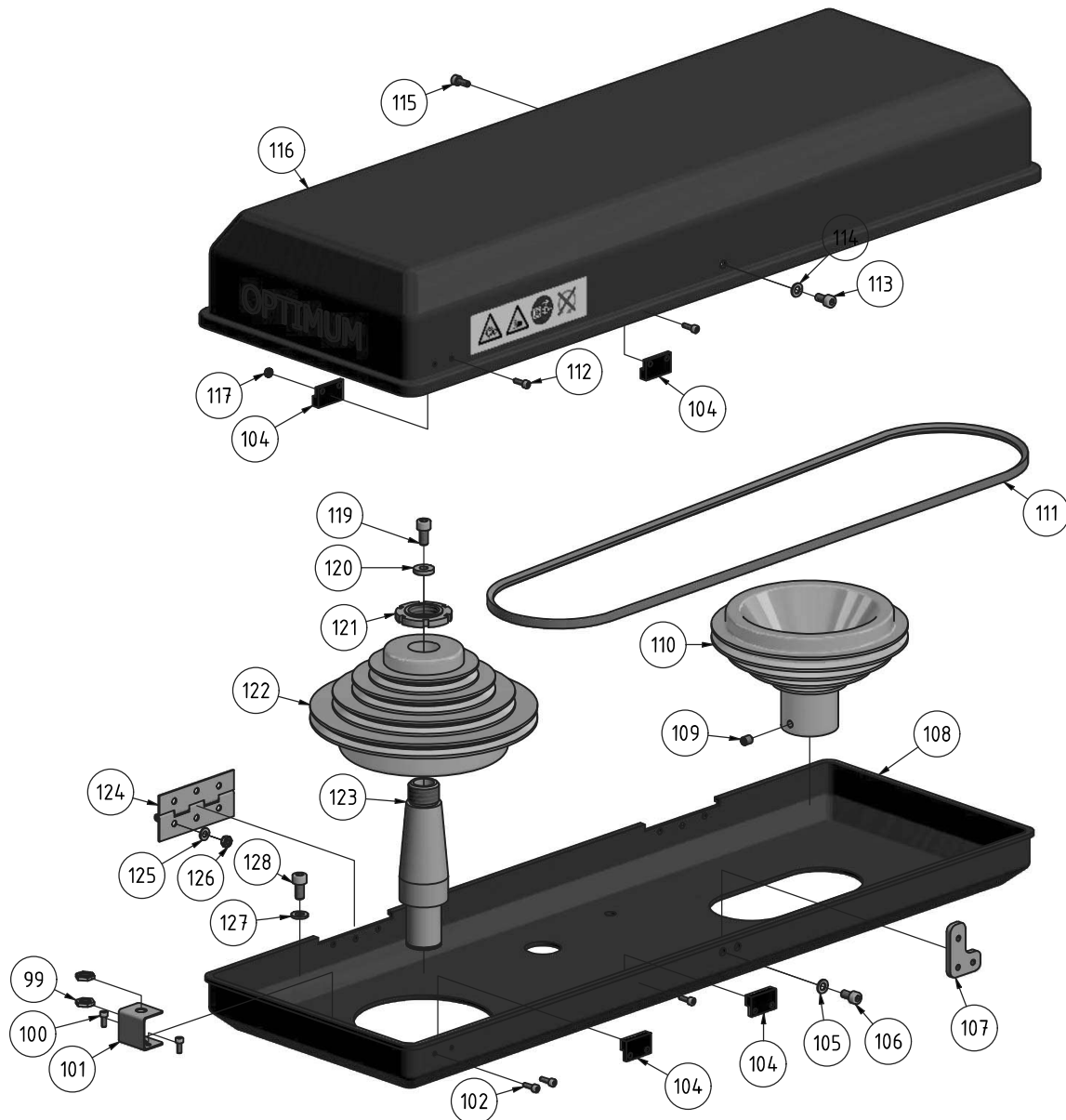
Img.1-6: Keilriemenscheiben B24HV - Pulleys B24HV
