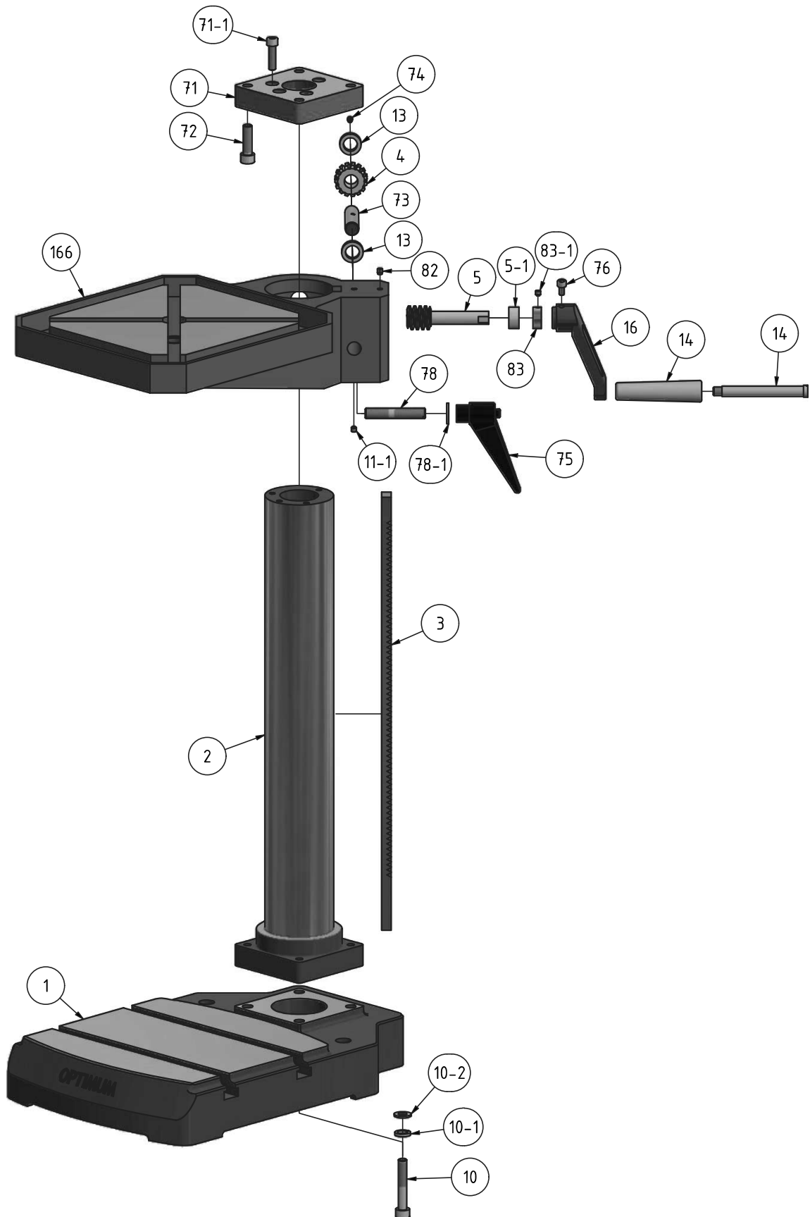
Img.1-2: Säule und Bohrtisch B24H - Column and drilling table B24H
