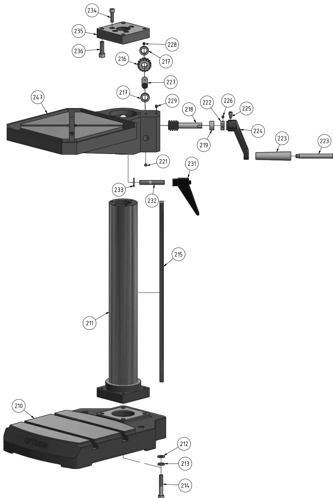
Img.1-5: Säule und Bohrtisch B24HV - Column and drilling table B24HV
