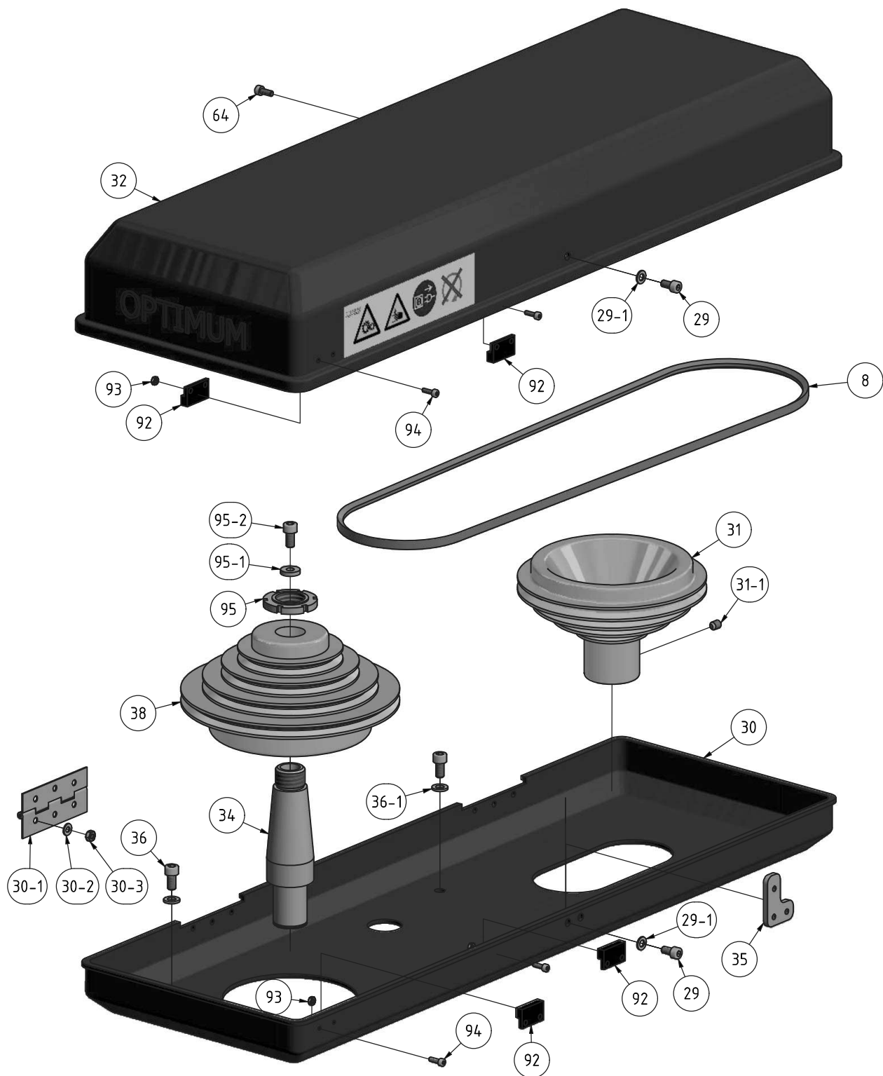
Img.1-3: Keilriemenscheiben B24H - Pulleys B24H
