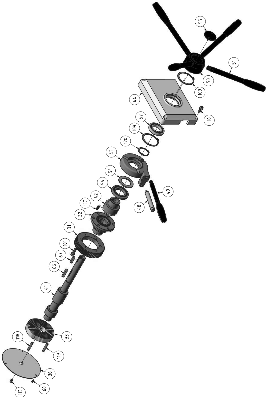
Abb.9-3: Getriebe Teil B - Gear part B
