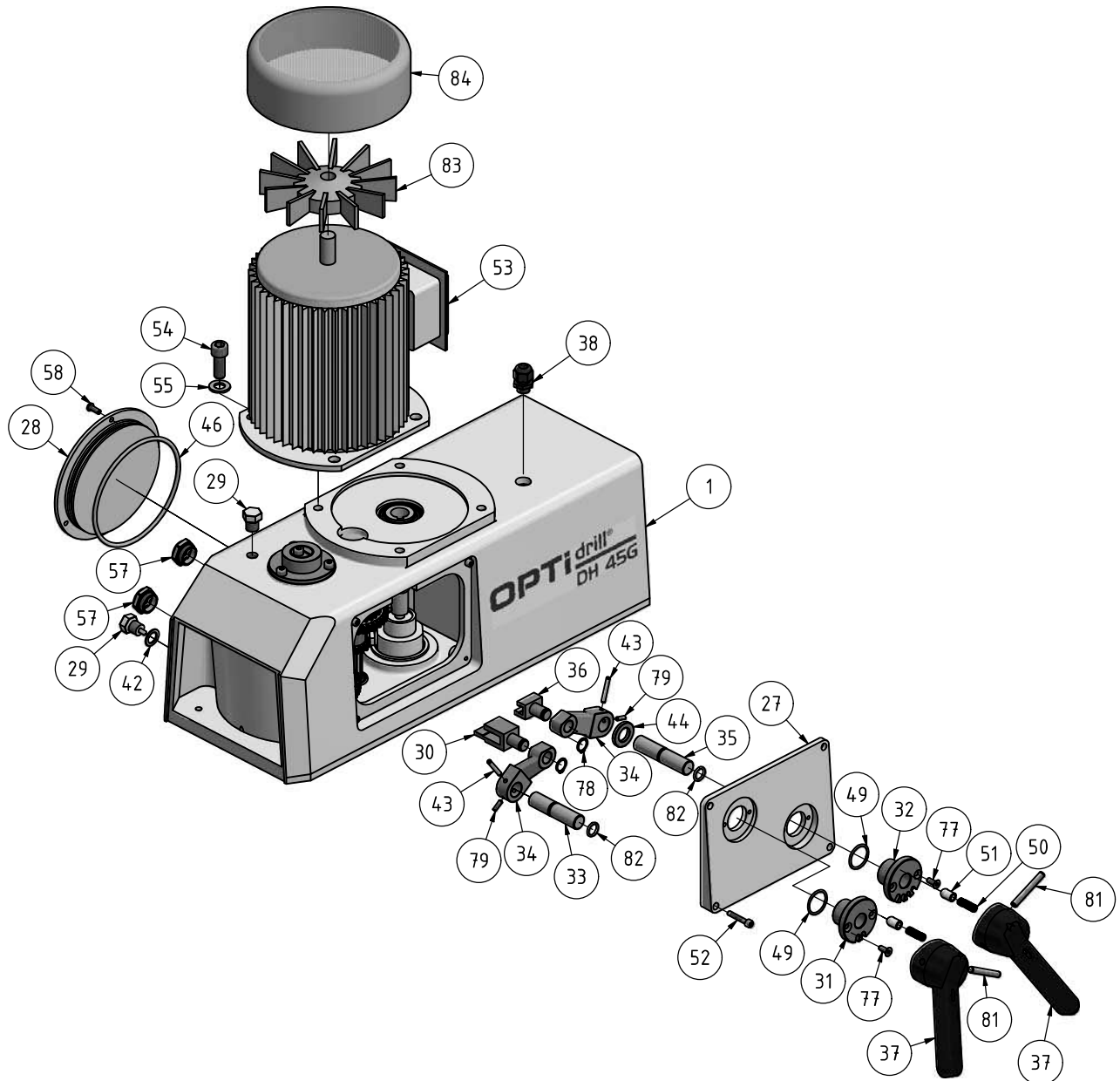
Abb.9-1: Getriebe Teil A - Gear part A
