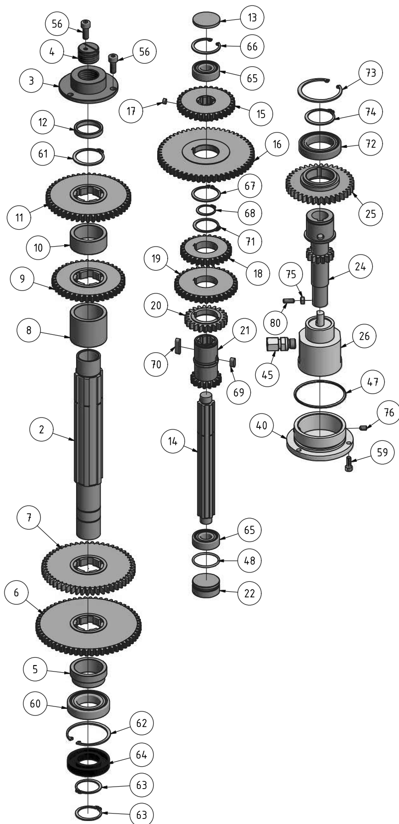
Abb.9-2: Getriebe Teil A - Gear part A
