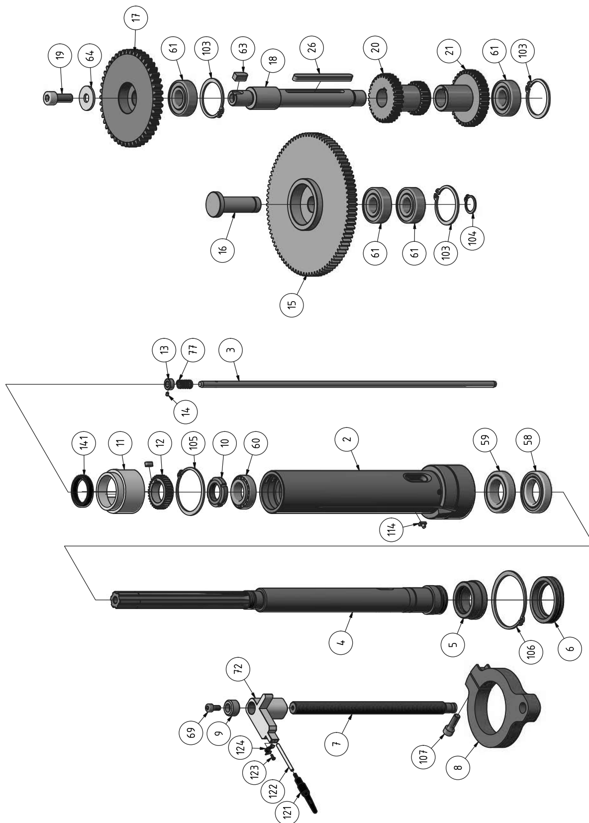
Abb.9-4: Getriebe Teil B - Gear part B
