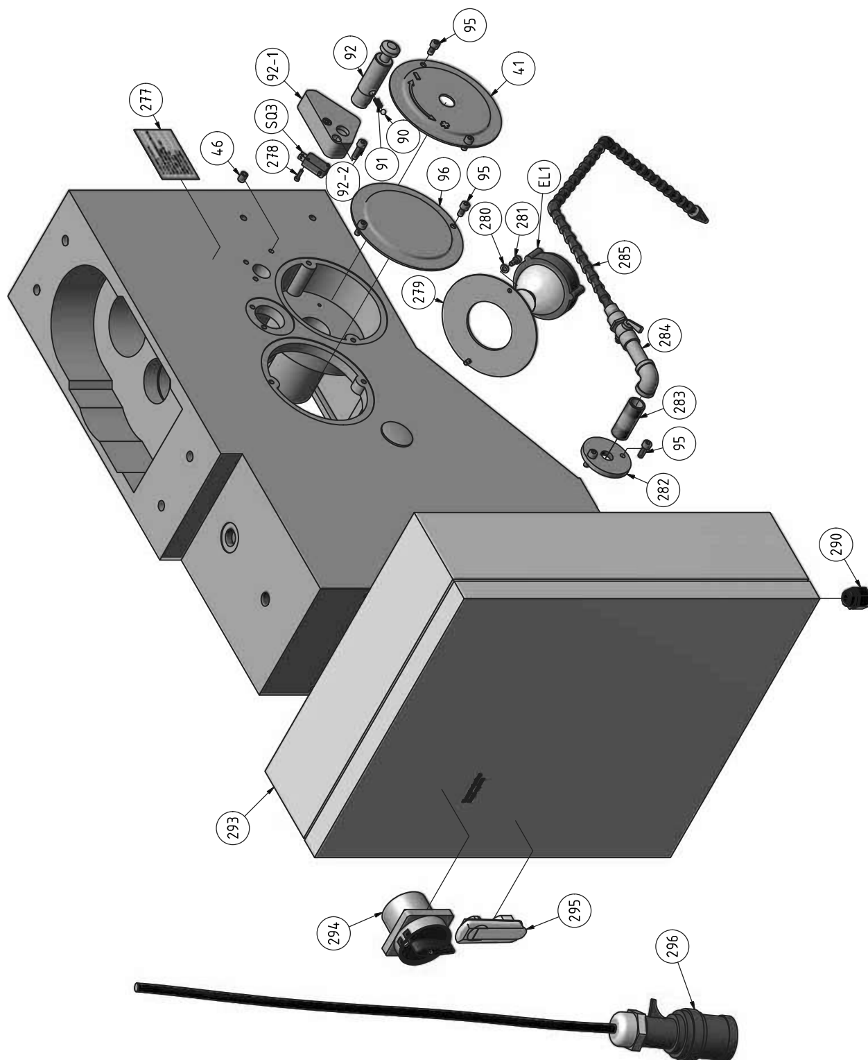
Img.1-10: Vorschubgetriebe 4 von 4 - Feed gear box 4 of 4
