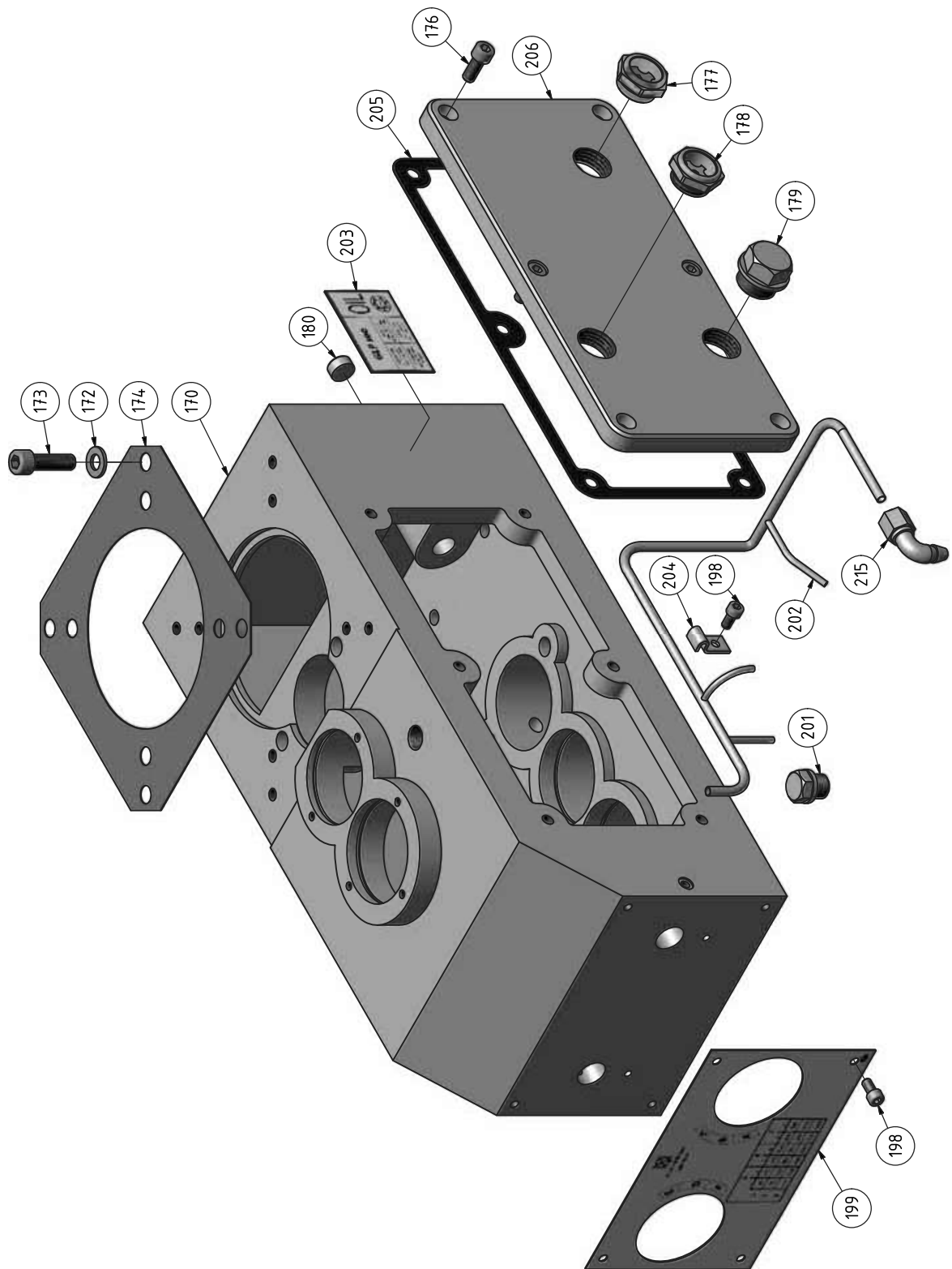
Img.1-5: Getriebe Bohrspindel 4 von 4 - Gear box main spindle 4 von 4
