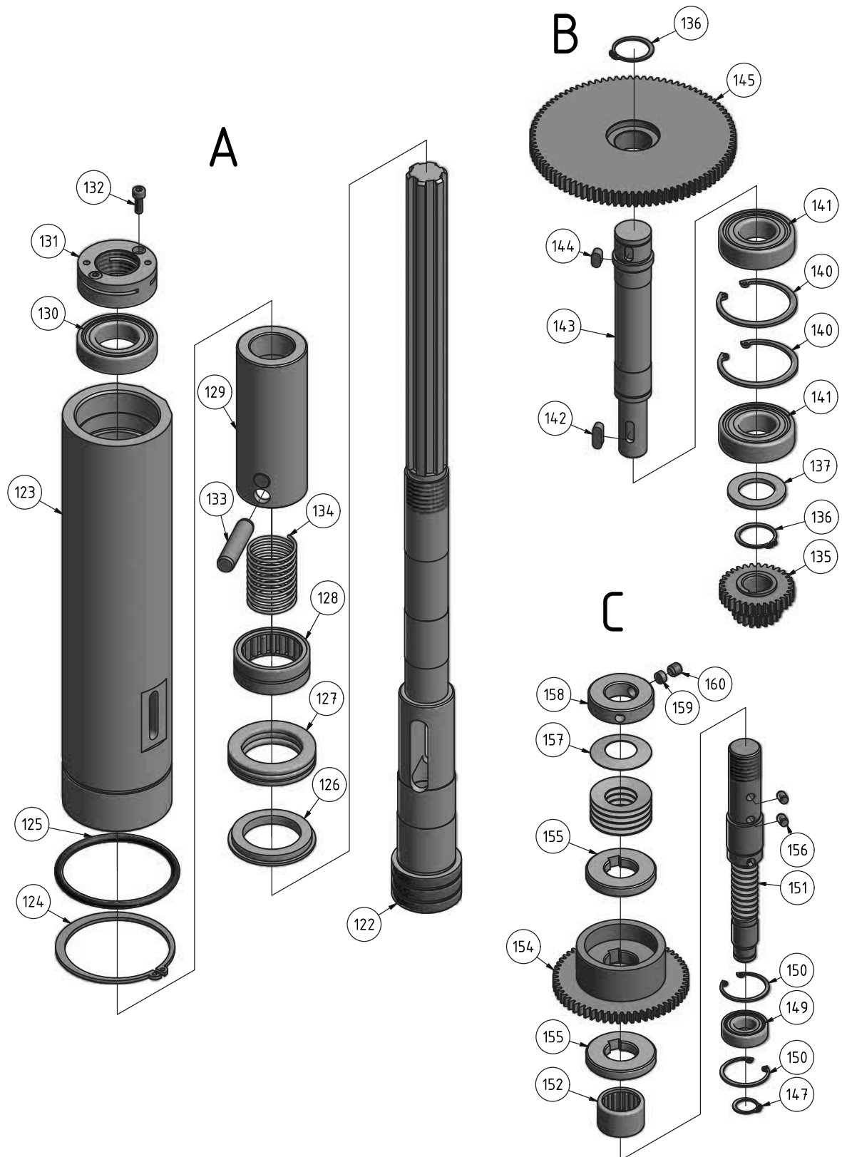
Img.1-7: Vorschubgetriebe 1 von 4 - Feed gear box 1 of 4
