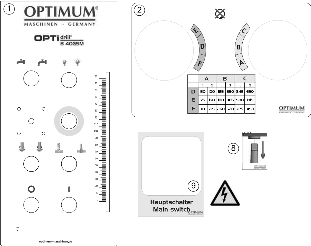
Img.1-13: Maschinenschilder - Machine labels
