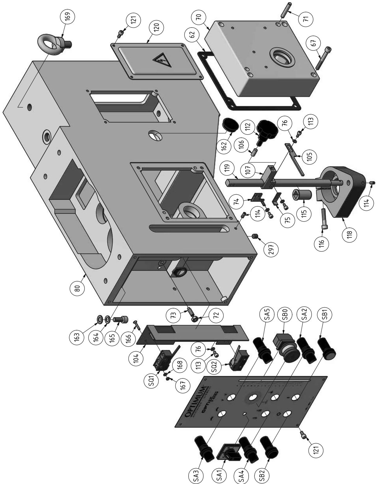
Img.1-9: Vorschubgetriebe 3 von 4 - Feed gear box 3 of 4
