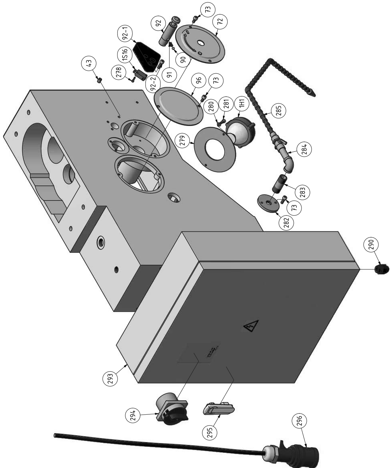
Abb.1-11: Vorschubgetriebe 4 von 4 - Feed gear box 4 of 4
