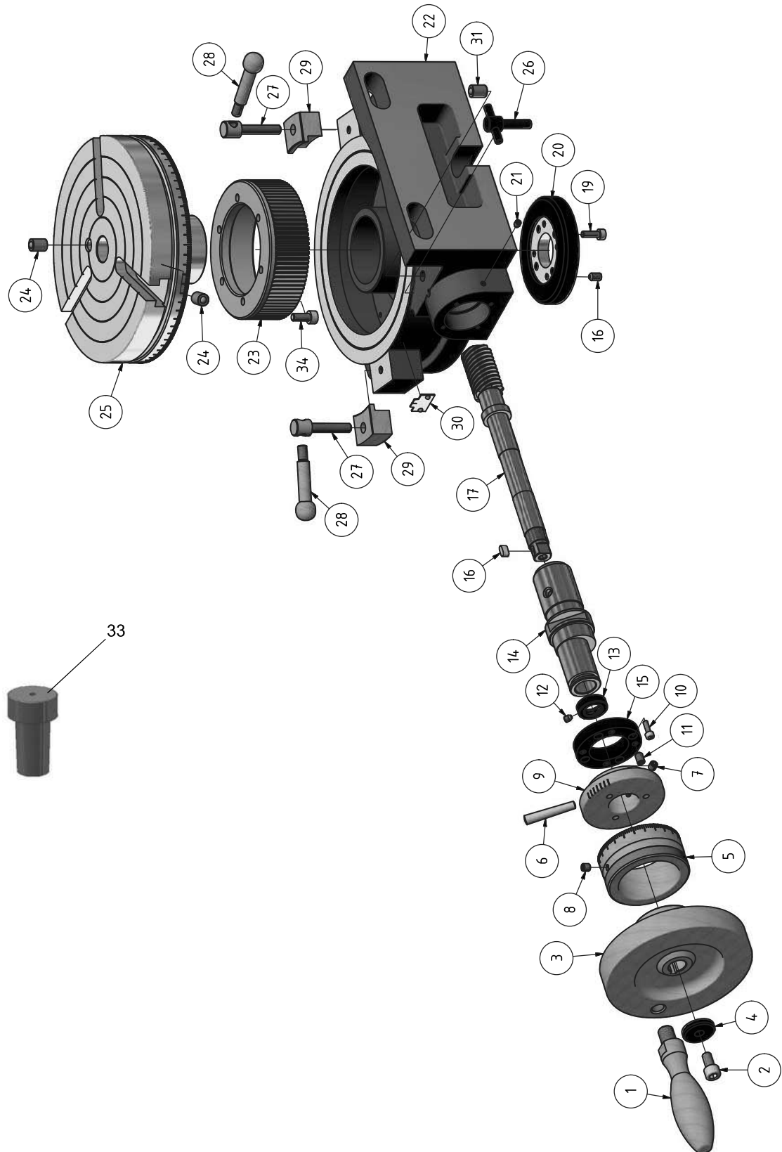
Abb.12-1: Rundteiltisch - RT 150
