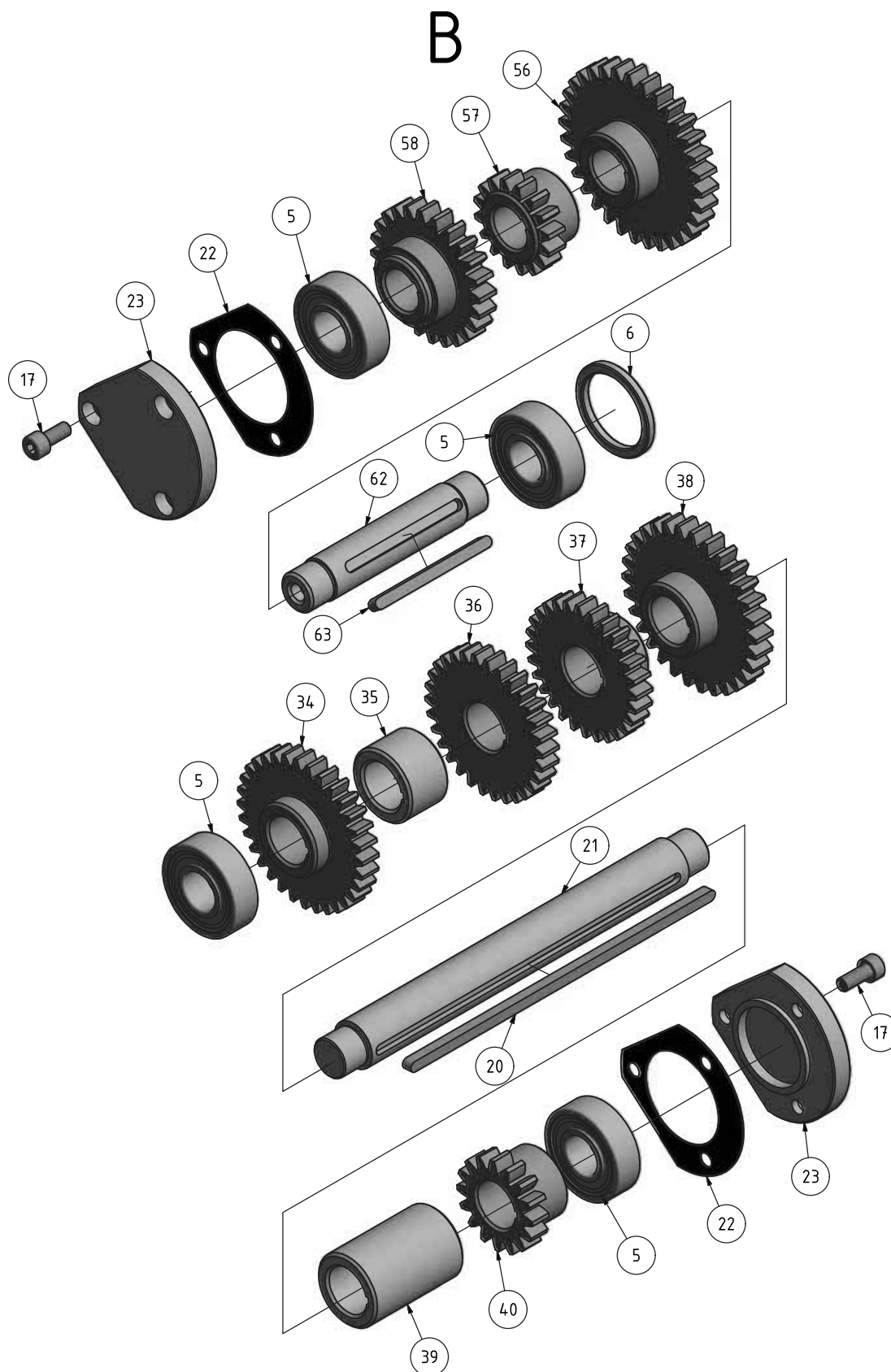
Abb. 1-11: Vorschubgetriebe 4-6 - Feed gear 4-6
