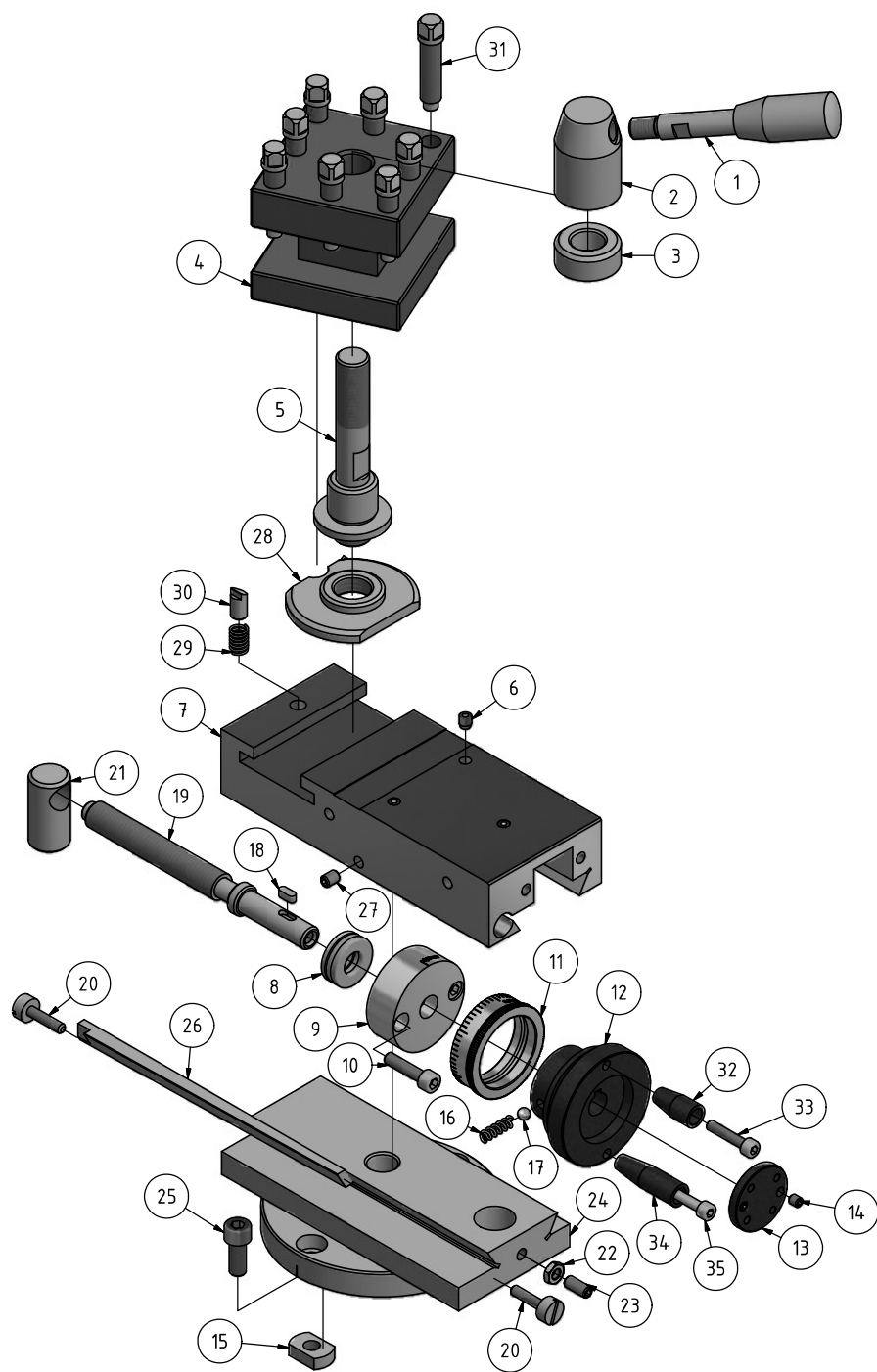
Abb. 1-18: Oberschlitten - Top slide
