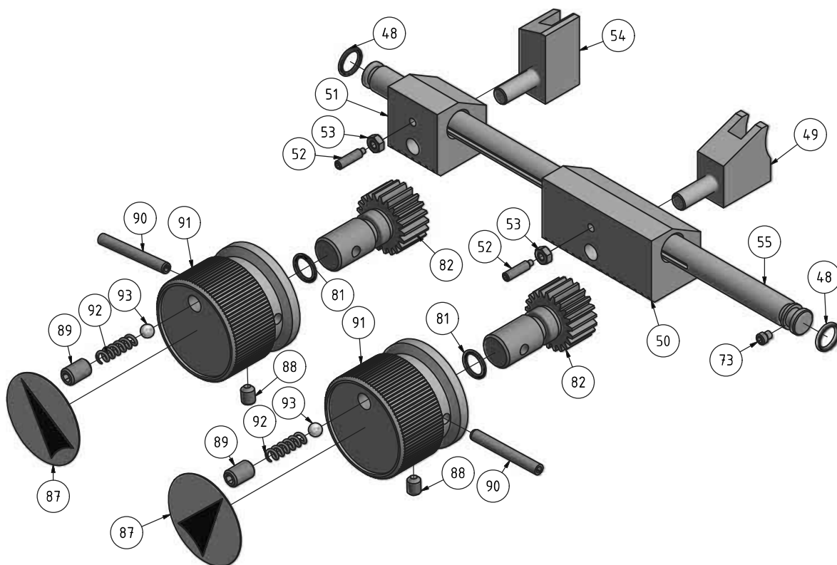
Abb. 1-13: Vorschubgetriebe 6-6 - Feed gear 6-6
