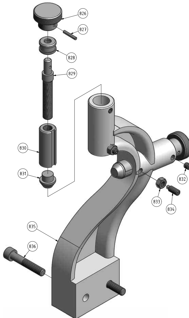
Abb.1-25: Mitlaufende Lünette - Follow rest
