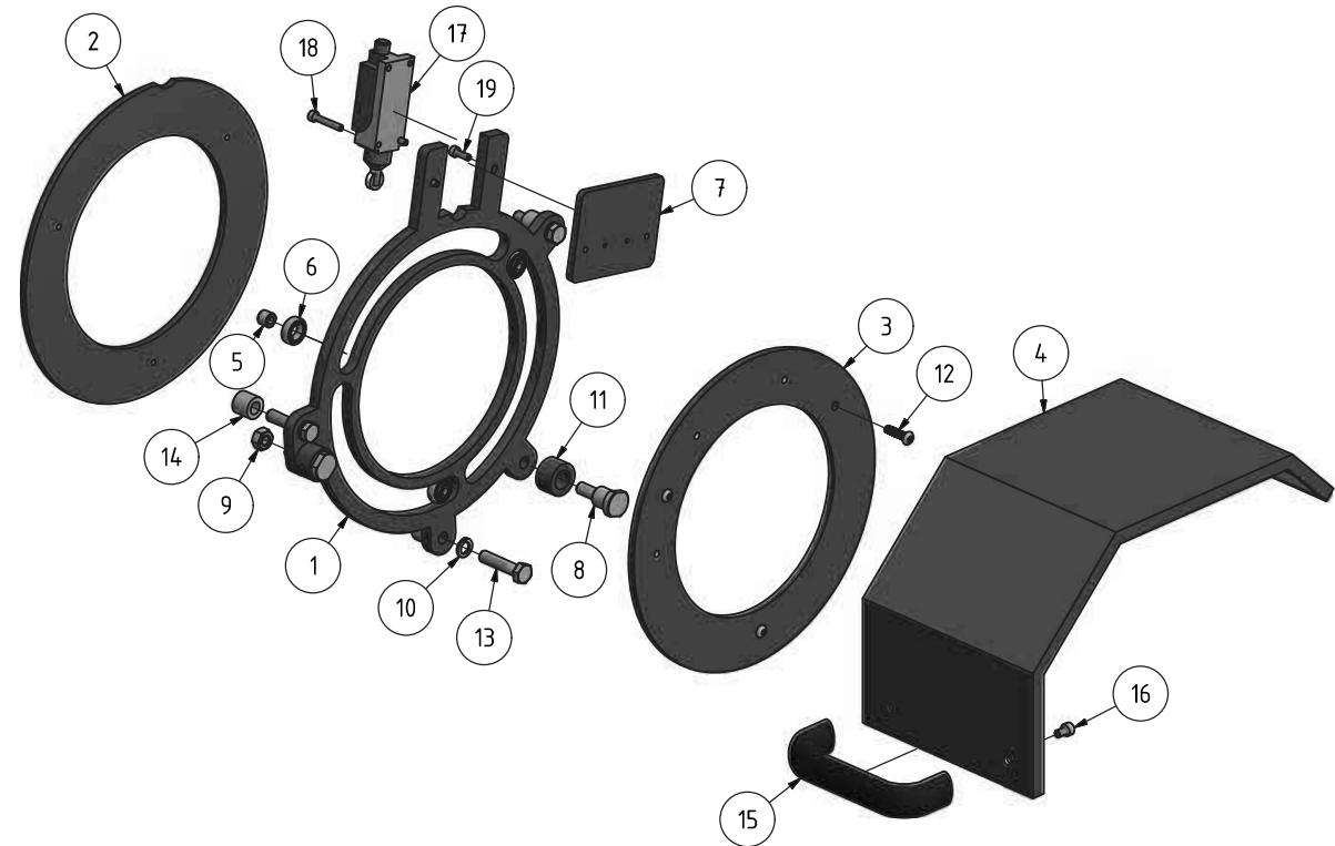
Abb.1-26: Drehfutterschutz - Chuch protection
