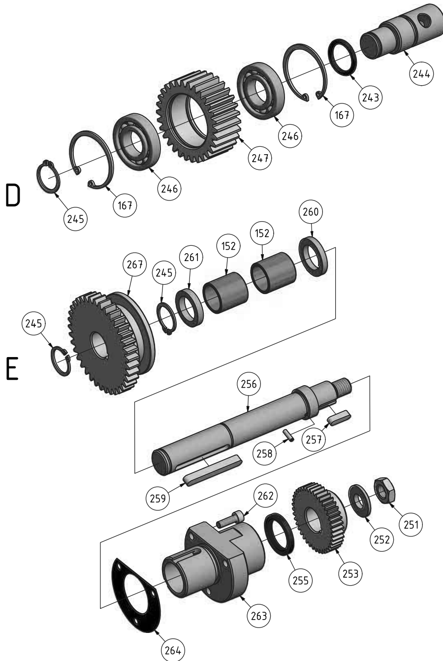
Abb.1-5: Getriebe Spindelstock 5-6 - Headstock gear 5-6
