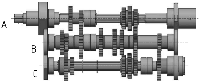
Abb. 1-9: Vorschubgetriebe 2-6 - Feed gear 2-6
