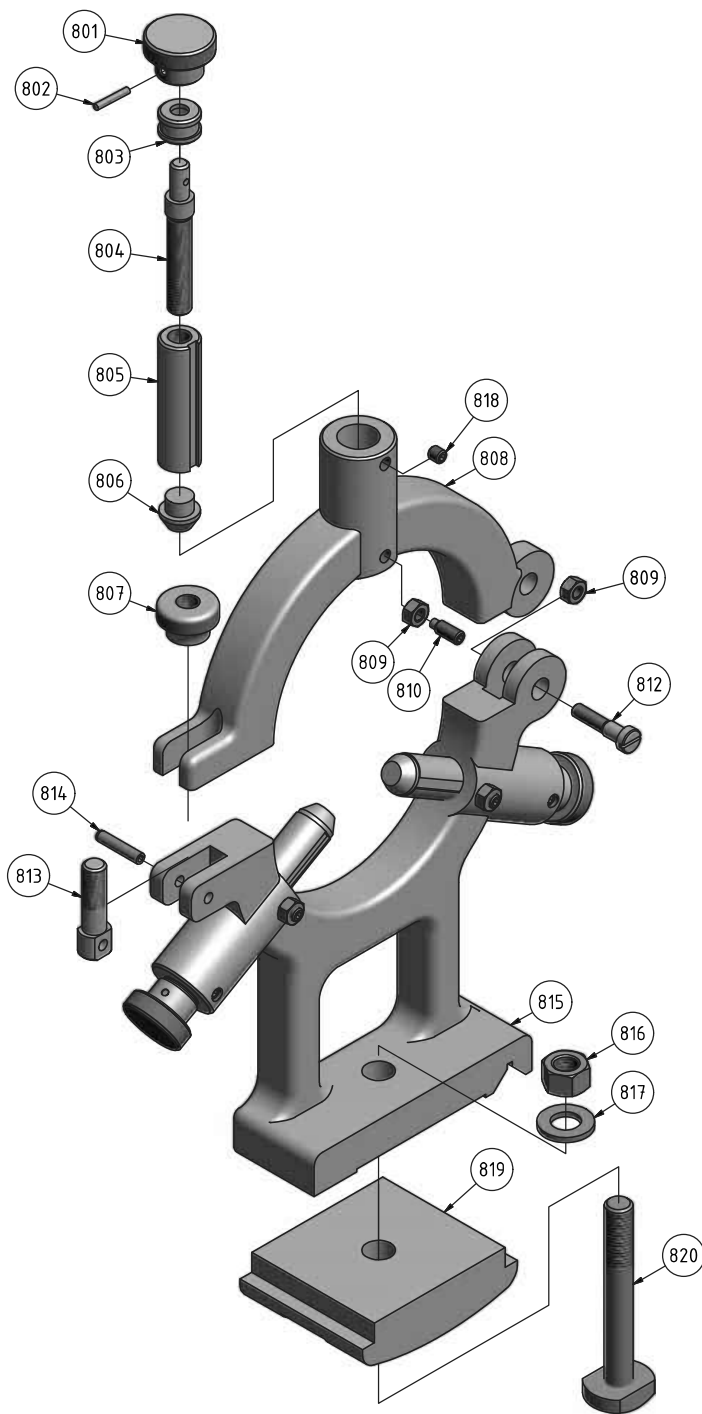
Img.1-23: Feststehende Lünette - Steady rest
