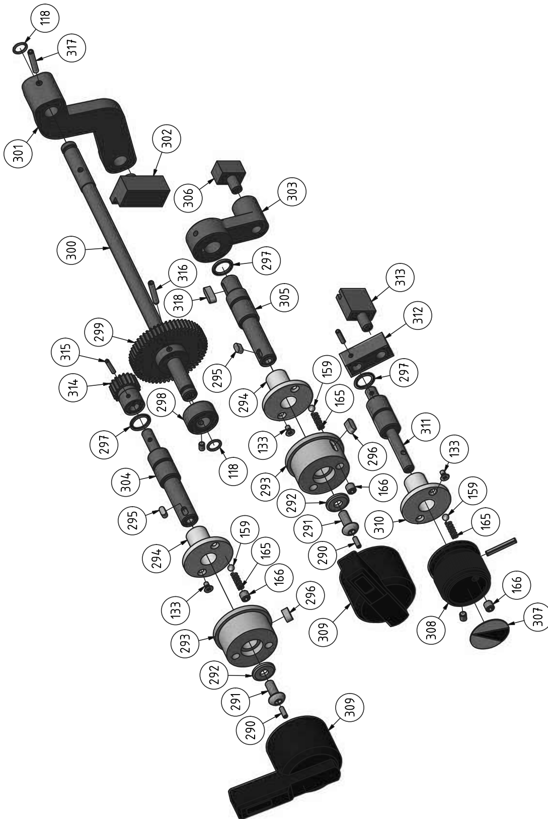
Img. 1-9: Getriebe Spindelstock 6-6 - Headstock gear 6-6
