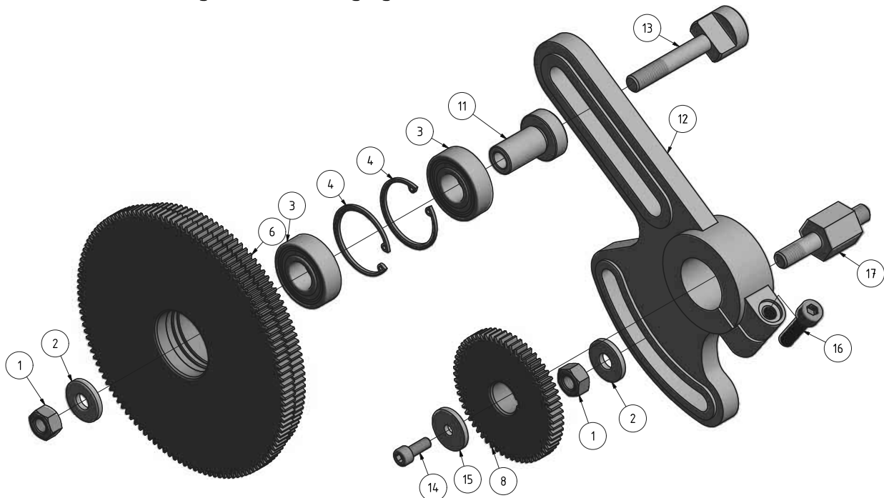
Img.1-16: Wechselradgetriebe- Change gear
