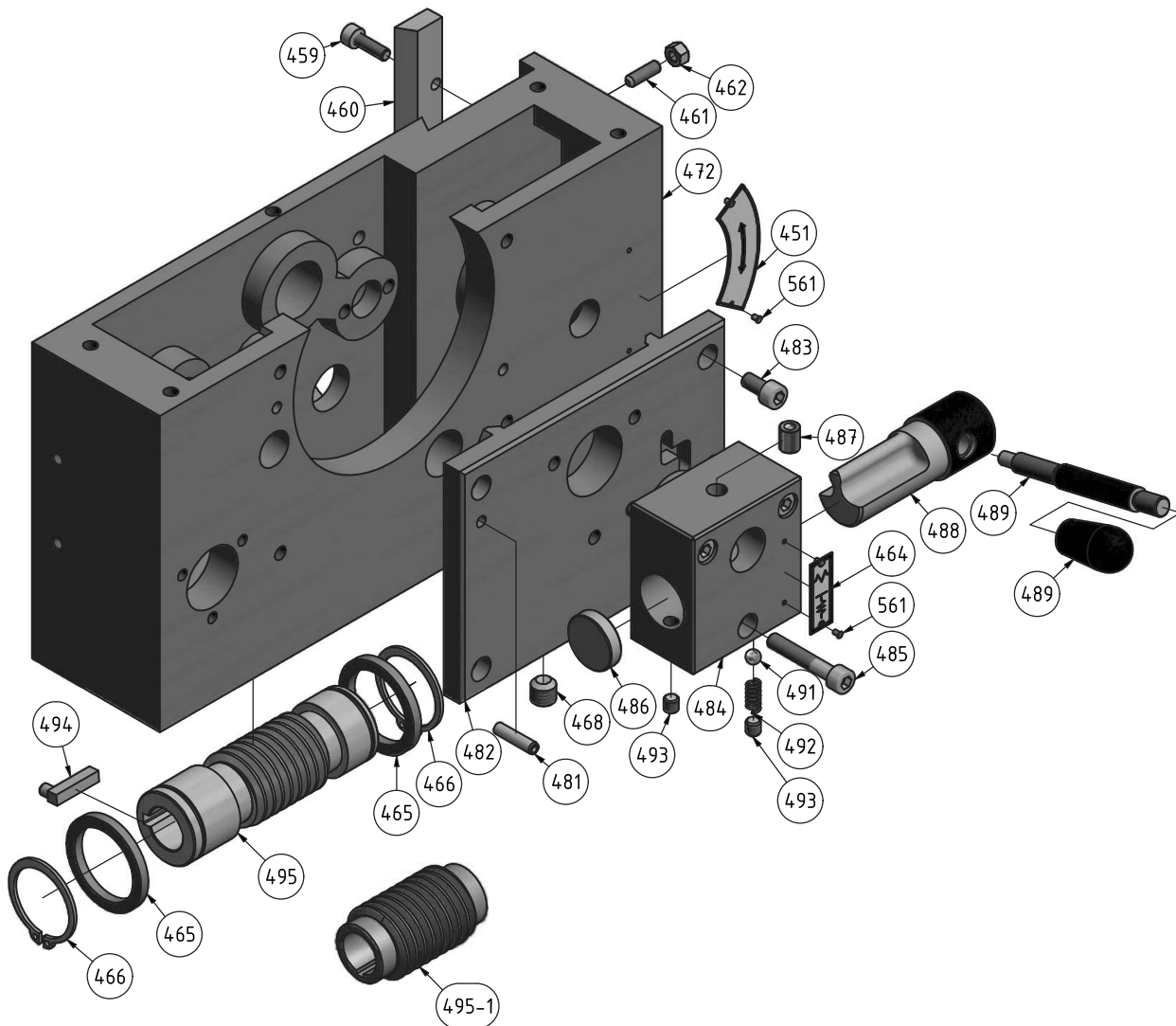
Img.1-17: Schlosskasten 1-3 - Apron 1-3
