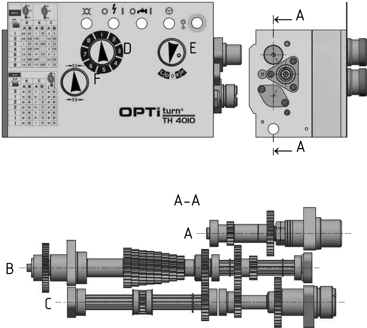
Abb.1-7: Vorschubgetriebe - Feed gear
