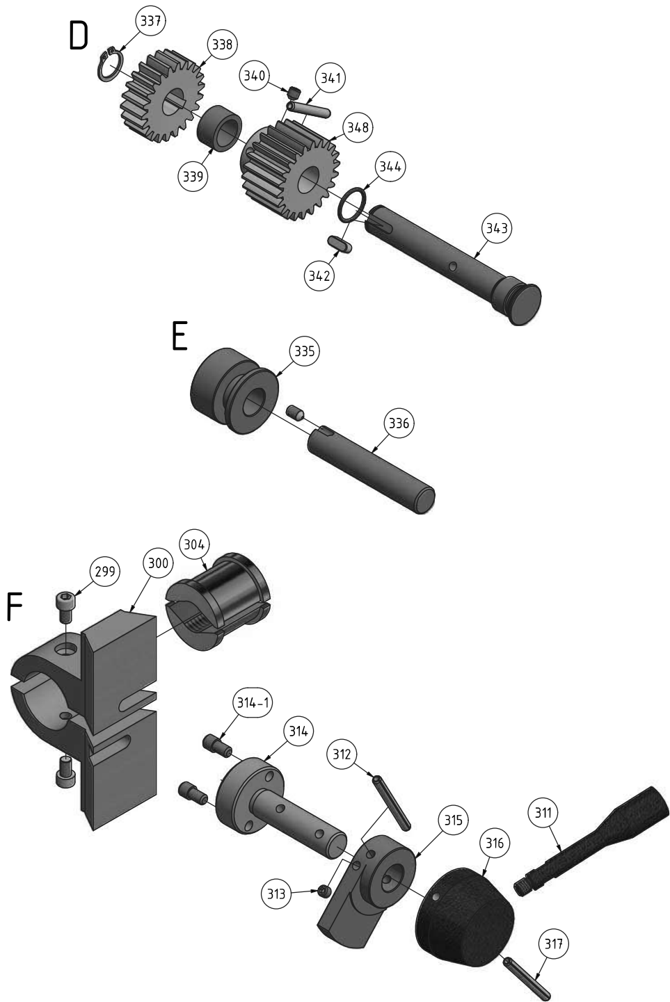
Abb. 1-13: Schlosskasten - Apron
