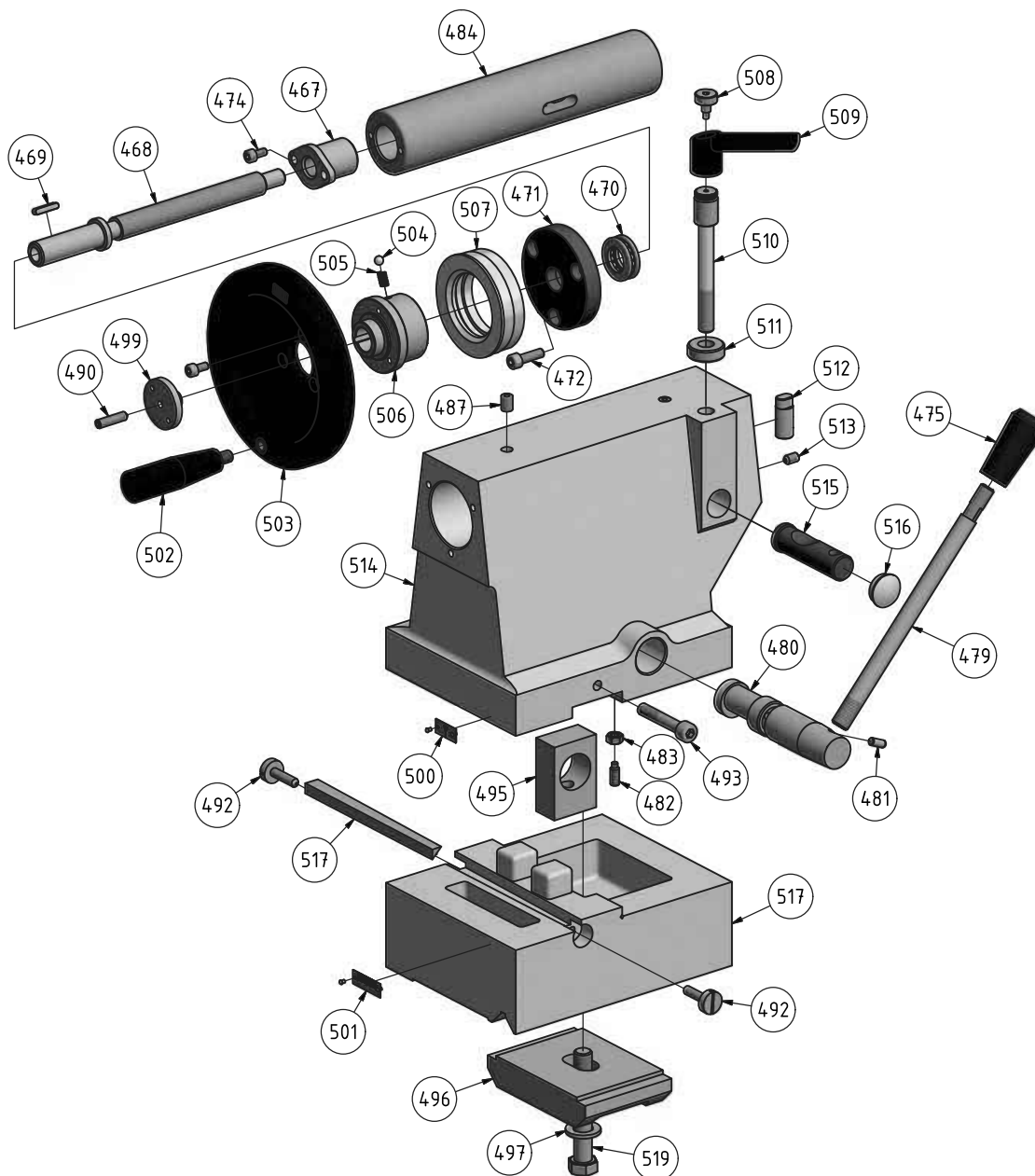
Abb. 1-16: Reitstock - Teilstock
