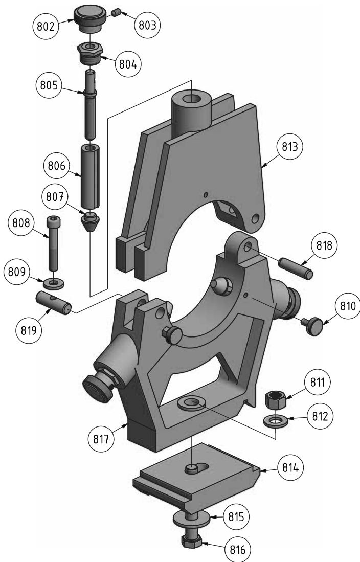
Abb. 1-17: Feststehende Lünette - Steady rest
