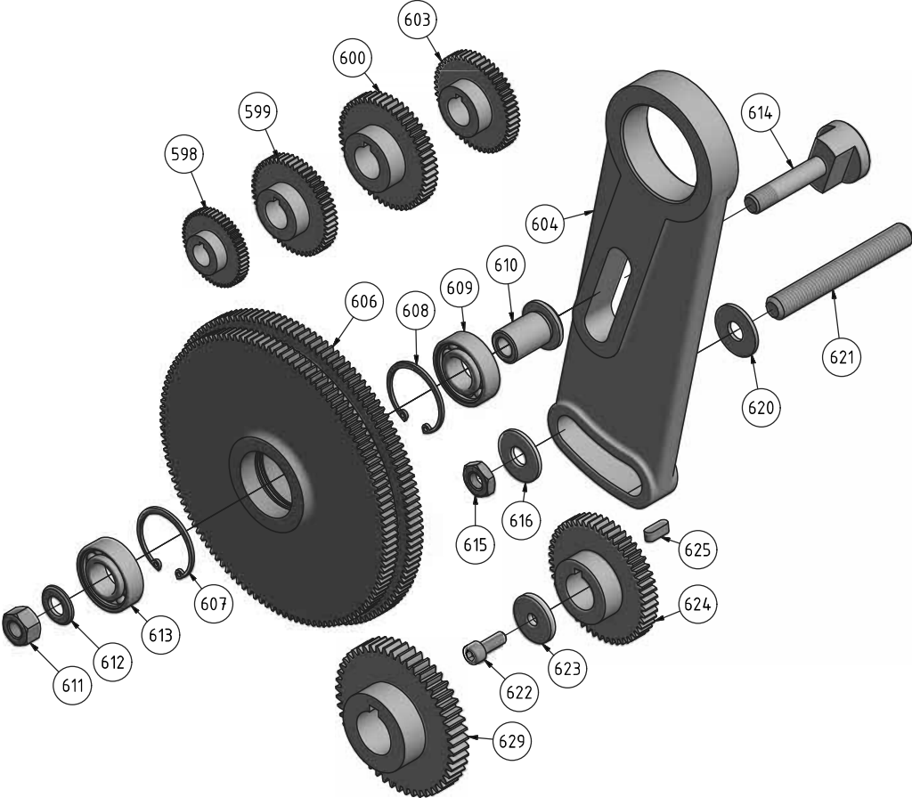
Abb.1-24: Wechselradgetriebe
