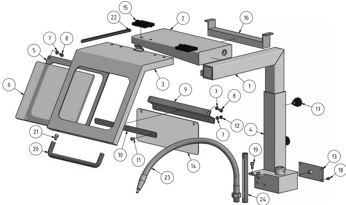
Abb.1-23: Späneschutz - Chip protection
