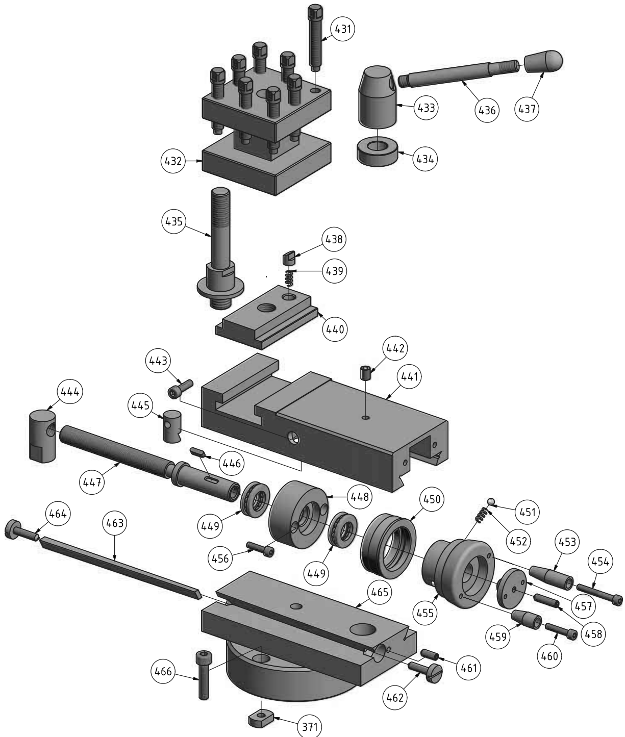
Abb. 1-15: Oberschlitten - Top slide
