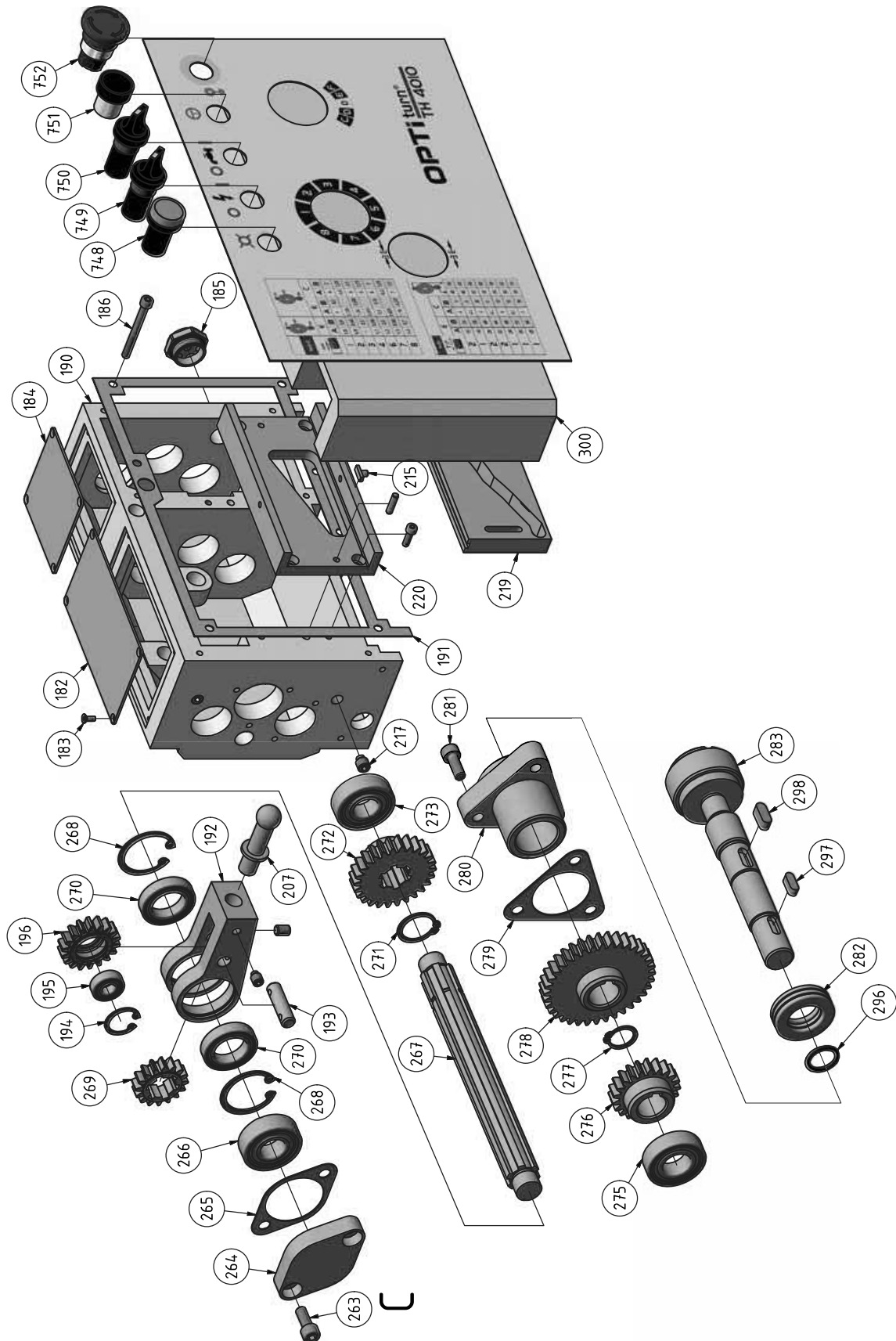
Abb. 1-9: Vorschubgetriebe - Feed gear
