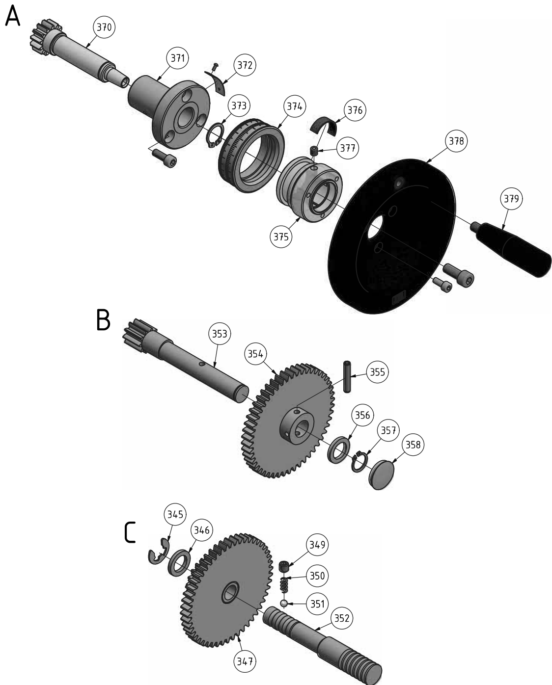
Abb.1-12: Schlosskasten - Apron
