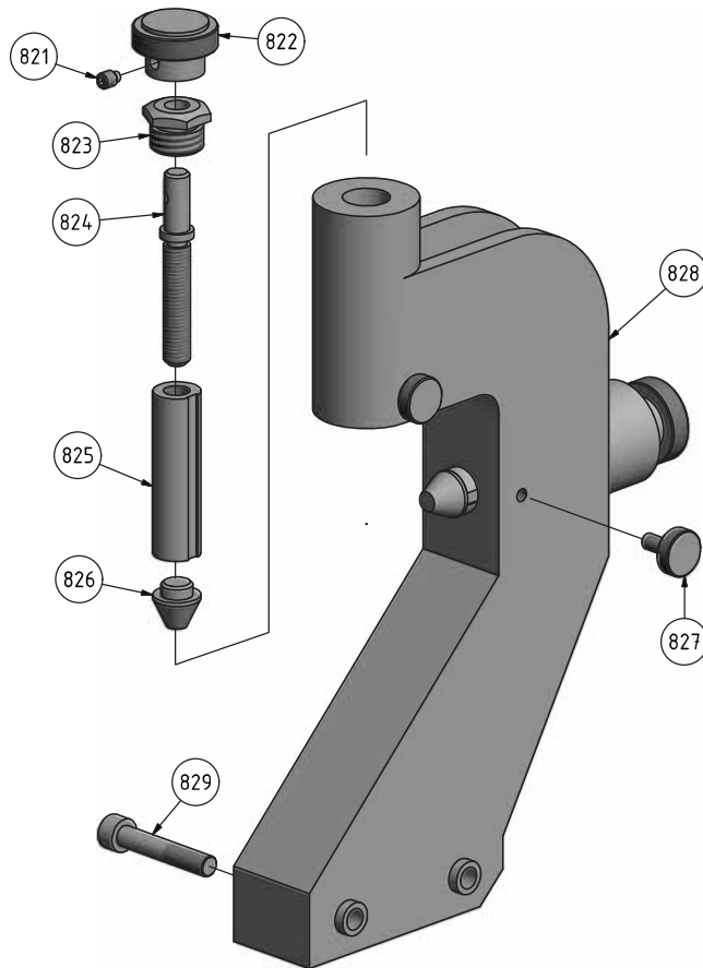
Abb. 1-18: Mitlaufende Lünette - Follow rest
