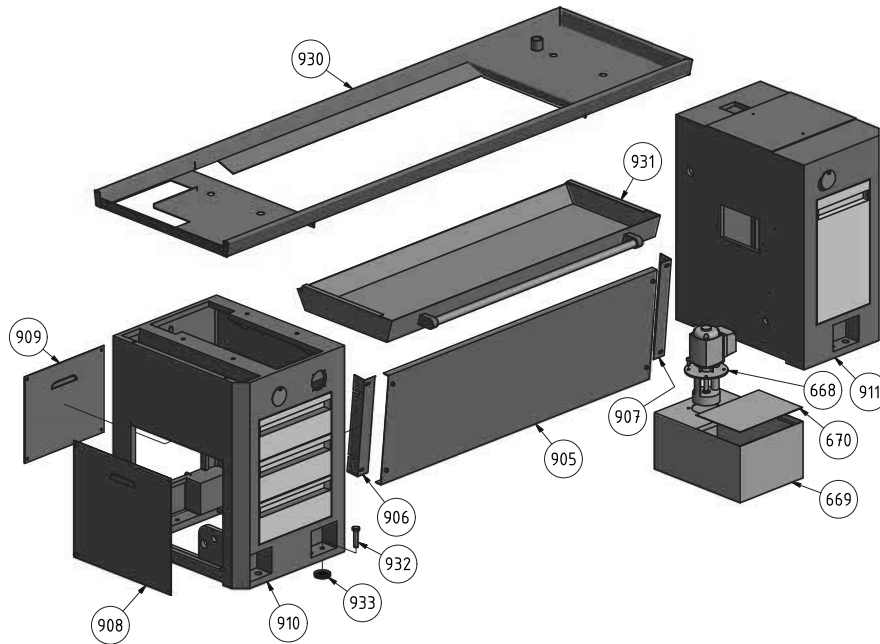
Abb. 1-21: Maschinenunterbau - Machine substructure
