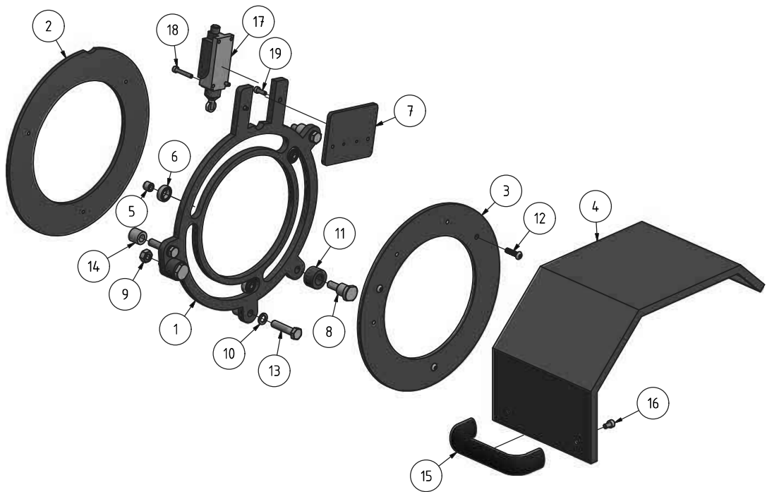
Abb. 1-22: Drehfutterschutz - Chuch protection
