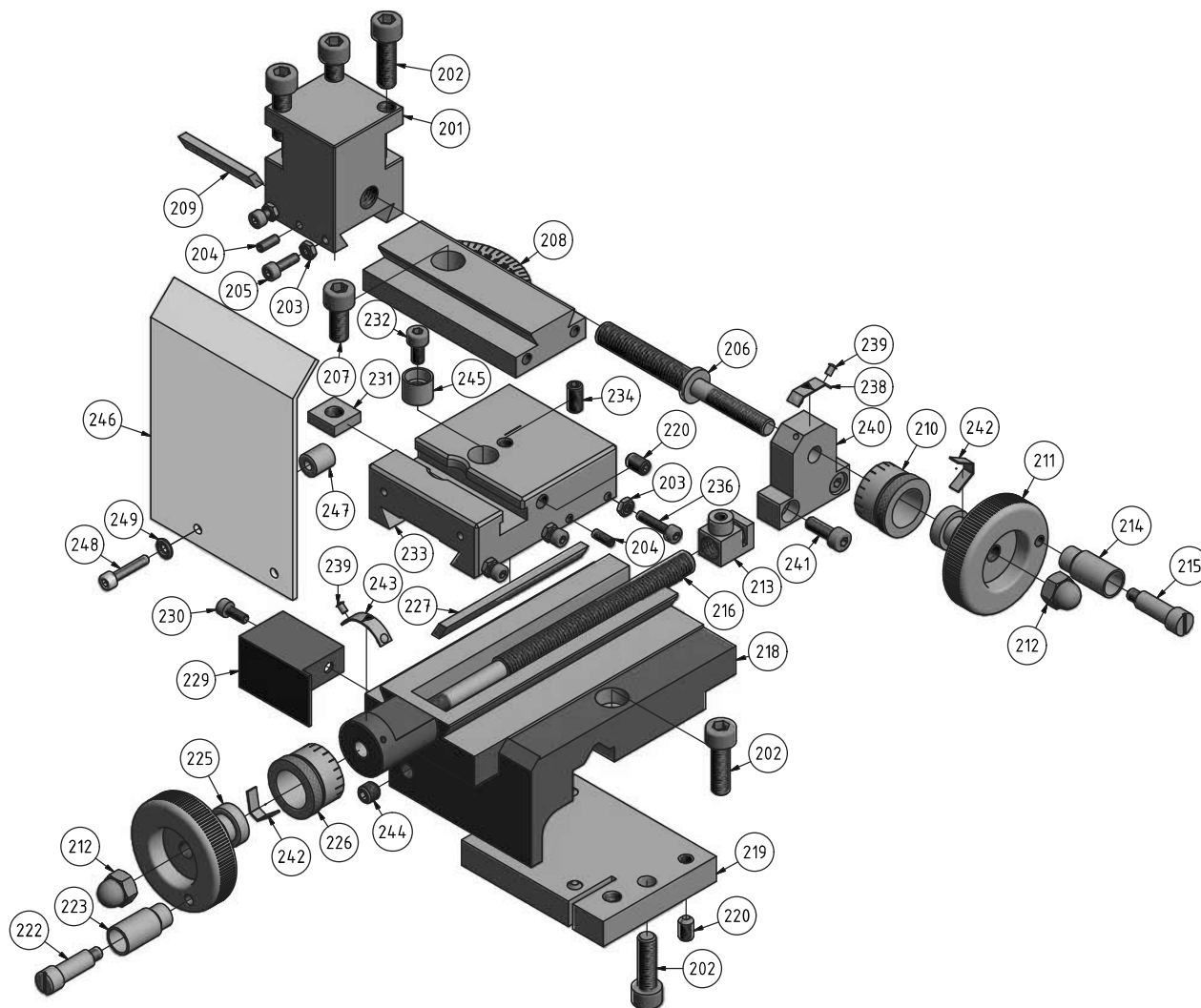
Ersatzteile Planschlitten, Oberschlitten - Spare parts list cross slide, top slide
