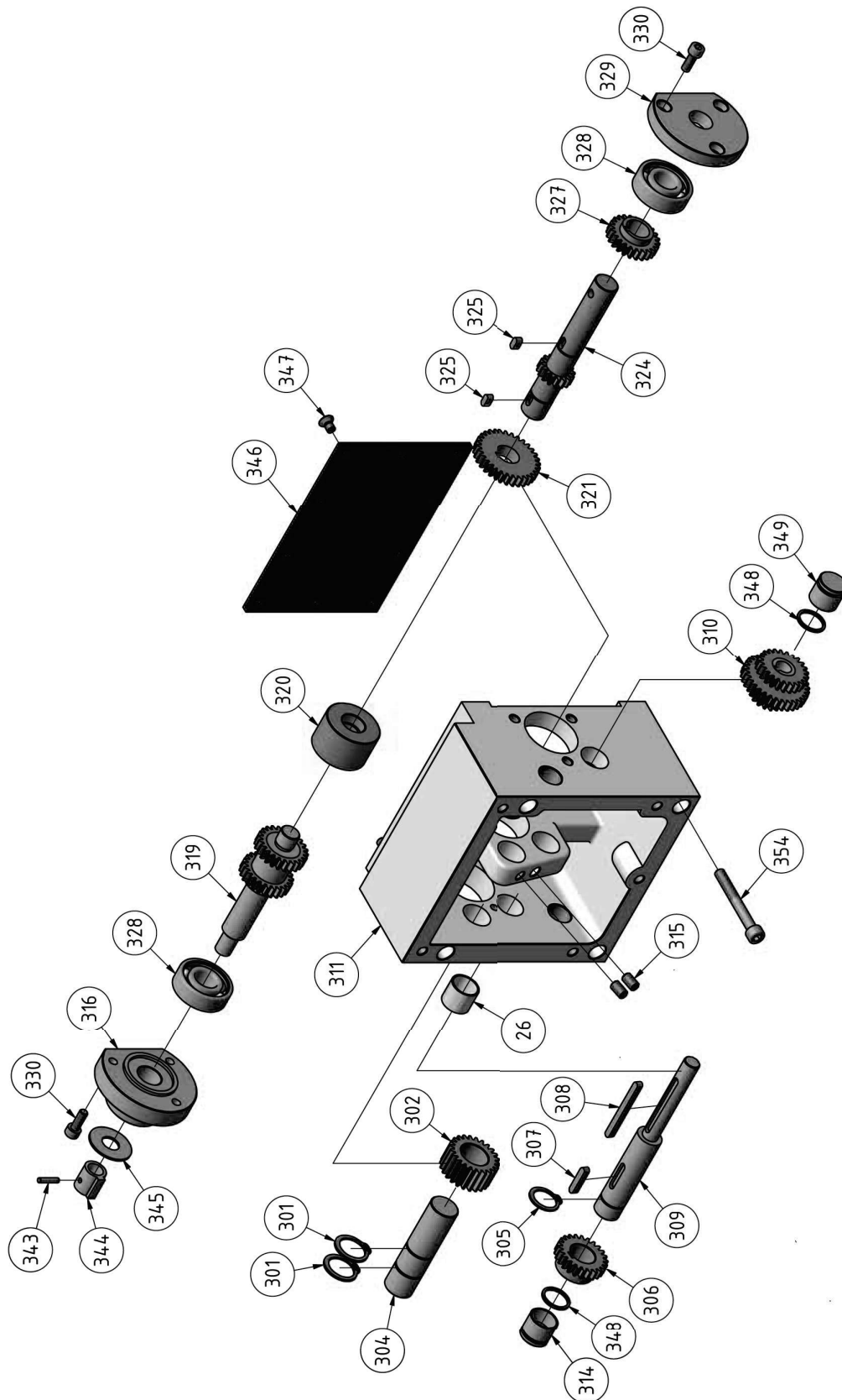
Abb.1-7: Vorschubgetriebe 2 von 2 - Feed gear 2 of 2 - TU2506
