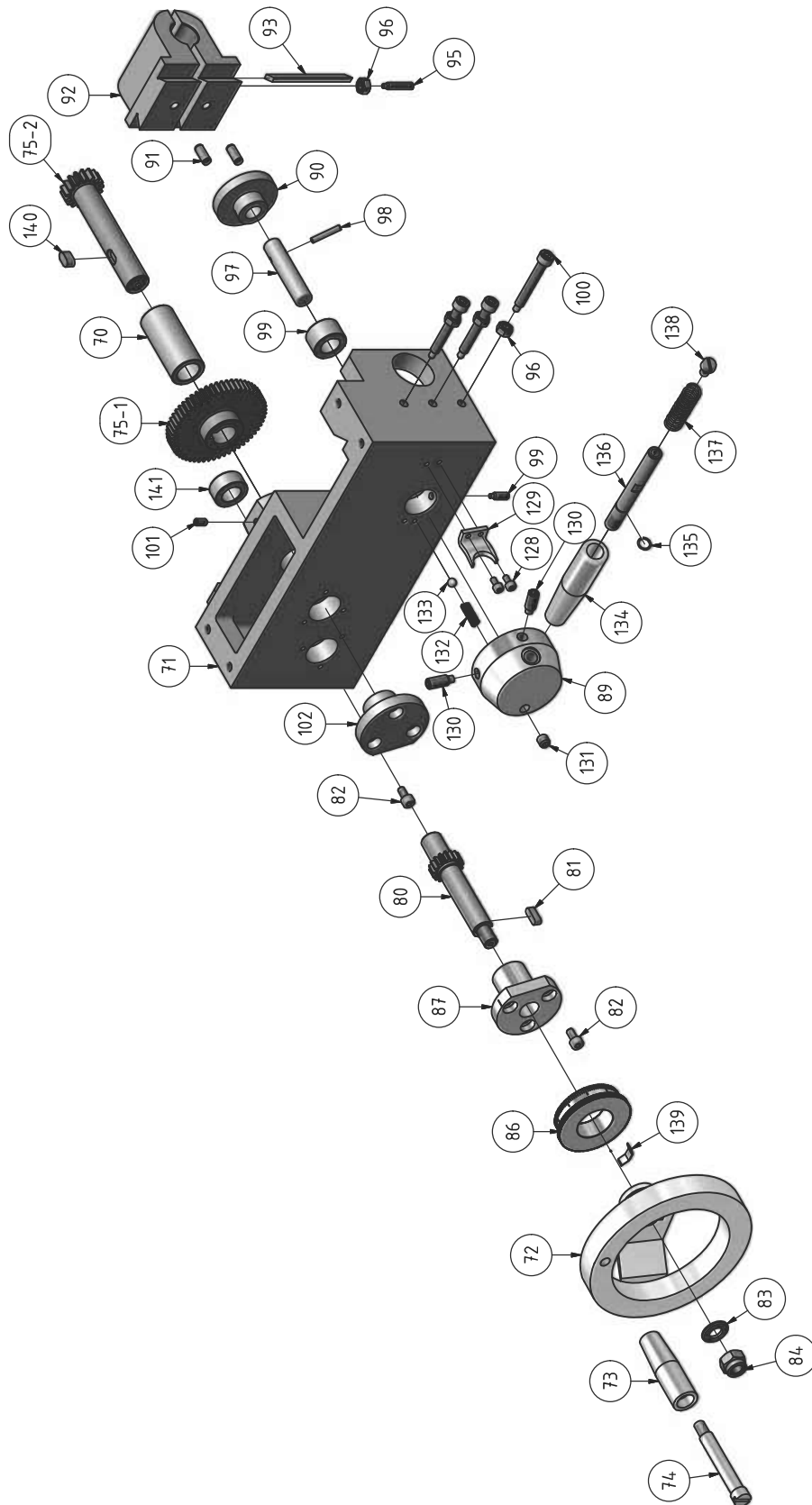
Abb. 1-3: Bettschlitten - Bed slide TU 2506
