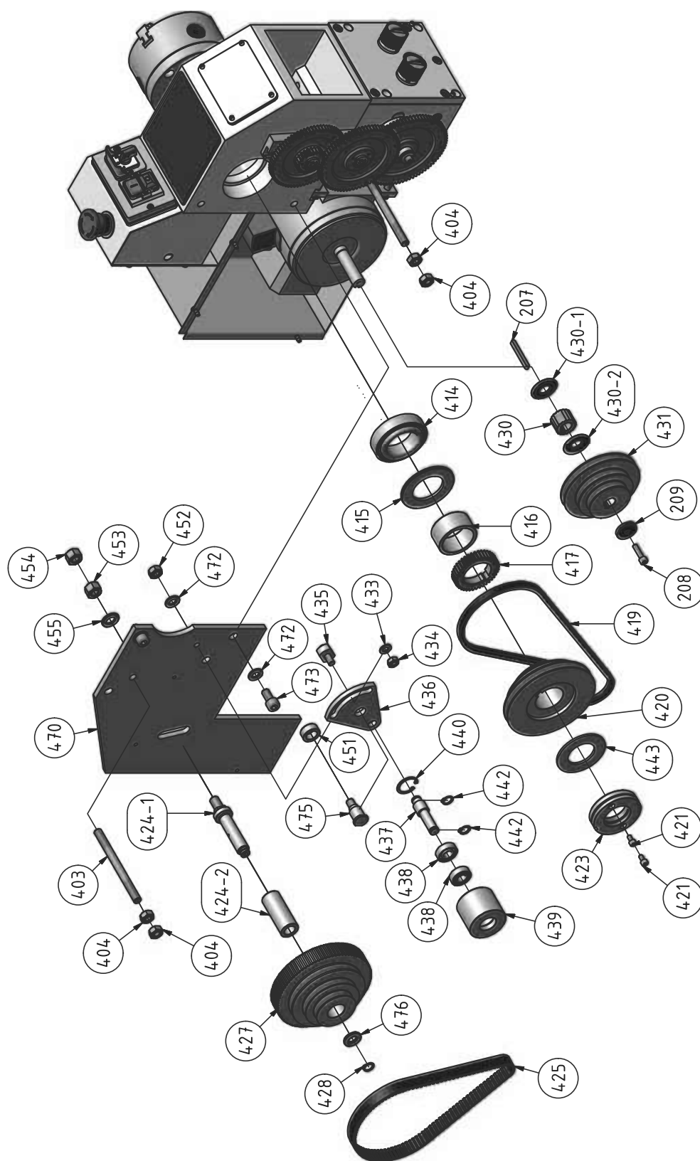
Abb. 1-8: Spindelstock 1 von 2 - Headstock 1 of 2 - TU2506
