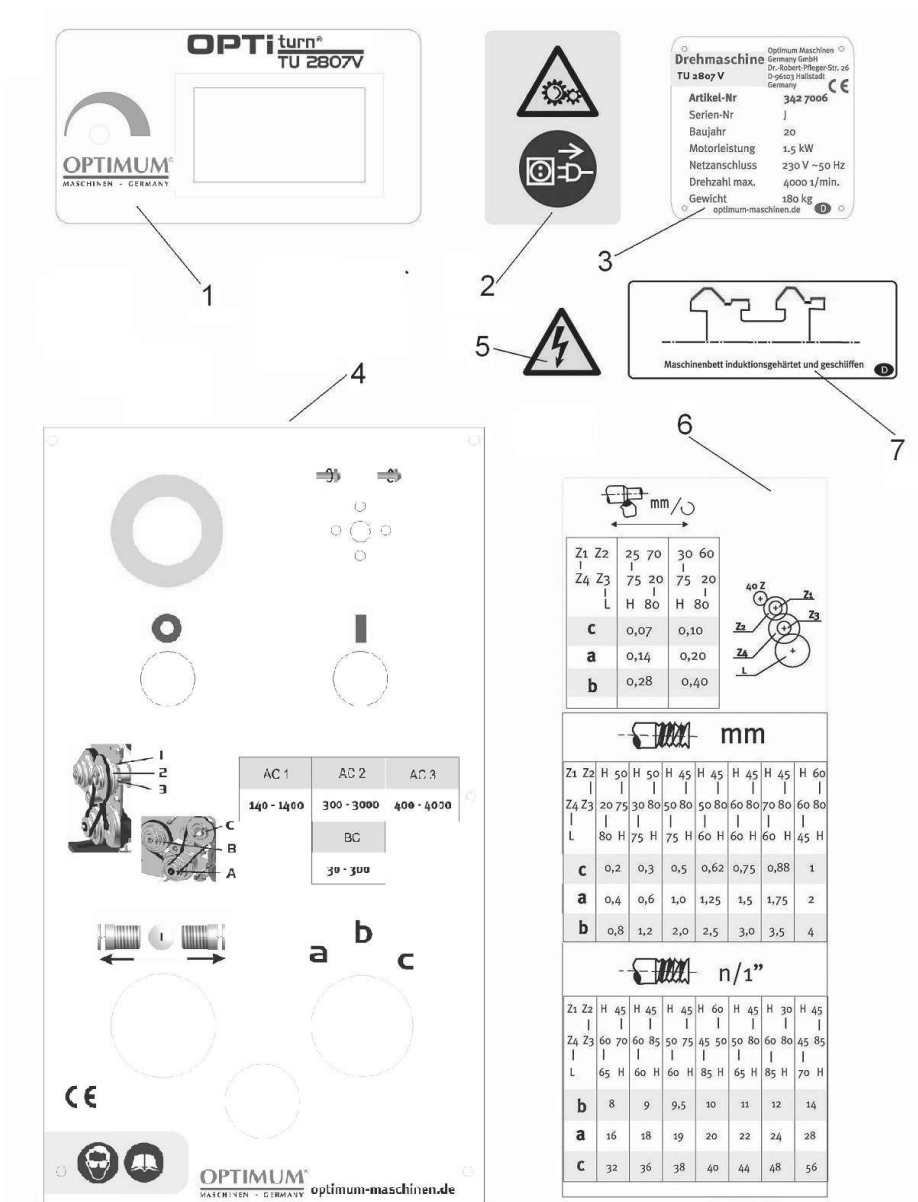
Abb. 1-26: Maschinenschilder - Machine labels
