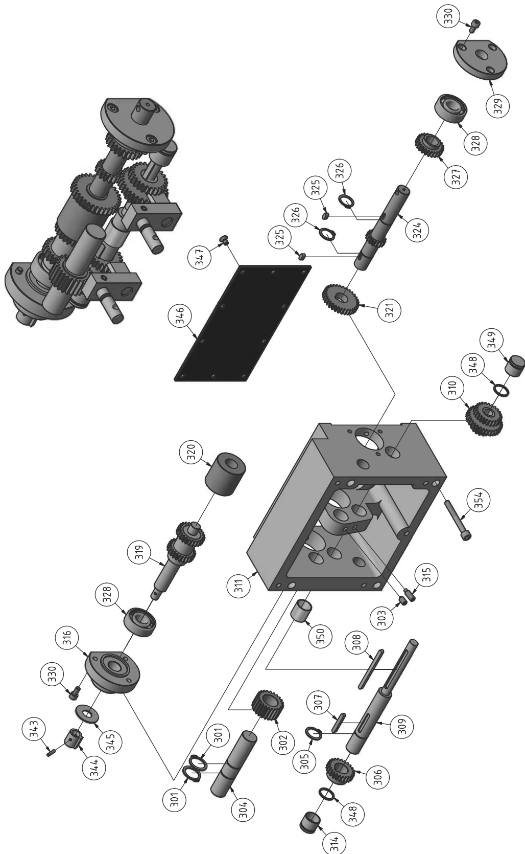
Abb.1-20: Vorschubgetriebe 2 von 2 - Feed gear 2 of 2 - TU 2807
