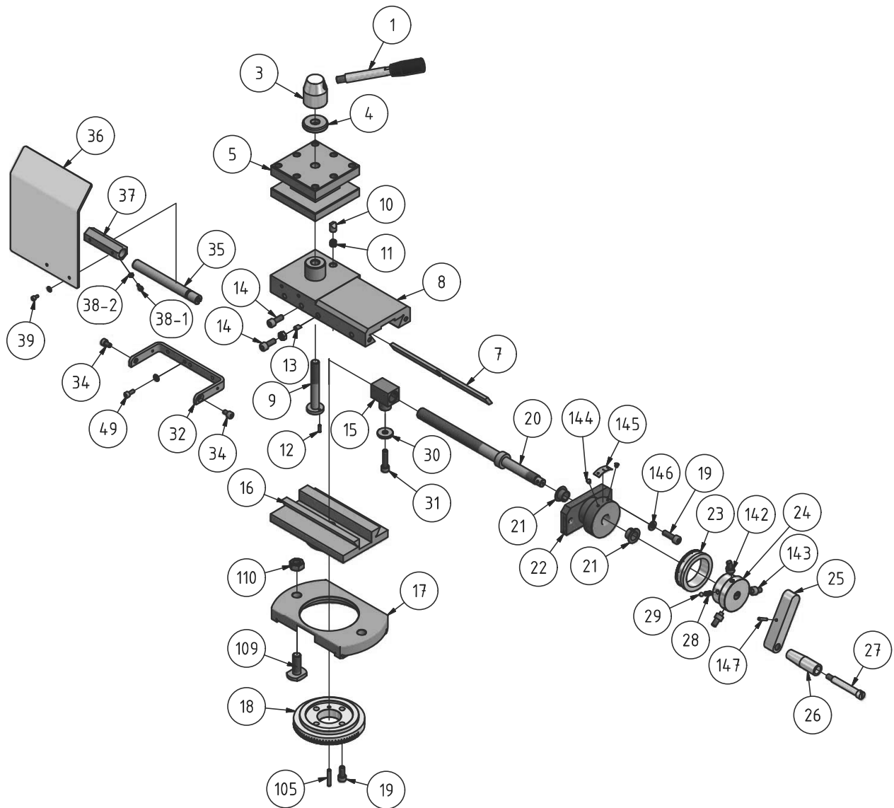
Abb.1-14: Oberschlitten - Top slide TU 2807
