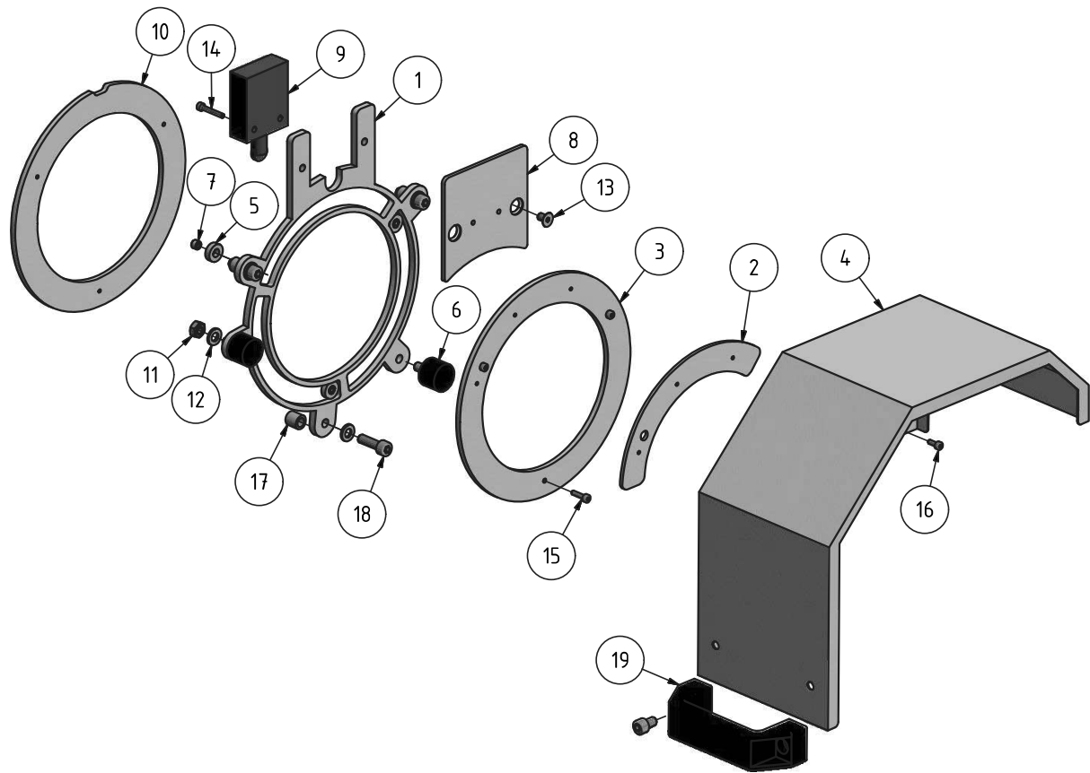
Abb.1-17: Drehfutterschutz - Lathe chuck cover
