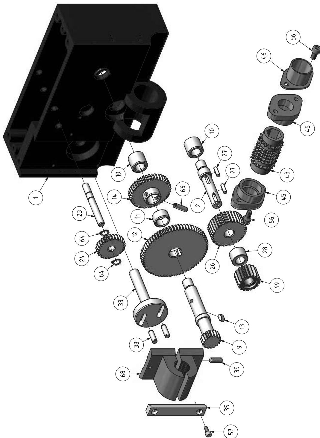
Abb. 1-10: Schlosskasten - Apron
