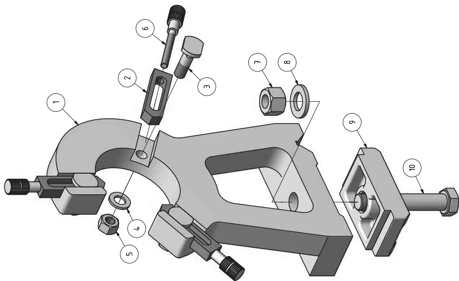
Abb. 1-16: Feststehende L nette - Fixed steady rest
