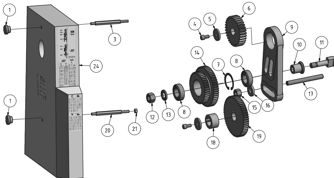
Img.1-3: Wechselradgetriebe - Change wheel gear
