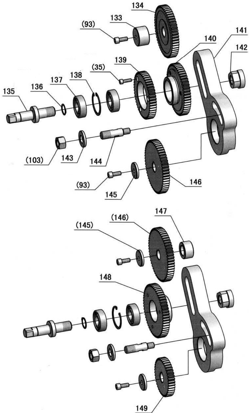
Img.1-26: Wechselradgetriebe (metrisch) - Change wheel gear (metric)
