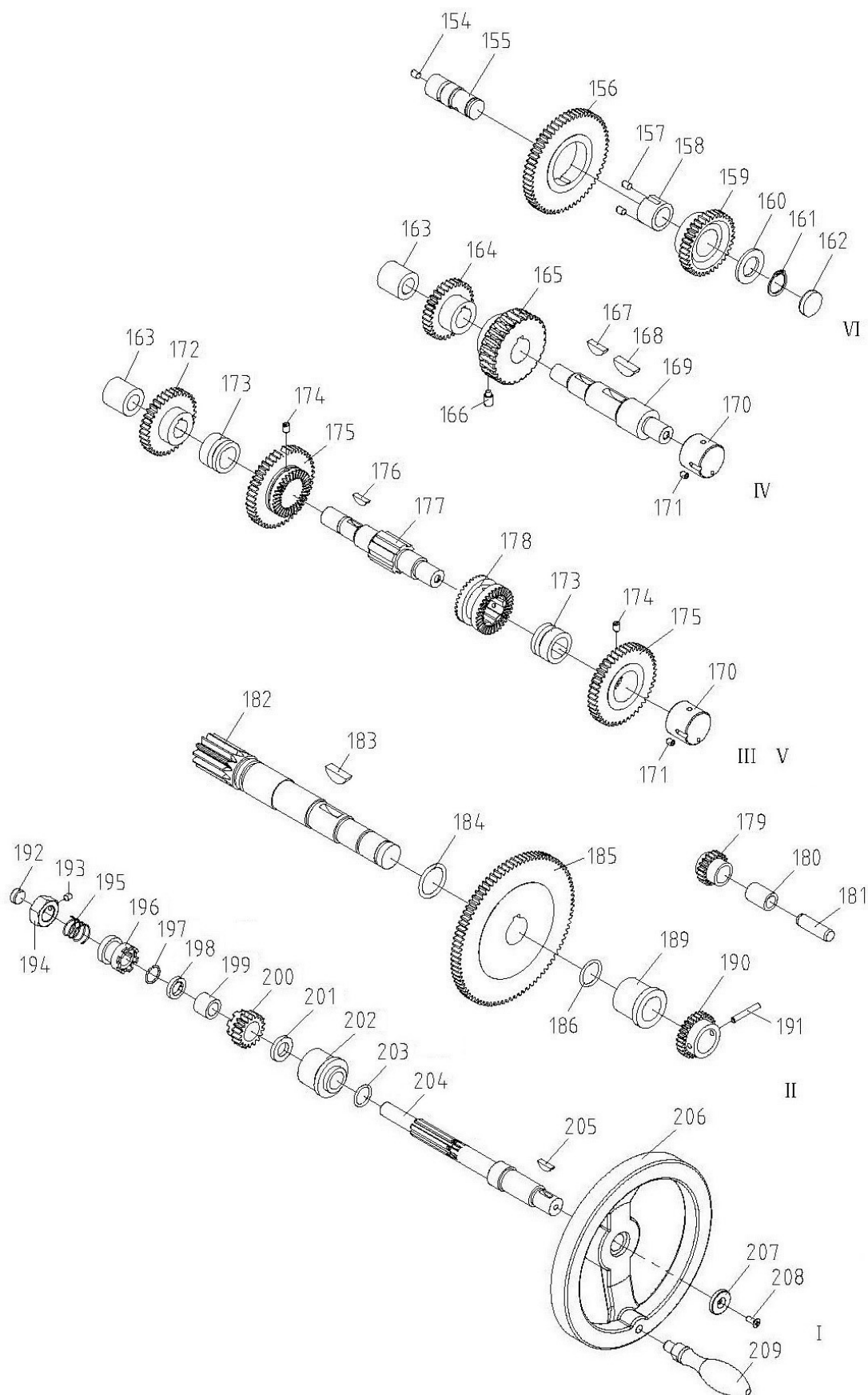
Img.1-22: Schlosskasten 3 von 3 - Apron 3 of 3
