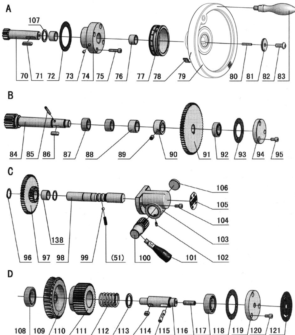
Img.1-18: Schlosskasten 2 von 2 - Apron 2 of 2
