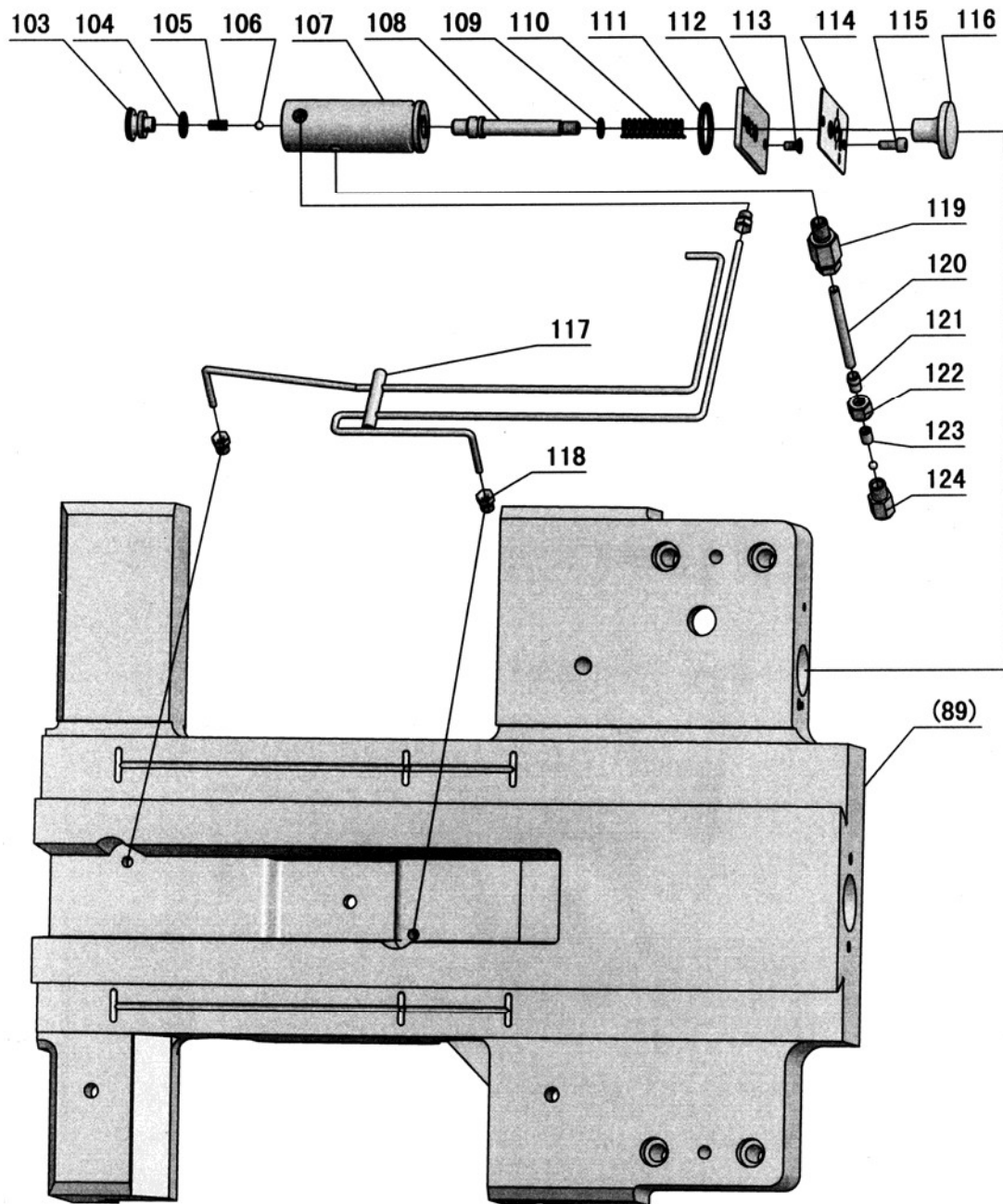
Img.1-16: Zentralschmierung - Central lubrication
