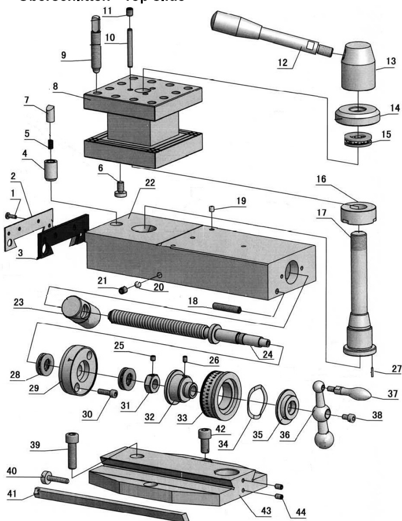
Img.1-14: Oberschlitten - Top slide
