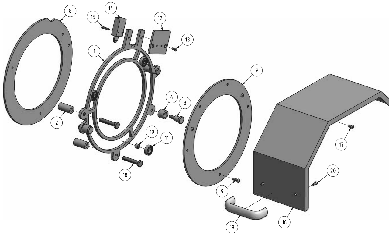
Img.1-28: Drehfutterschutz - Chuck protection
