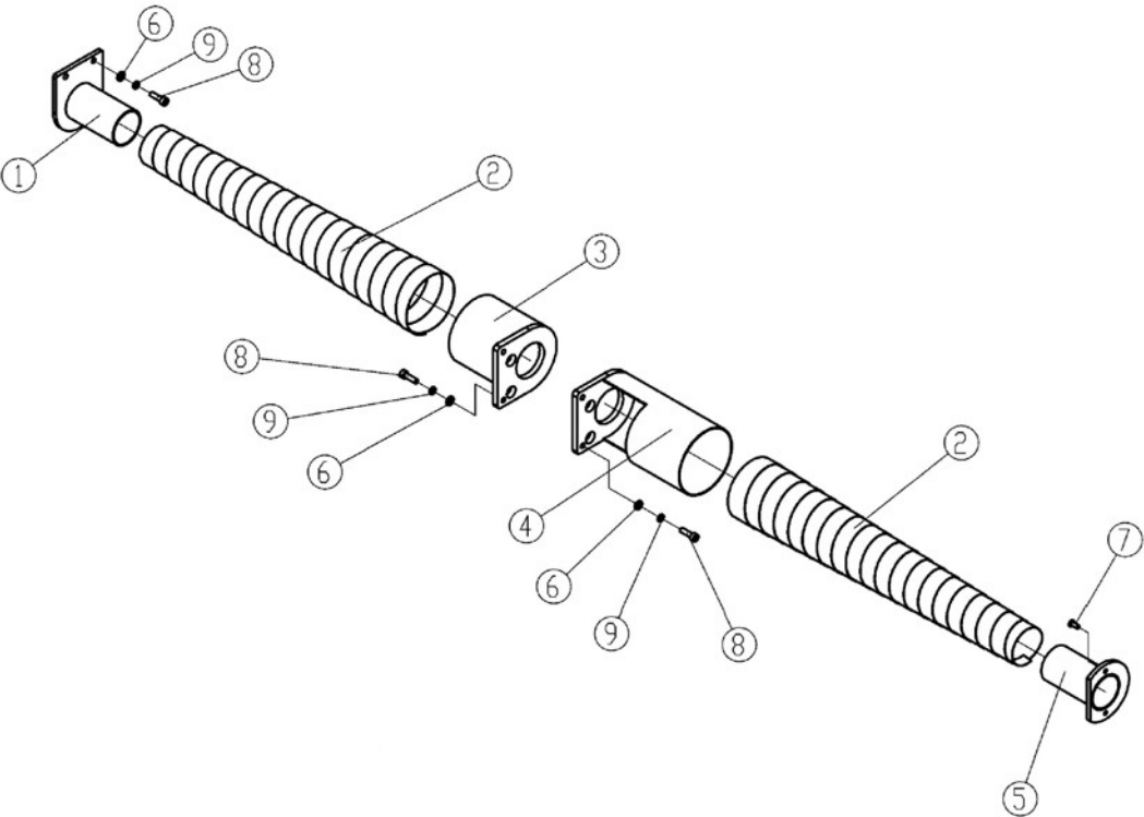
Img.1-30: Späneschutz - Chip protection
