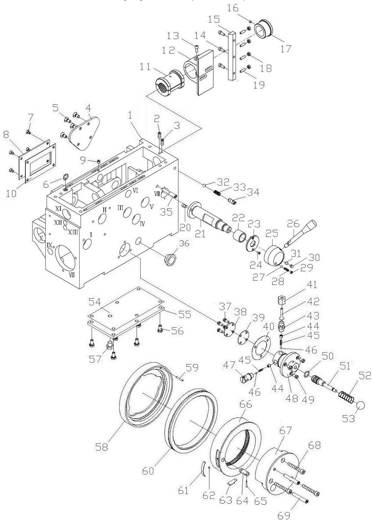
Img.1-20: Bettschlitten 1 von 3 - Apron 1 of 3
