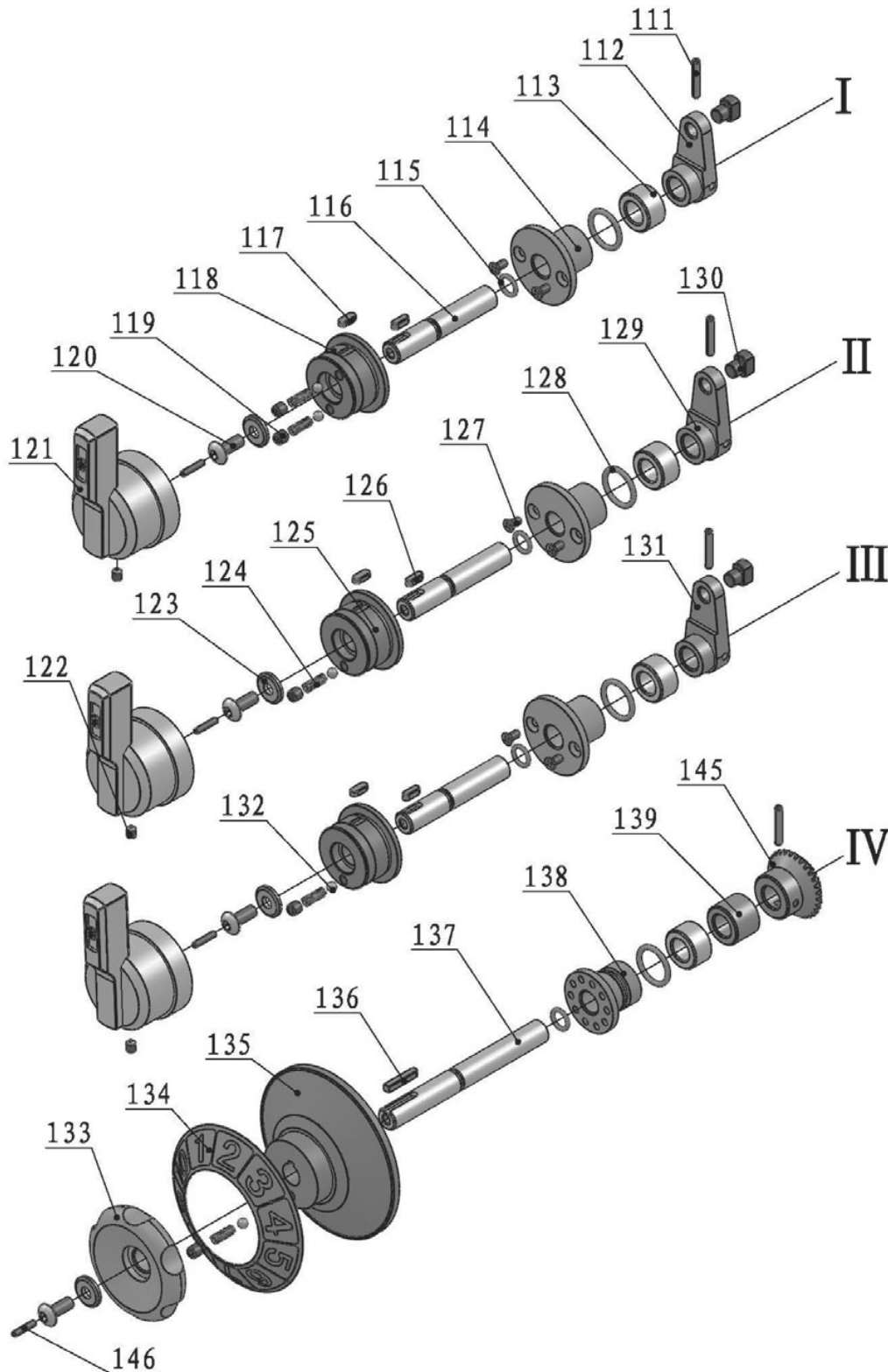
Img.1-13: Vorschubgetriebe 4 von 4 - Headstock feed gear 4 of 4
