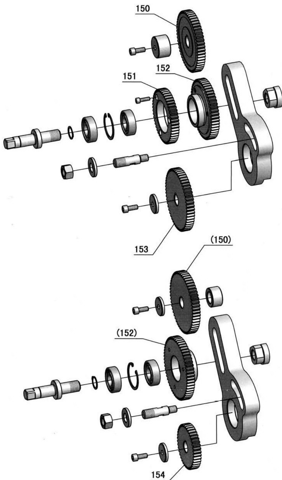
Img.1-27: Wechselradgetriebe (Inch) - Change wheel gear (Inch)
