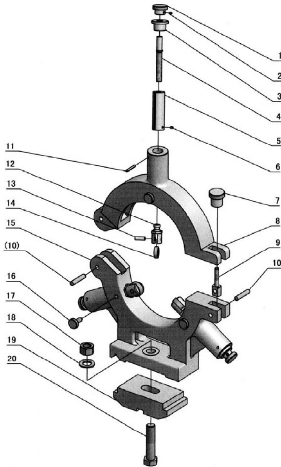
Img.1-32: Fest stehende Lünette - Steady rest
