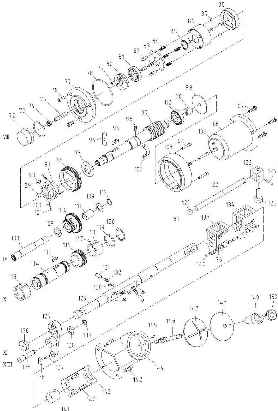
Img.1-21: Schlosskasten 2 von 3 - Apron 2 of 3
