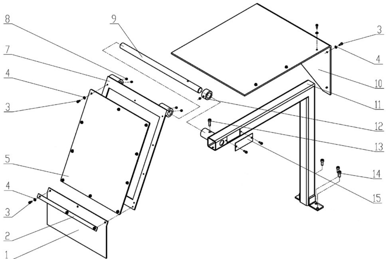
Img. 1-29: Späneschutz - Chip protection
