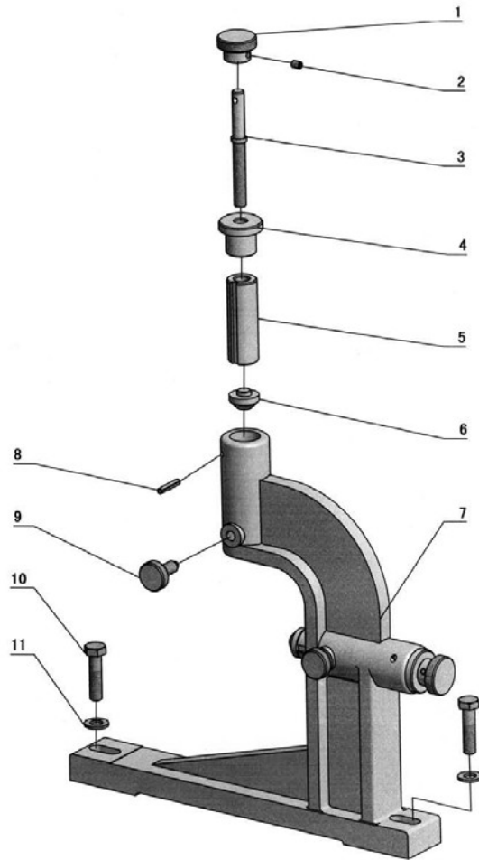
Img.1-33: Mitlaufende Lünette - Follow rest
