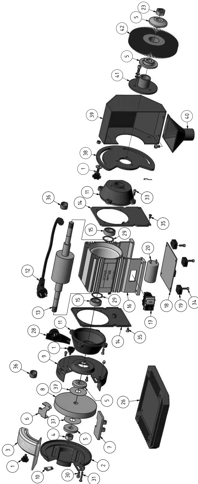
1-1: Ersatzteilzeichnung - Spare parts drawing
