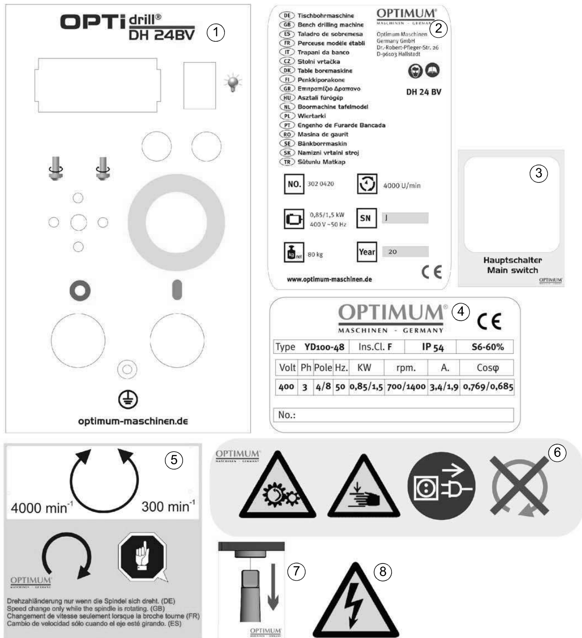
Abb.1-6: Maschinenschilder - Machine labels
