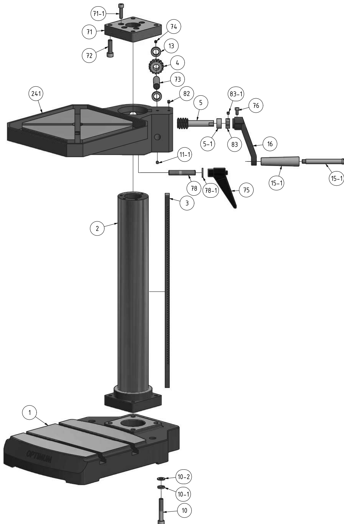
Abb. 1-2: Säule und Bohrtisch DH24BV - Column and drilling table DH24BV
