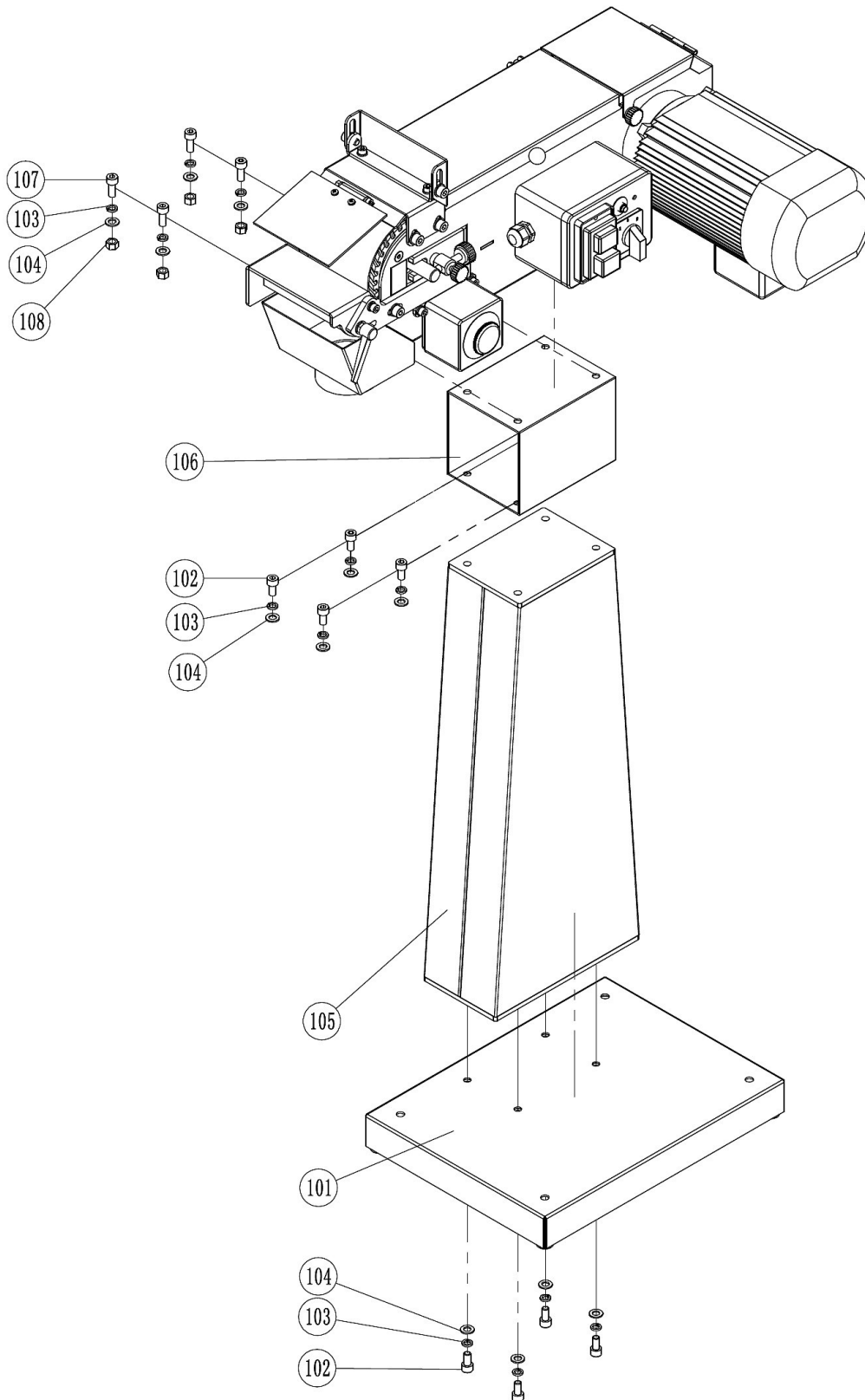
Abb. / Fig. 1: Ersatzteilzeichnung 1 MBSM 100-140-1 230V und MBSM 100-140-2 400V / Spare parts drawing 1 MBSM 100-140-1 230V and MBSM 100-140-2 400V
