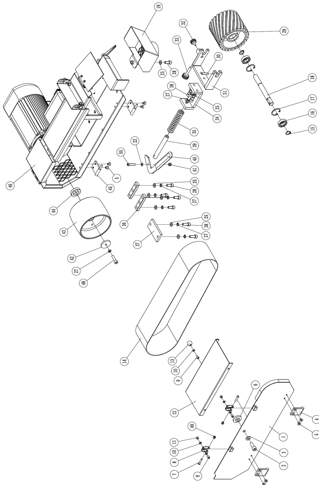
Abb. / Fig. 2: Ersatzteilzeichnung 2 MBSM 100-140-1 230V und MBSM 100-140-2 400V Spare parts drawing 2 MBSM 100-140-1 230V and MBSM 100-140-2 400V
