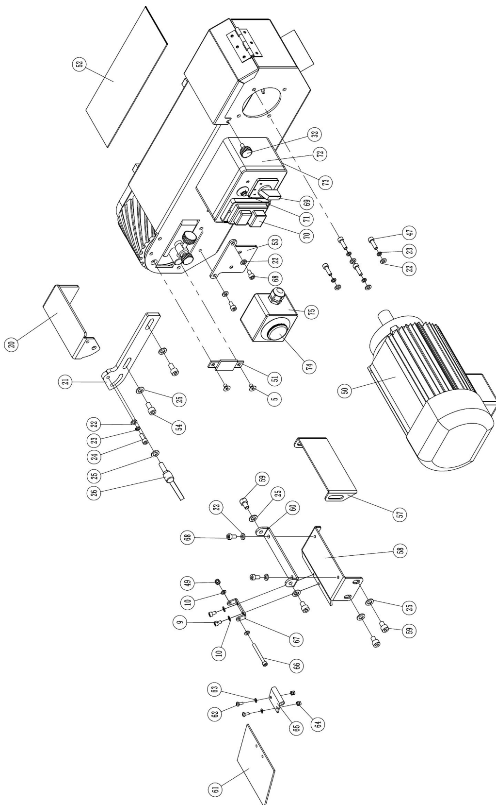
Abb./Fig. 3: Ersatzteilzeichnung 3 MBSM 100-140-1 230V und MBSM 100-140-2 400V Spare parts drawing 3 MBSM 100-140-1 230V and MBSM 100-140-2 400V
