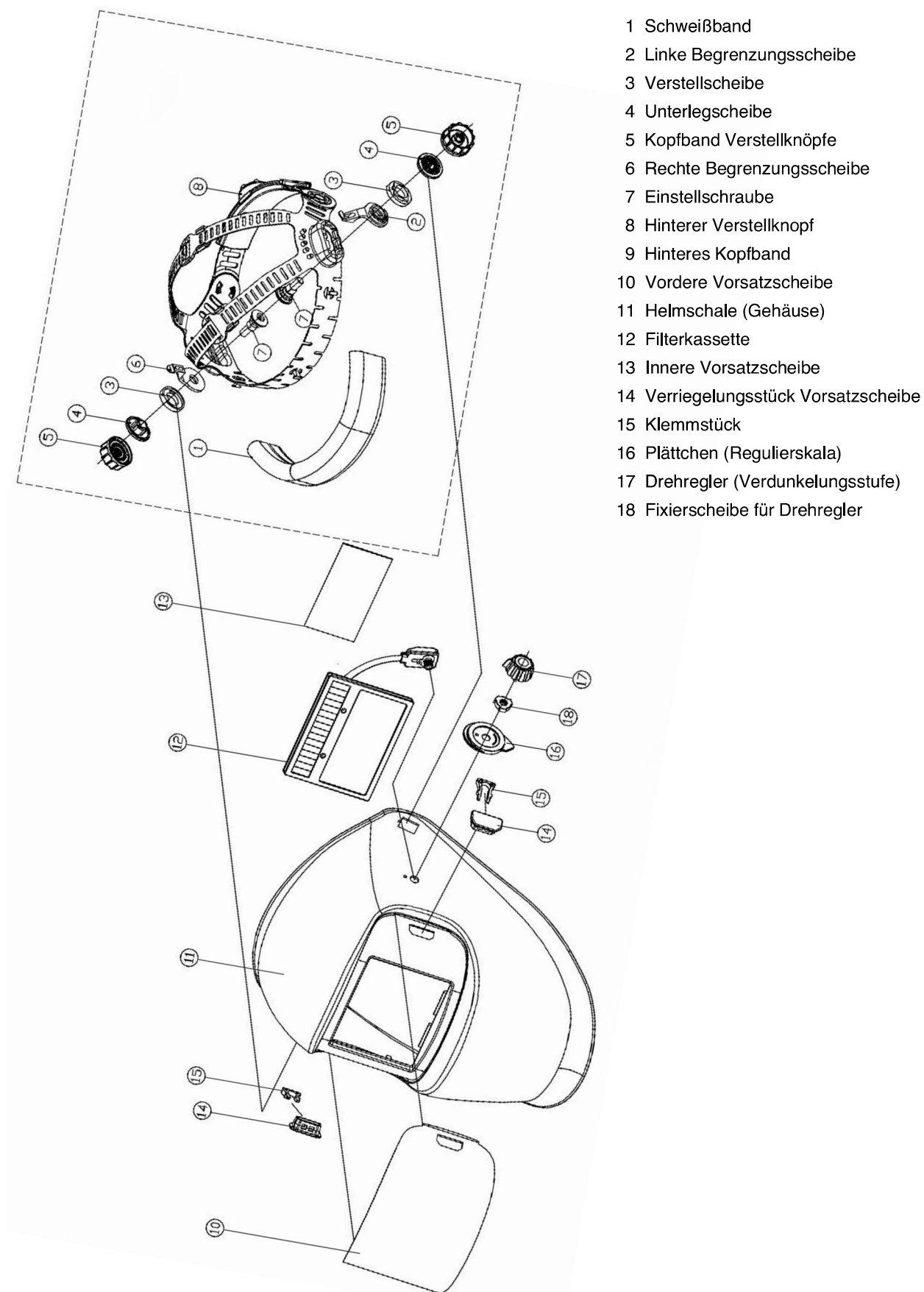
Abb. / Fig. 2: Ersatzteilzeichnung 2 / Spare parts drawing 2
