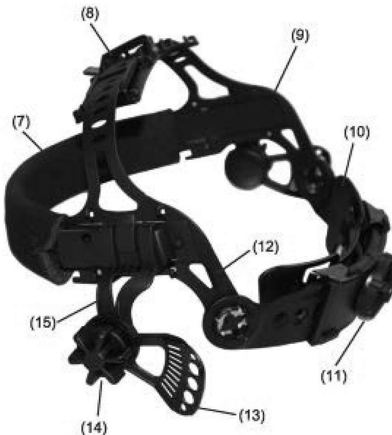
Abb./Fig. 2: Ersatzteilzeichnung 2 / Spare parts drawing 2
