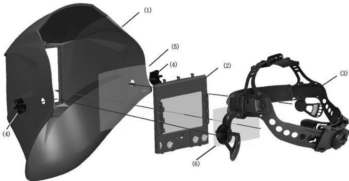
Abb./Fig. 1: Ersatzteilzeichnung 1 / Spare parts drawing 1
