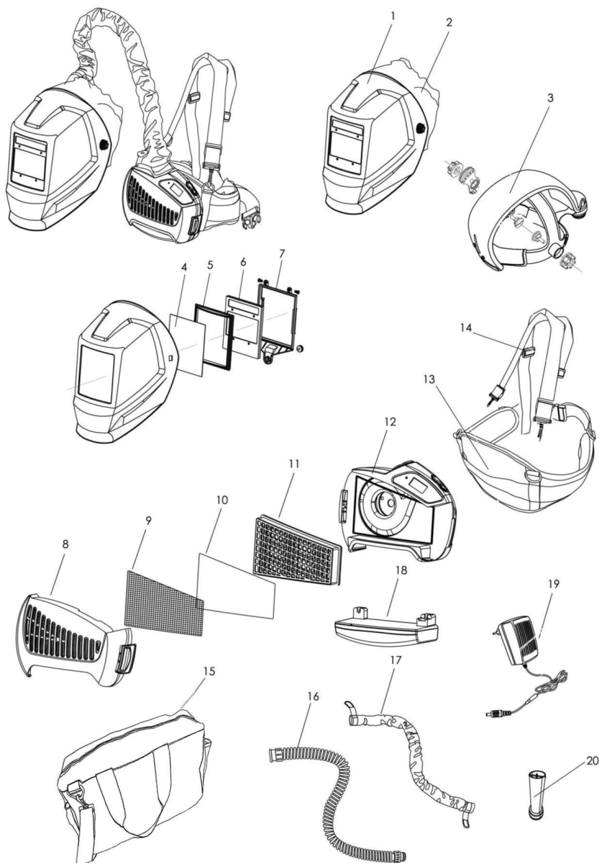
Abb./Fig. 2: Ersatzteilzeichnung 2 / Spare parts drawing 2
