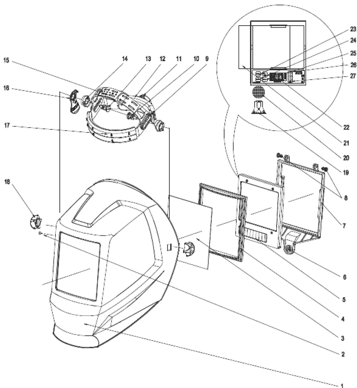
Abb./Fig. 1: Ersatzteilzeichnung 1 / Spare parts drawing 1
