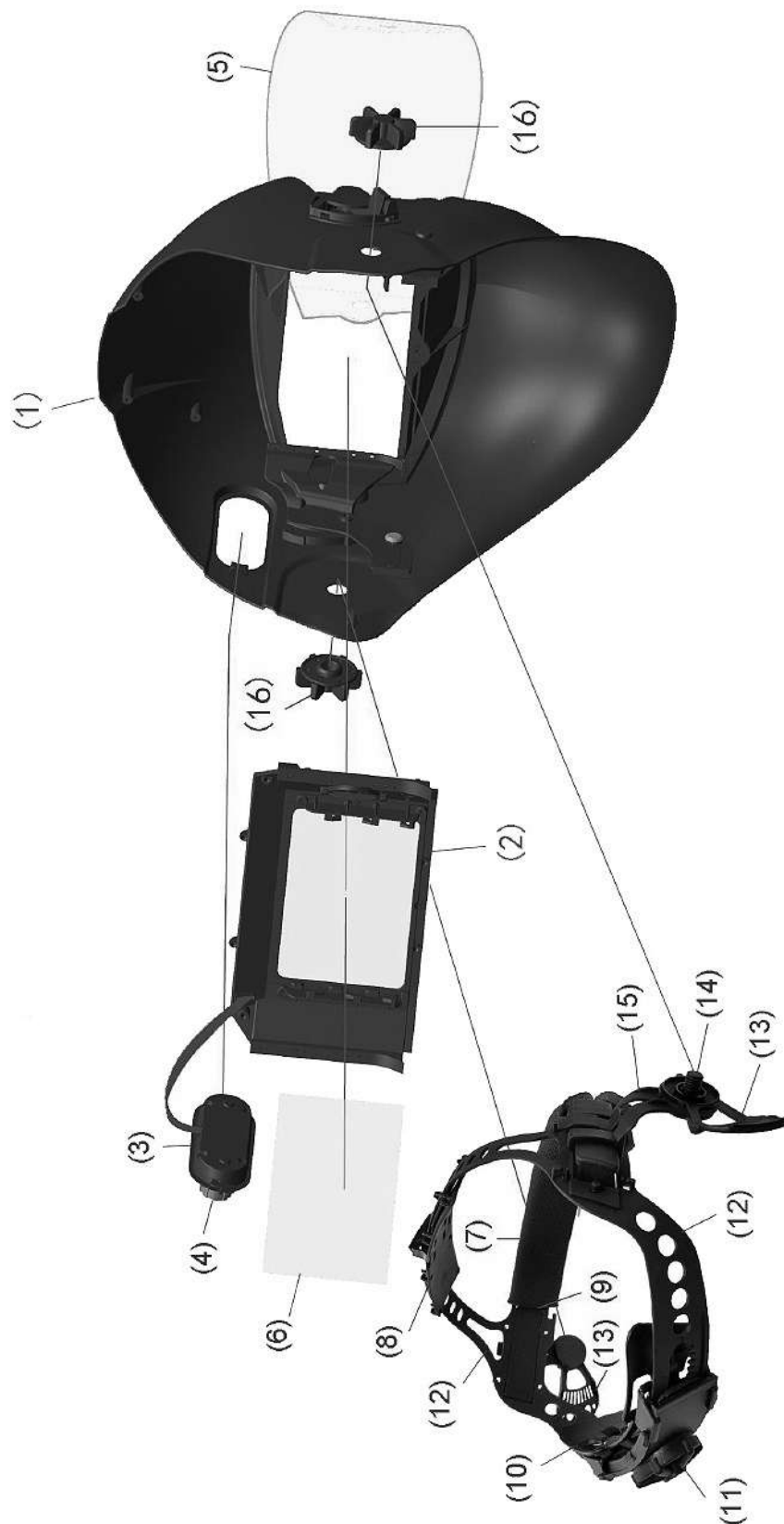
Abb./Fig. 1: Ersatzteilzeichnung 1 / Spare parts drawing 1 VarioProtect XXL-W_F-TC
