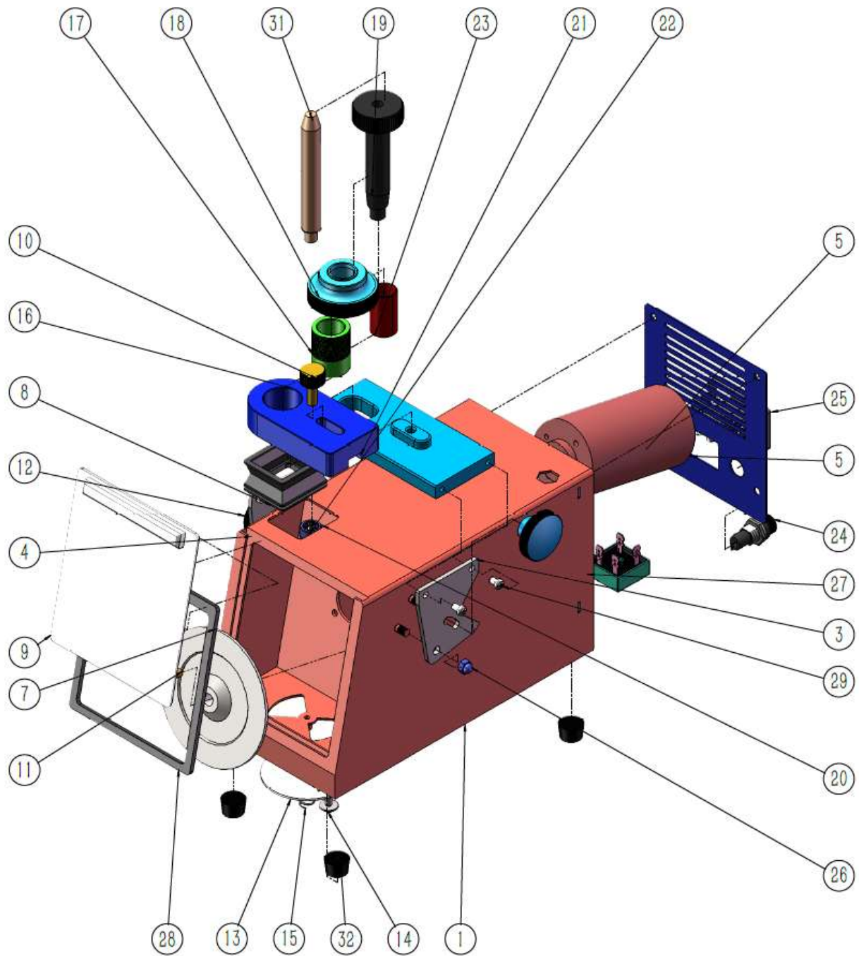
Abb. / Fig. 1: Ersatzteilzeichnung EG 5 / Spare parts drawing EG 5
