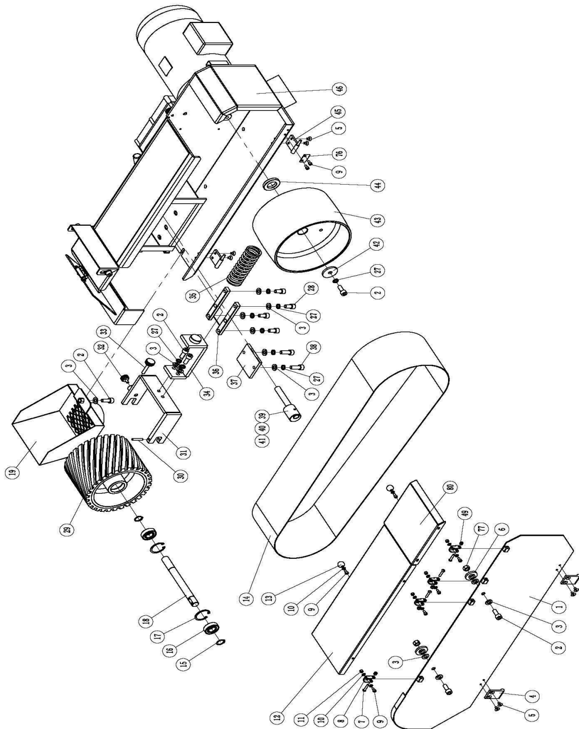
Abb. 24: Ersatzteilzeichnung 2 MBSM 75-203-2 AS/400V, MBSM 150-203-2 AS/400V
