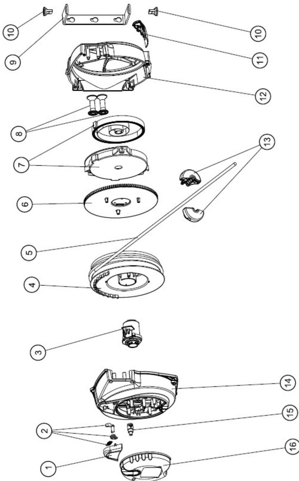
Abb.7-1: Ersatzteilzeichnung
