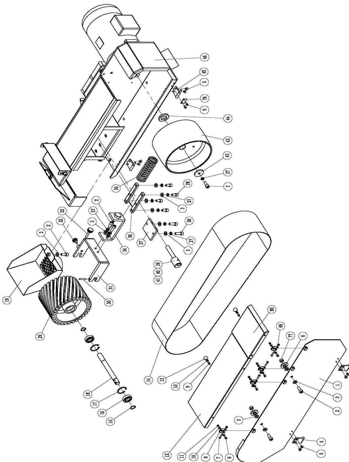
Abb. 27: Ersatzteilzeichnung 2 MBSM 75-240-2 AS/400V, MBSM 150-240-2 AS/400V
