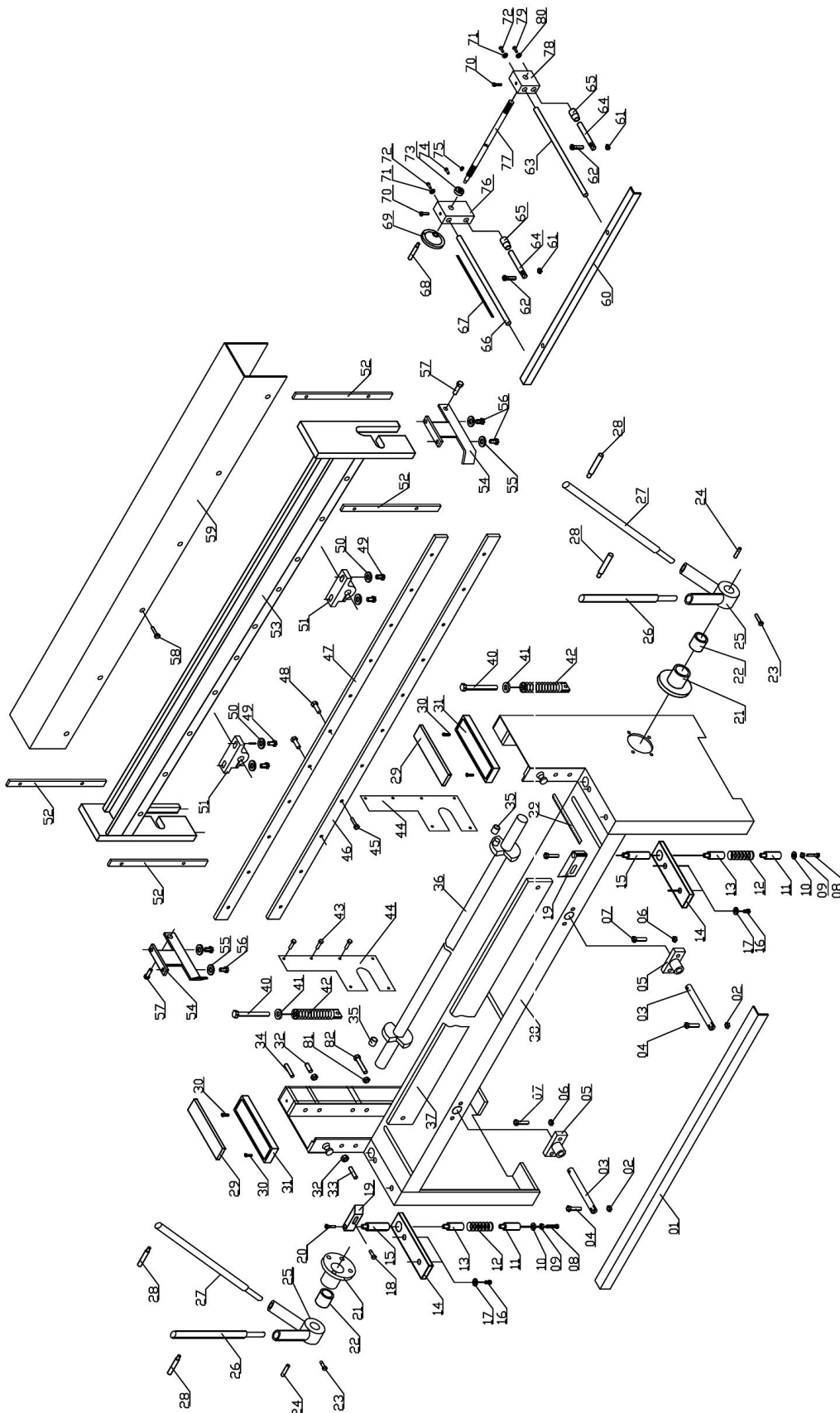
Abb.9-1: Ersatzteilzeichnung
