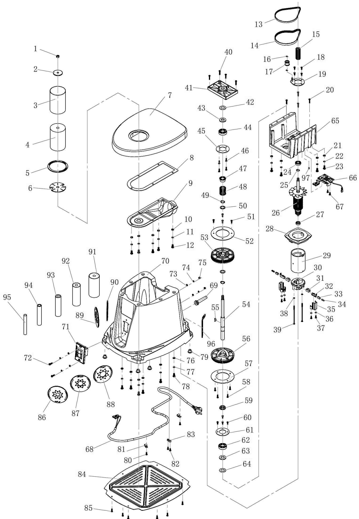
Abb. 1: Ersatzteilzeichnung OSS 100 / Spare parts drawing OSS 100
