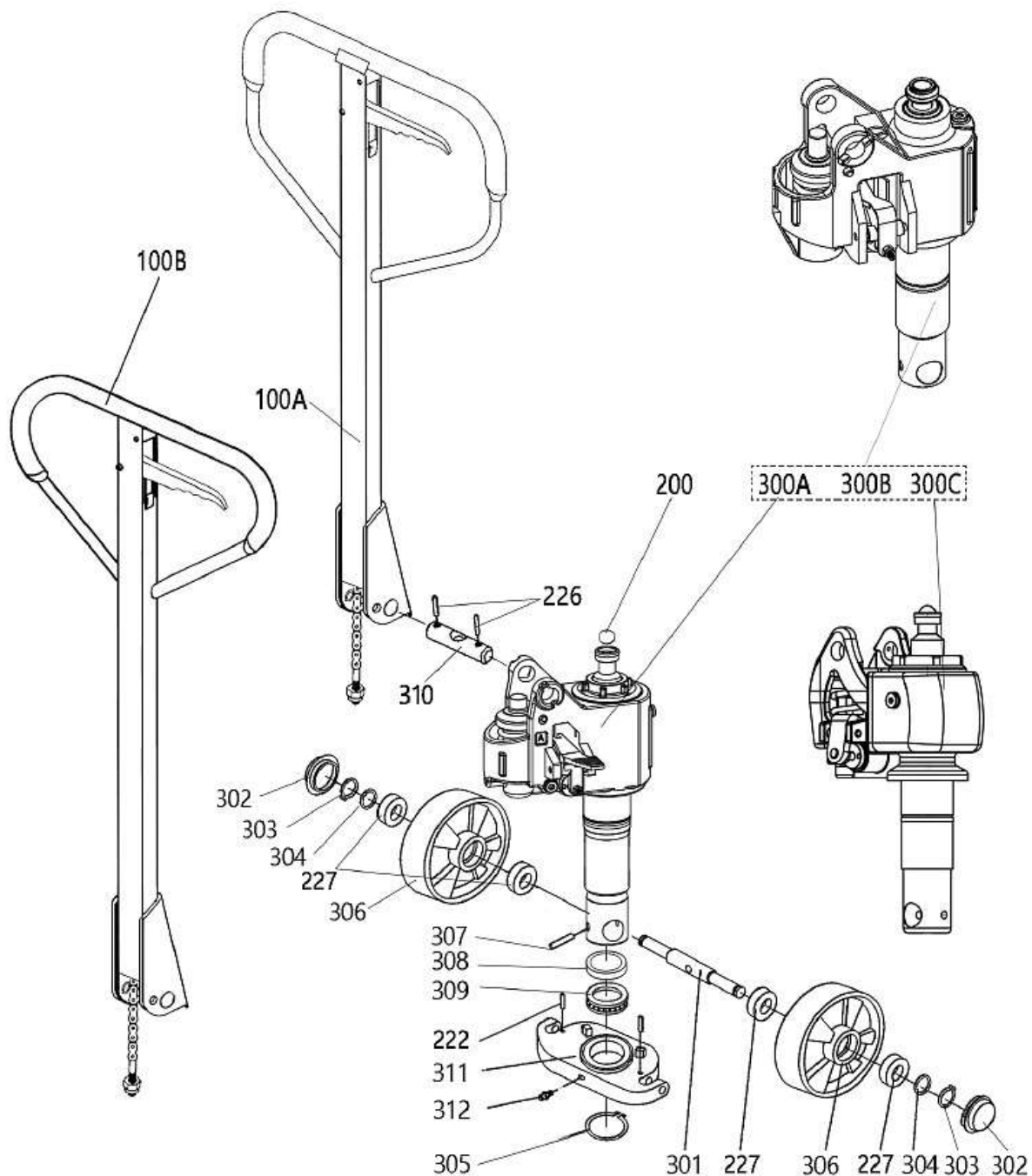
Abb.10-2: Ersatzteilzeichnung 2
