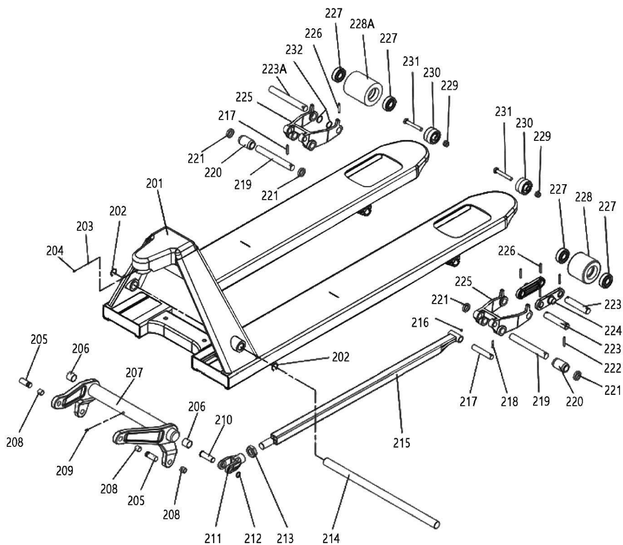
Abb.10-1: Ersatzteilzeichnung 1
