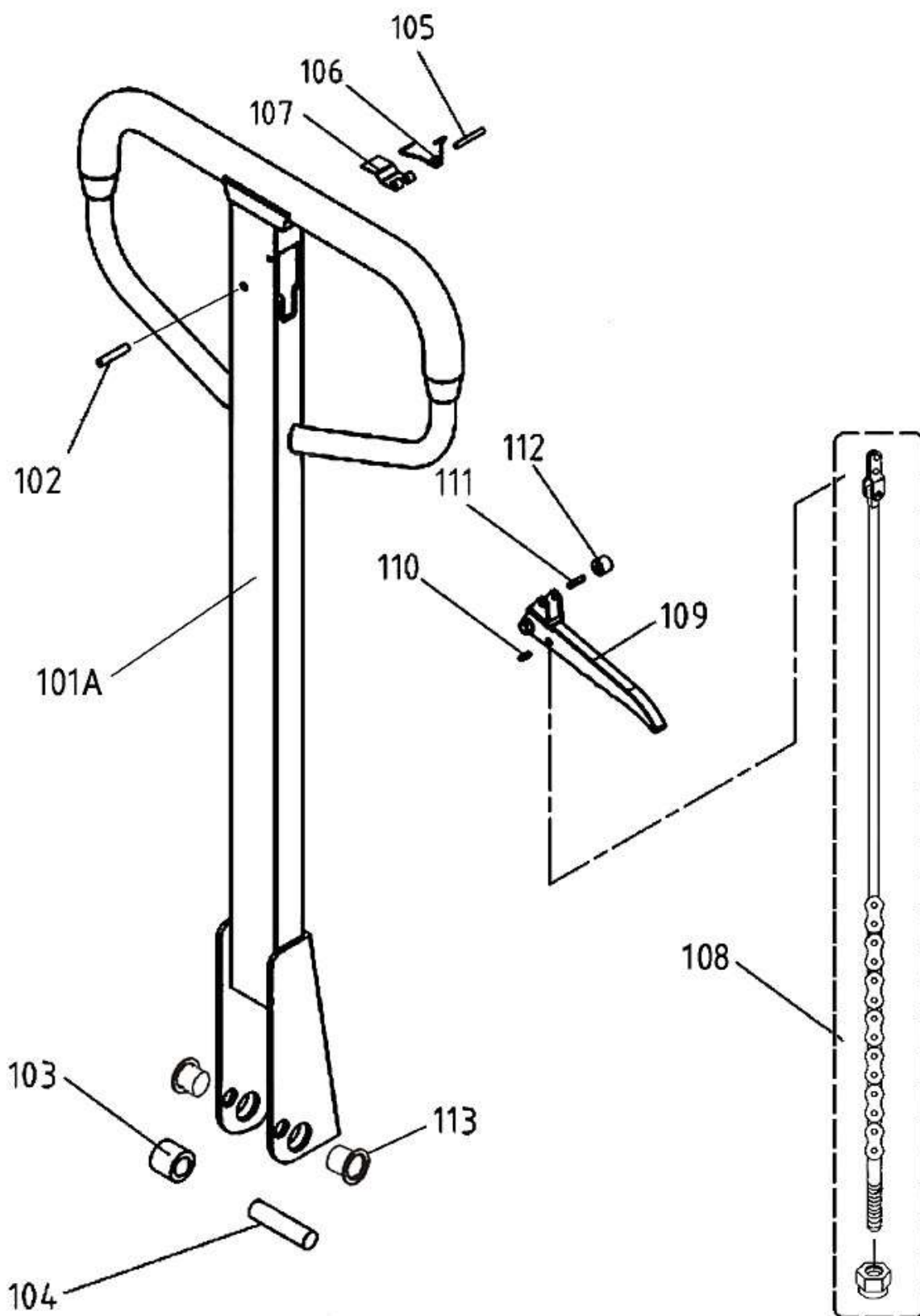
Abb.10-3: Ersatzteilzeichnung 3
