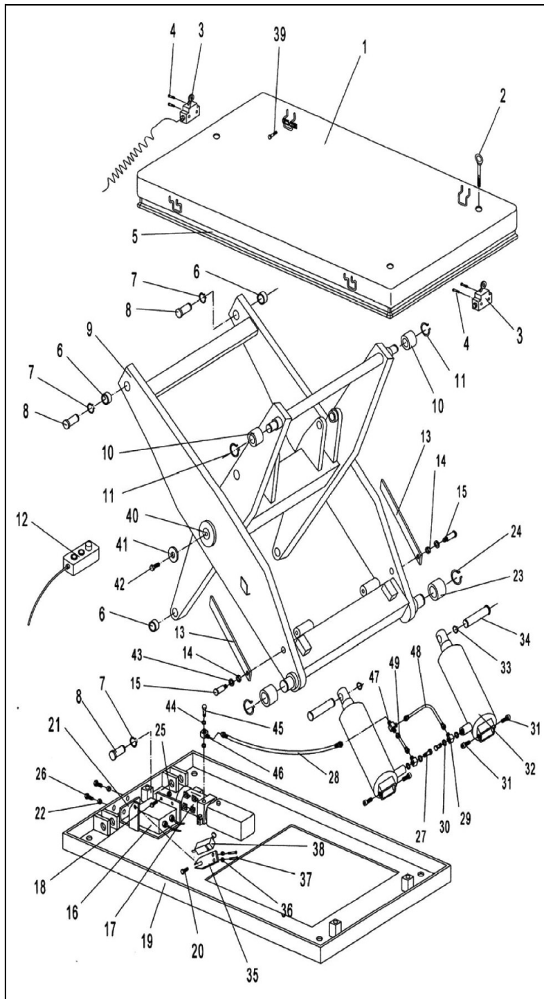
Abb. 2: Ersatzteilzeichnungen 1 &amp; 2 - SHT 2000 / Spare parts drawings 1 &amp; 2 - SHT 2000
