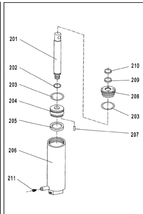
Ersatzteilzeichnung 3 / Spare parts drawing 3
