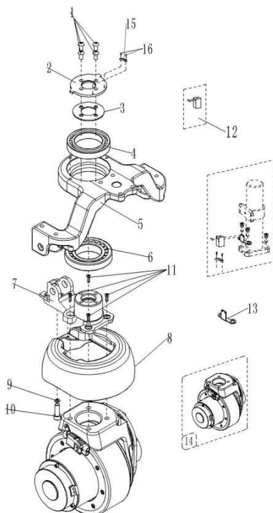
Abb. / Fig. 3: Ersatzteilzeichnung 3 EHW 12 / Spare parts drawing 3 EHW 12
