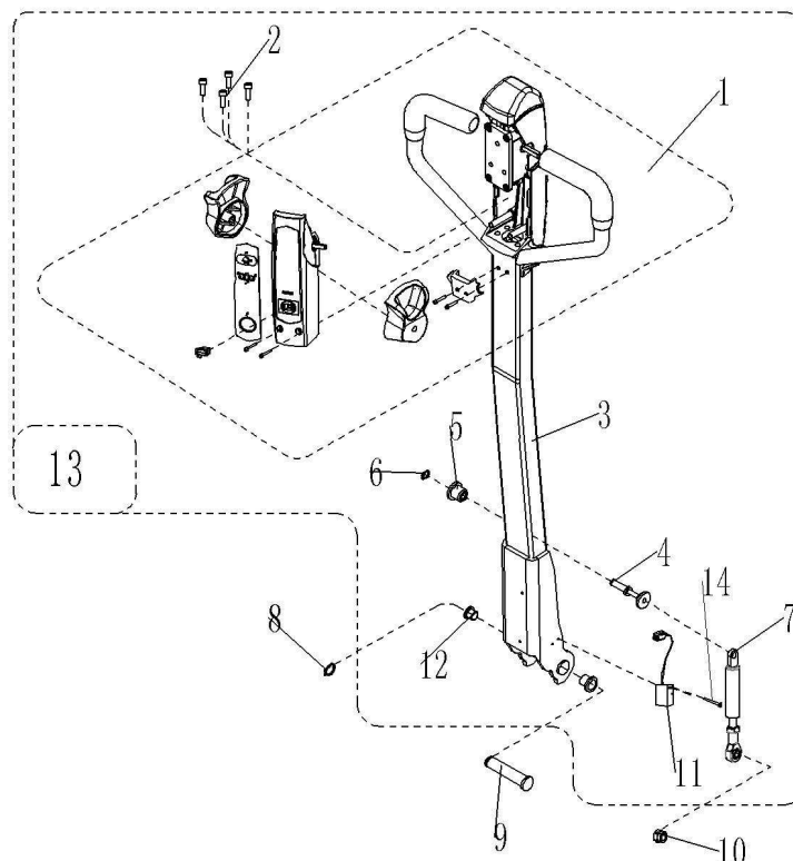
Abb. / Fig. 11: Ersatzteilzeichnung 11 EHW 12 / Spare parts drawing 11 EHW 12
