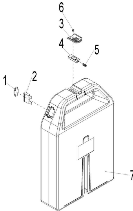
Abb. / Fig. 12: Ersatzteilzeichnung 12 EHW 12 / Spare parts drawing 12 EHW 12
