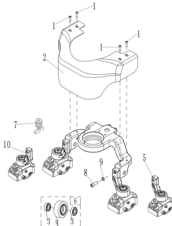
Abb. / Fig. 8: Ersatzteilzeichnung 8 EHW 12 / Spare parts drawing 8 EHW 12
