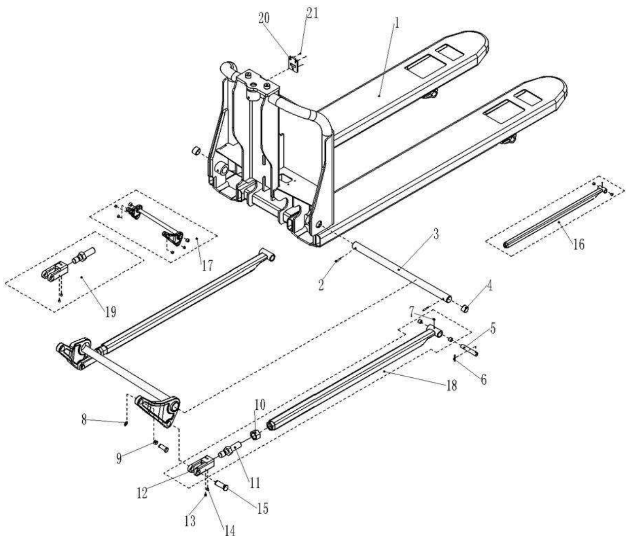
Abb. / Fig. 1: Ersatzteilzeichnung 1 EHW 12 / Spare parts drawing 1 EHW 12
