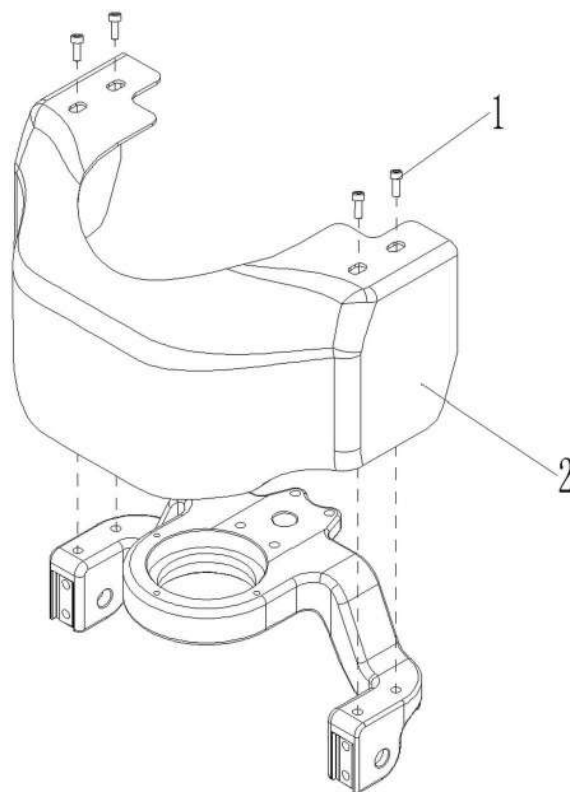
Abb. / Fig. 7: Ersatzteilzeichnung 7 EHW 12 / Spare parts drawing 7 EHW 12
