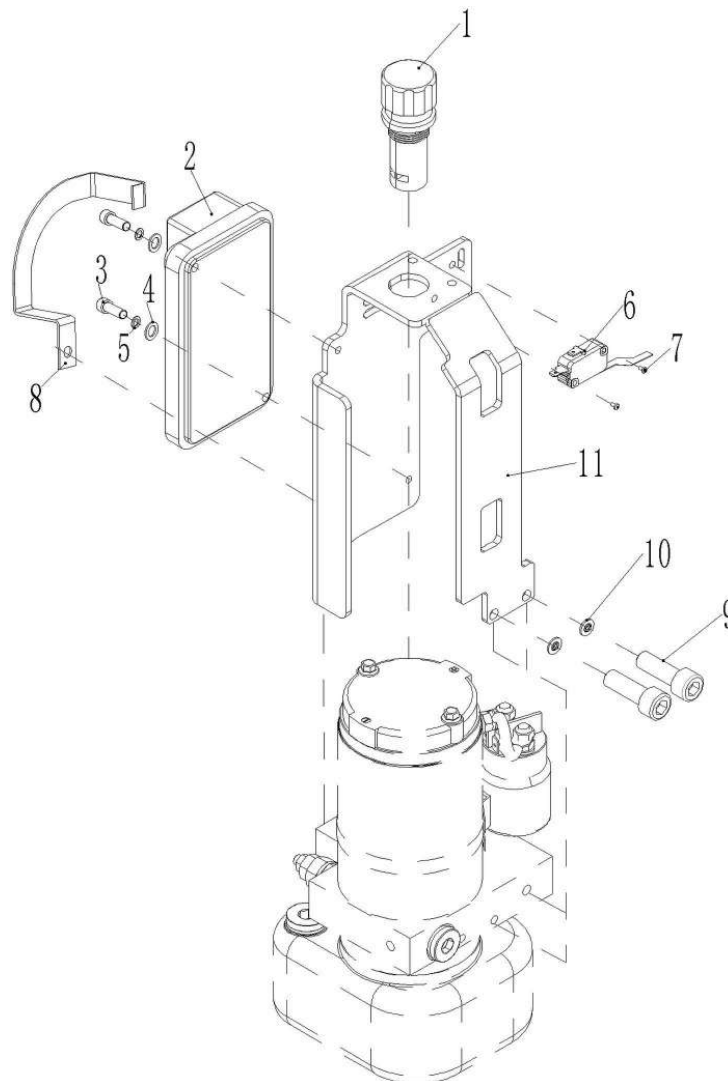
Abb. / Fig. 14: Ersatzteilzeichnung 14 EHW 12 / Spare parts drawing 14 EHW 12
