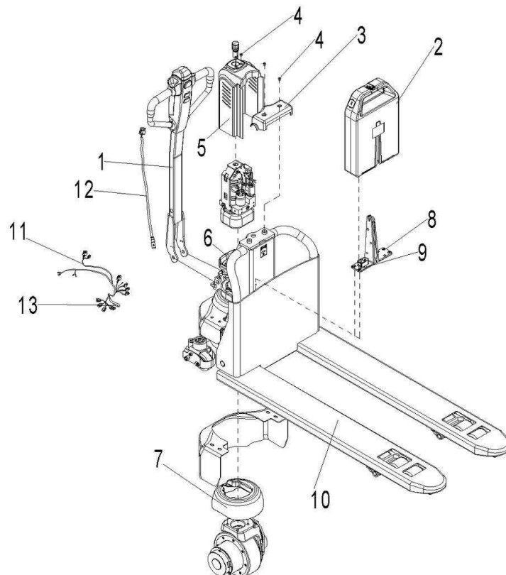
Abb. / Fig. 13: Ersatzteilzeichnung 13 EHW 12 / Spare parts drawing 13 EHW 12
