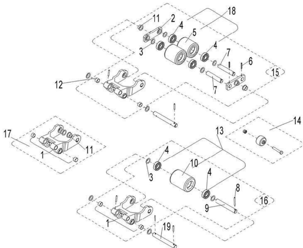
Abb. / Fig. 2: Ersatzteilzeichnung 2 EHW 12 / Spare parts drawing 2 EHW 12
