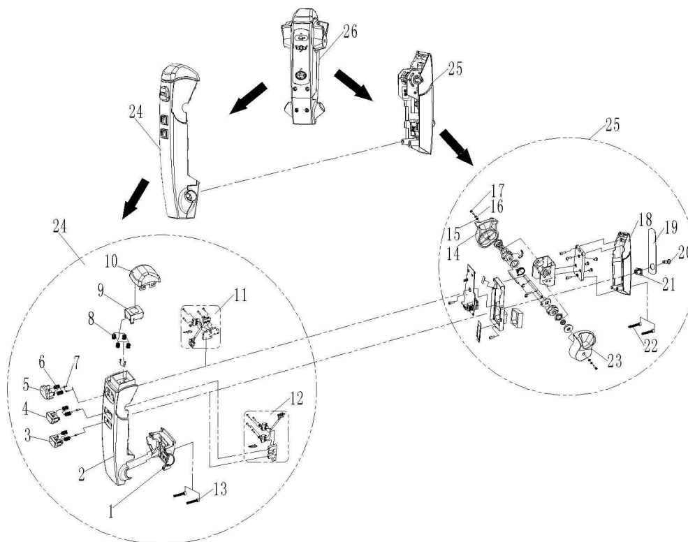
Abb. / Fig. 10: Ersatzteilzeichnung 10 EHW 12 / Spare parts drawing 10 EHW 12
