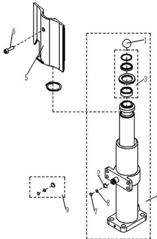
Abb. / Fig. 4: Ersatzteilzeichnung 4 EHW 12 / Spare parts drawing 4 EHW 12
