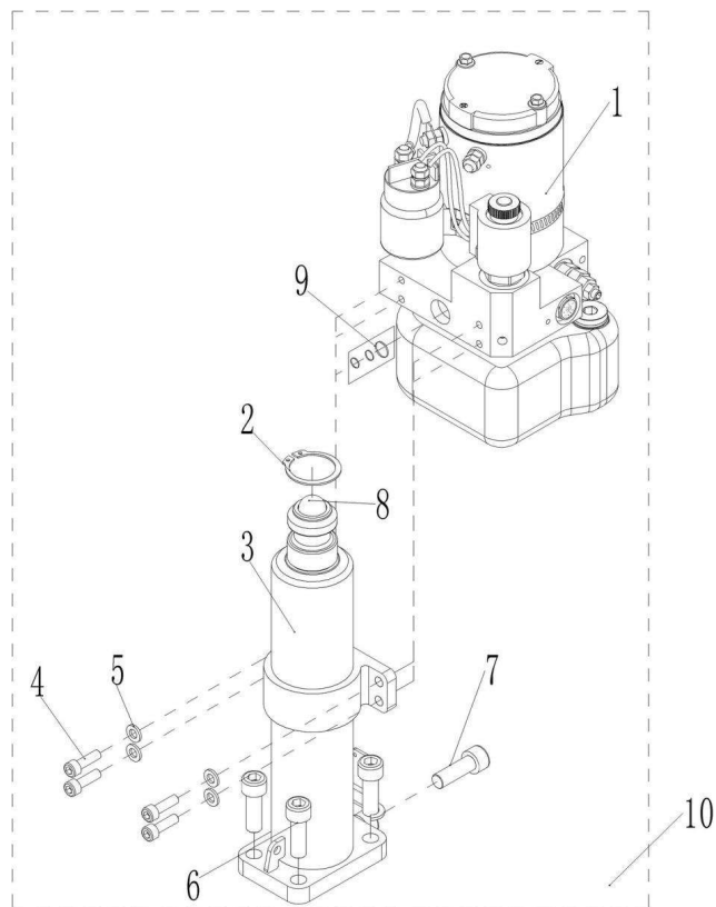
Abb. / Fig. 9: Ersatzteilzeichnung 9 EHW 12 / Spare parts drawing 9 EHW 12
