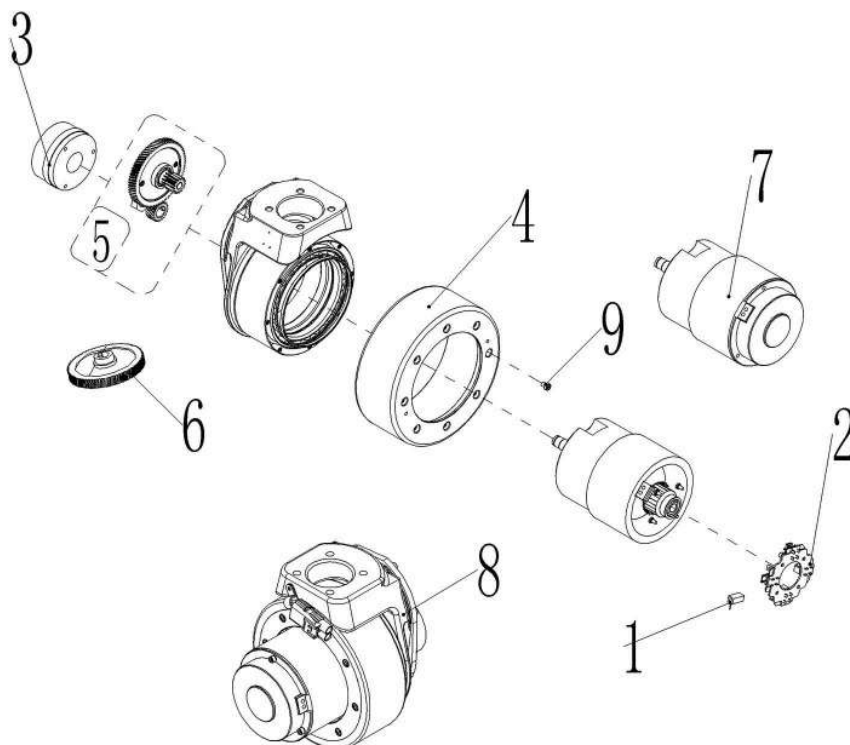
Abb. / Fig. 5: Ersatzteilzeichnung 5 EHW 12 / Spare parts drawing 5 EHW 12
