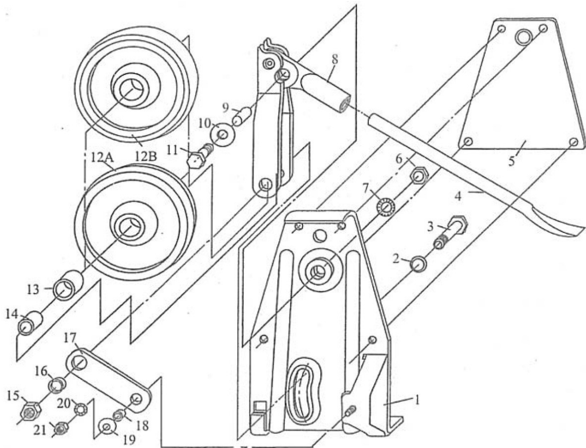
Abb. / Fig. 1: Ersatzteilzeichnung - HR 1000 / Spare parts drawing - HR 1000
