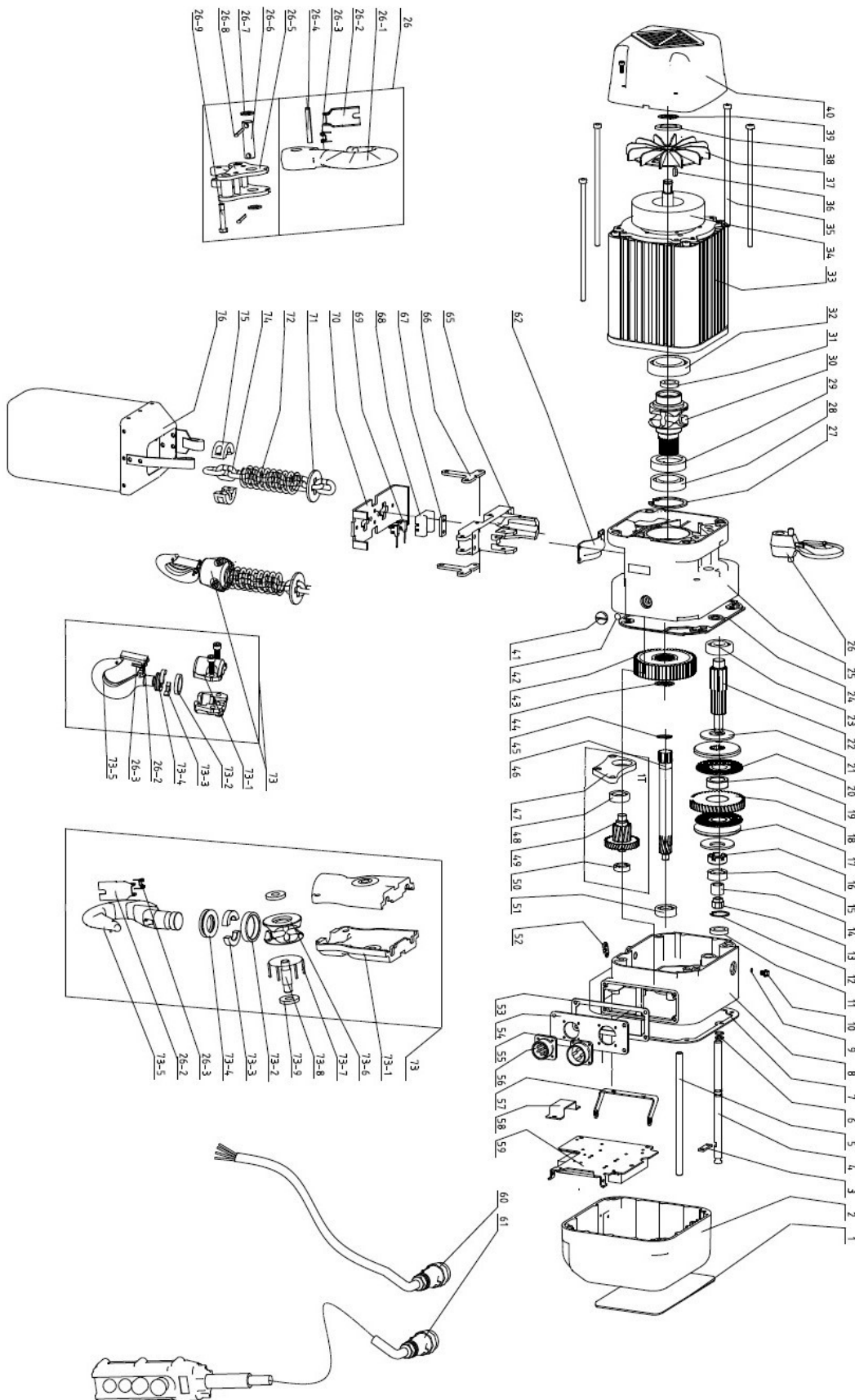
Abb. / Fig. 1: Ersatzteilzeichnung / Spare parts drawing - EKZT 5-1,5-2 & EKZT 10-1,10-2 & EKZT 20-1,20-2
