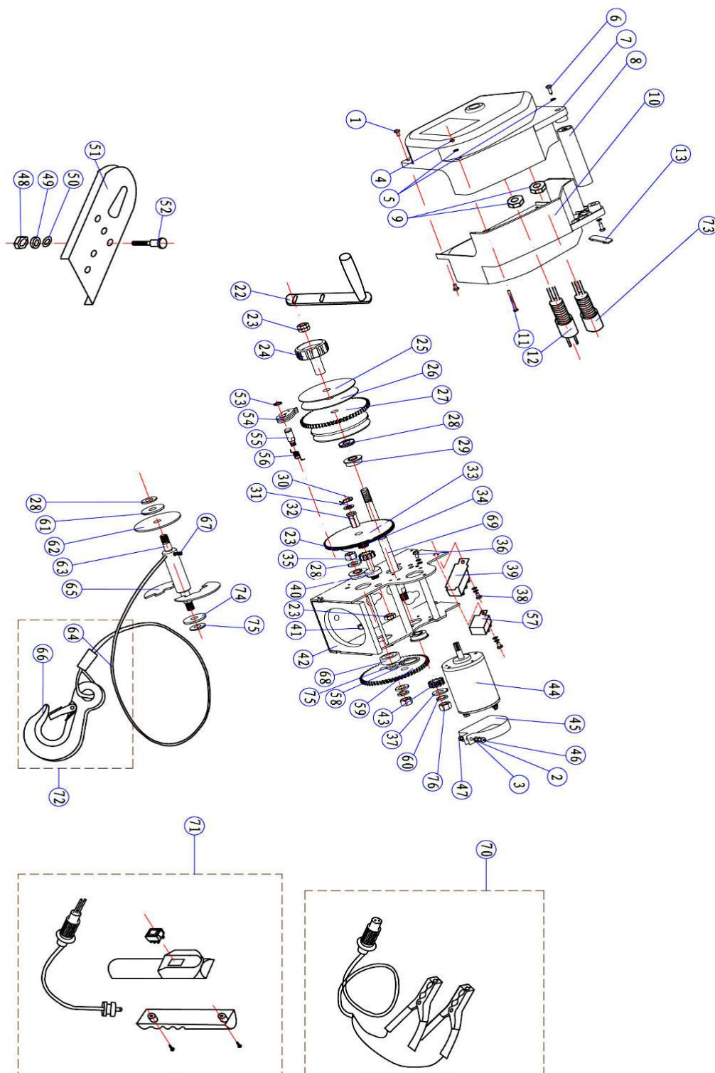
Abb. / Fig. 1: Ersatzteilzeichnung ESW 901 / Spare parts drawing ESW 901
