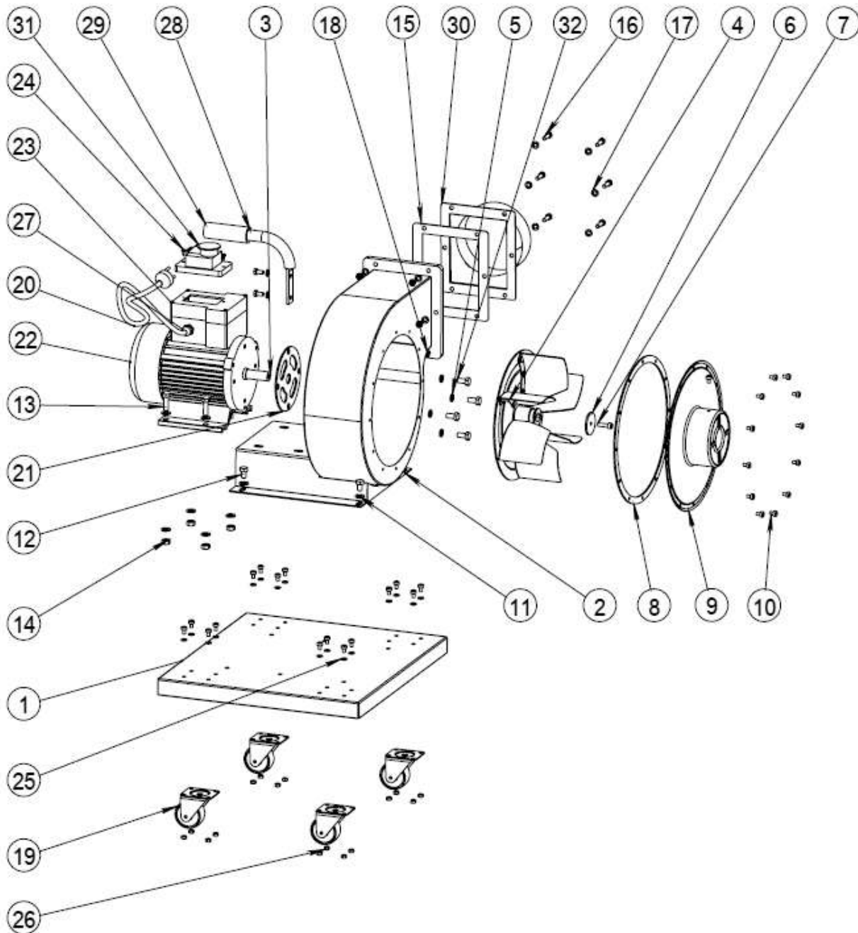
Abb./Fig. 1: Ersatzteilzeichnung RV 230 / Spare parts drawing RV 230
