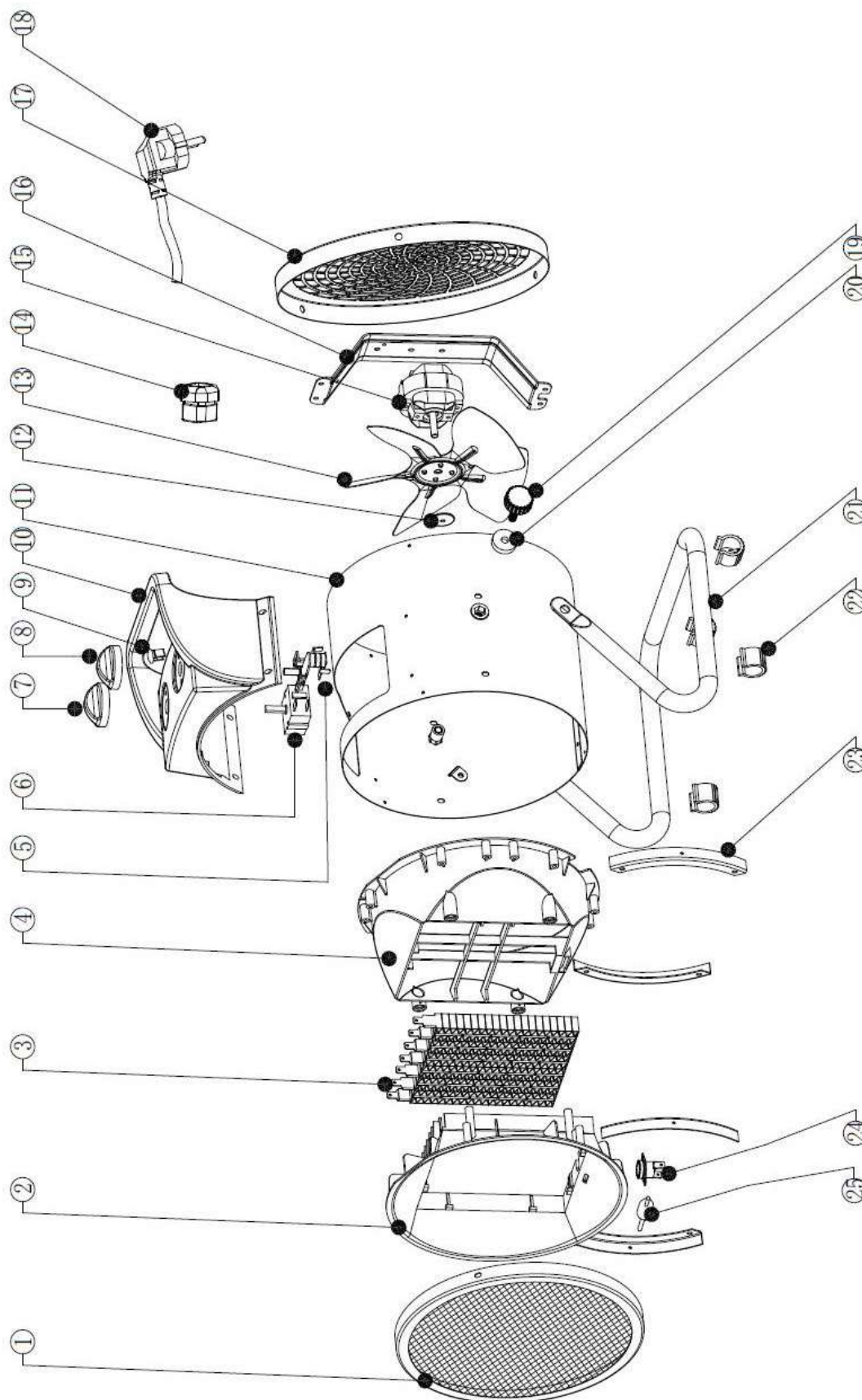
Abb.8-6: Ersatzteilzeichnung 6
