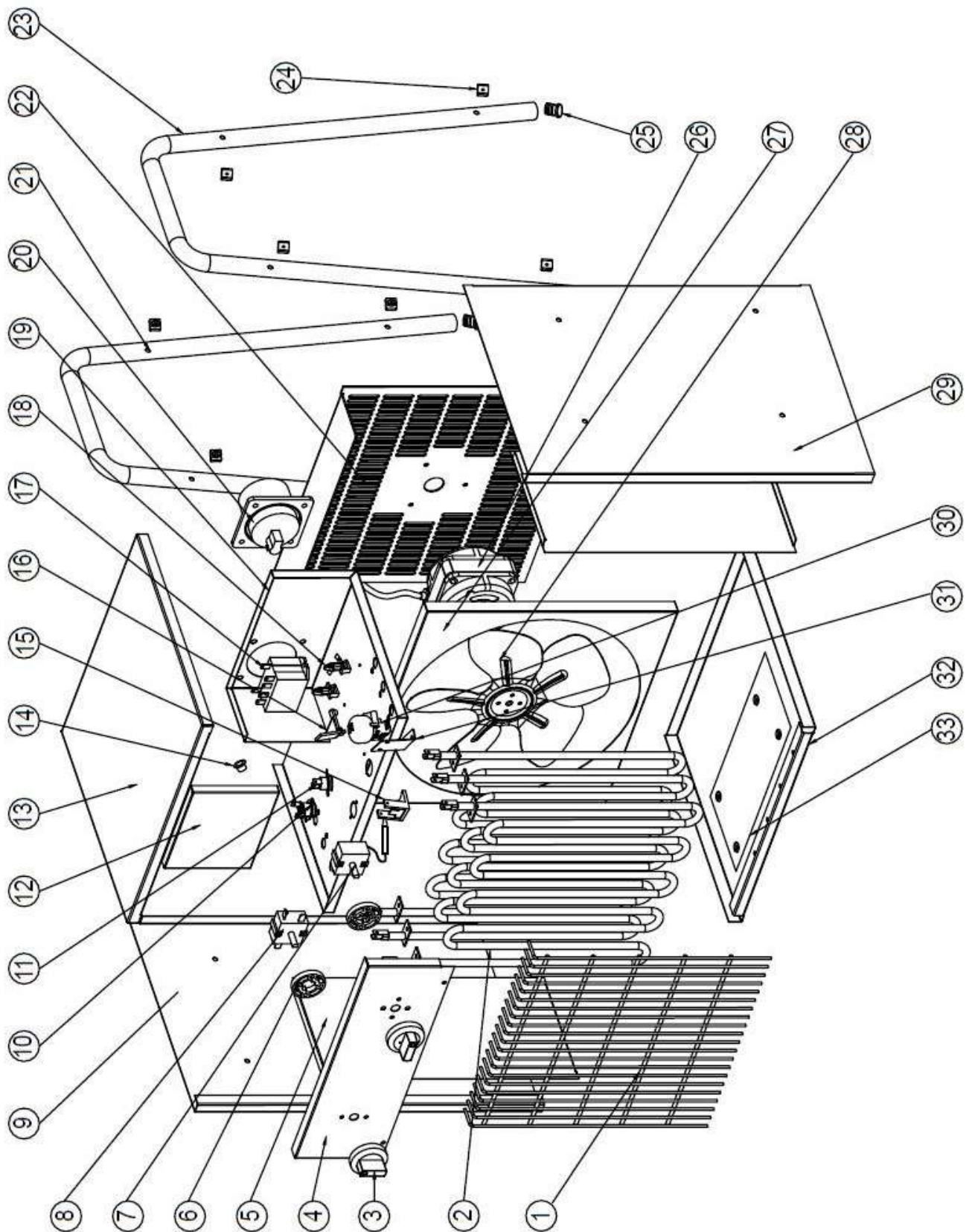
Abb.8-3: Ersatzteilzeichnung 3
